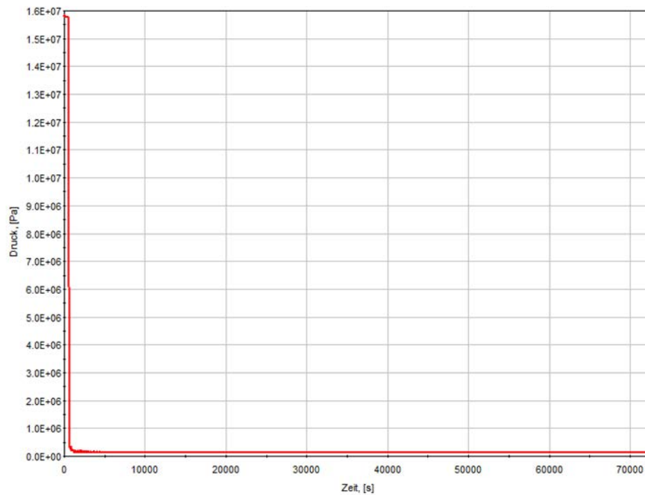
Abb. 4.18 2F-Bruch im kalten Strang: Verlauf des Primärkreisdrucks
