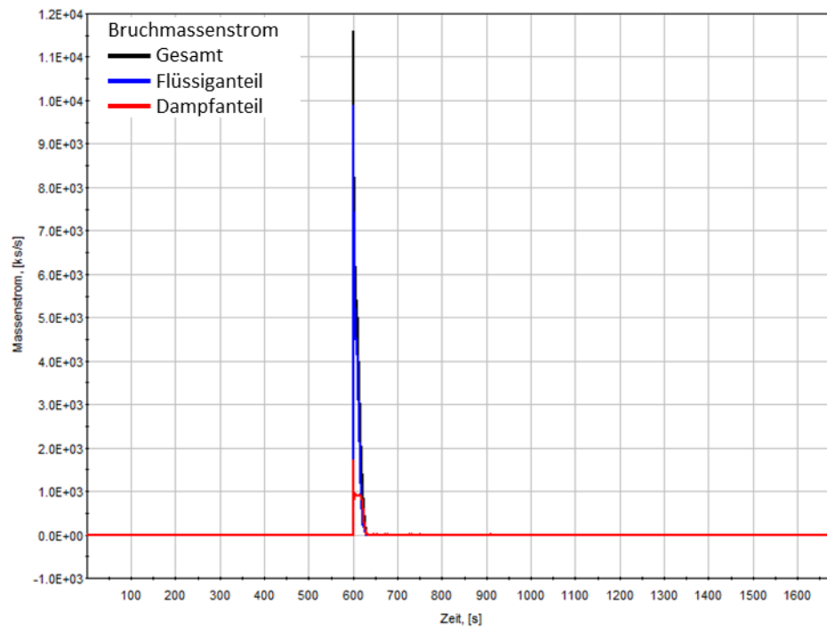
Abb. 4.10 2F-Bruch im heißen Strang: Bruchmassenstrom (schwarz: Gesamtmassenstrom, blau: Flüssiganteil, rot: Dampfanteil) auf der Dampferzeuger-Seite
