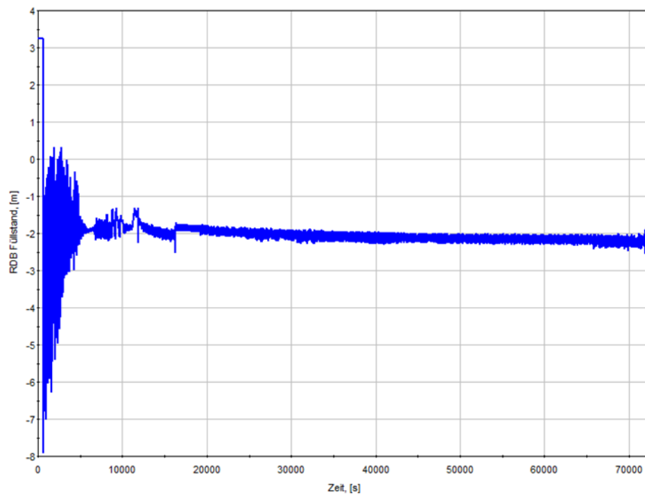
Abb. 4.19 2F-Bruch im kalten Strang: RDB-Füllstand
