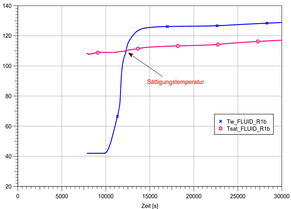
Abb. 2.108 COCOSYS, Wassertemperatur in der Spalte hinter der Seitenplatte (Zone R1b)
