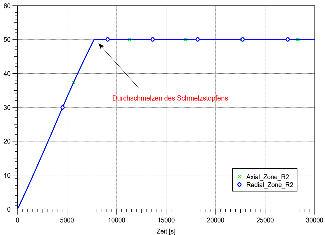
Abb. 2.103 COCOSYS, radiale und axiale Erosionstiefe in der Reaktorgrube (Zone R2)
