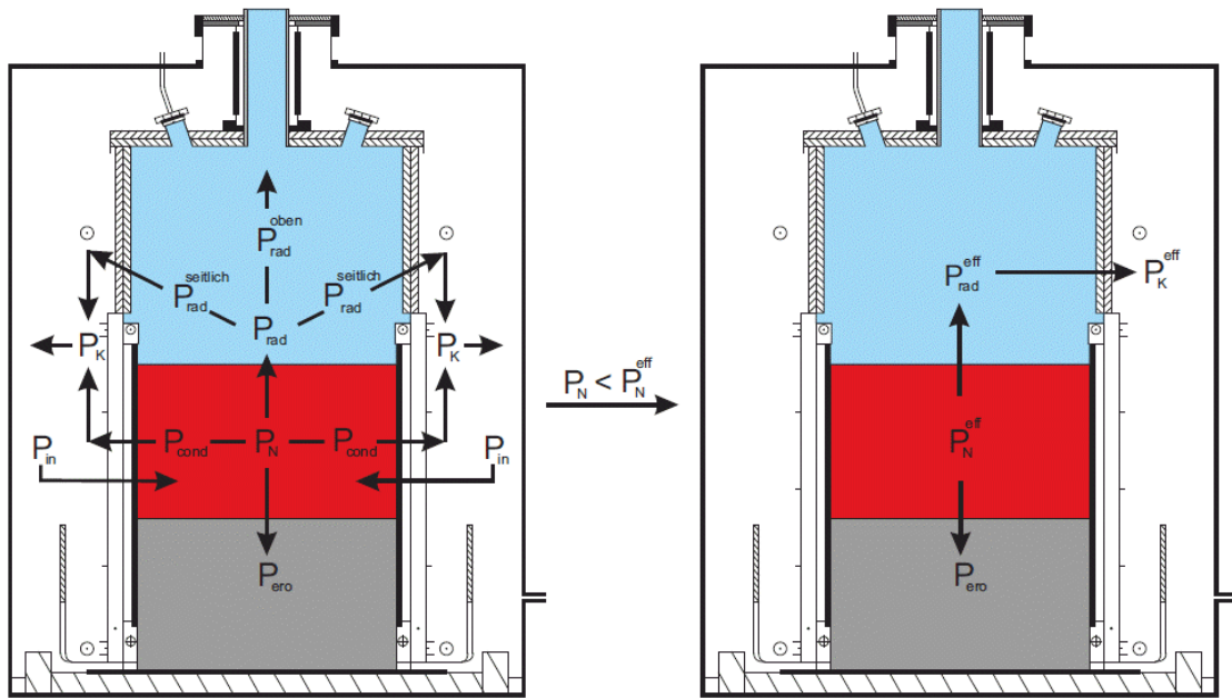
Abb. 2.77 Aufteilung der eingespeisten Leistung in den ACE-Versuchen /AGE 17/
