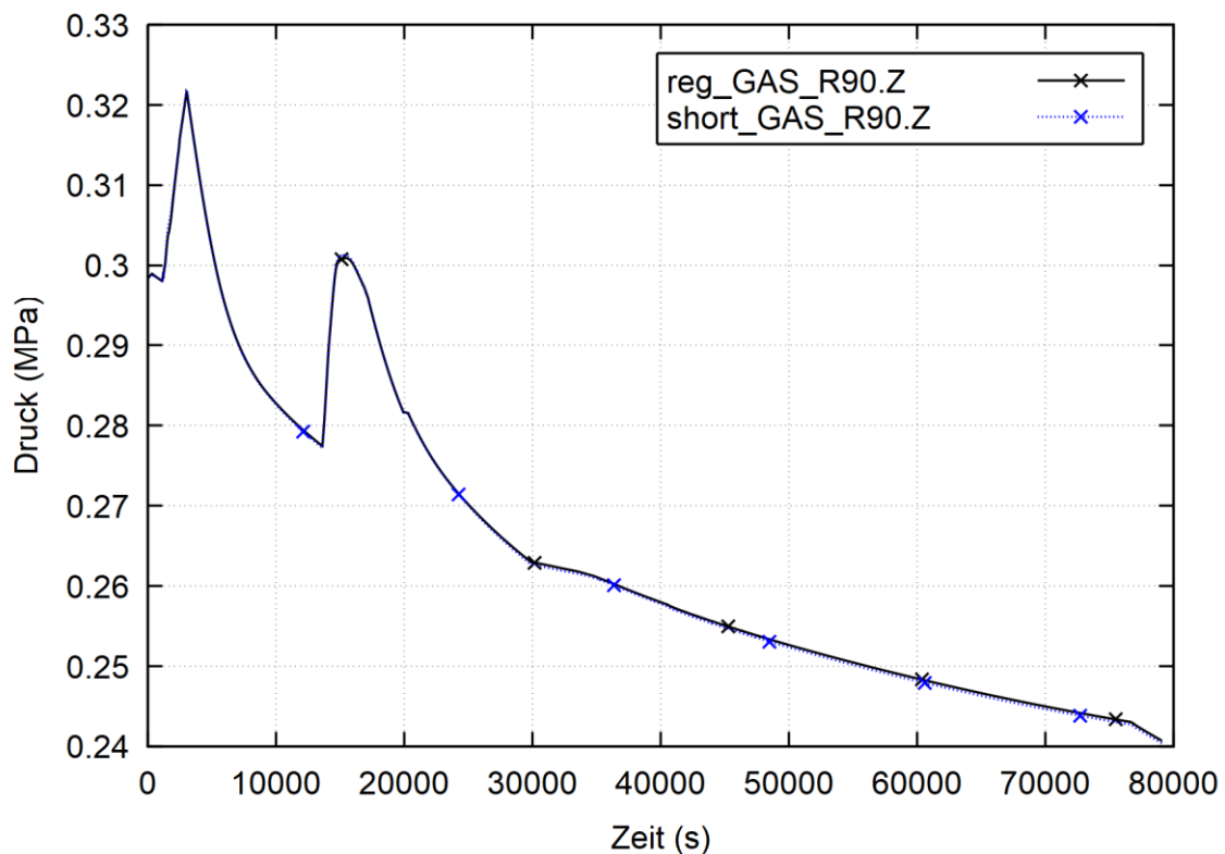
Abb. 4.12 Druck im PAR-Versuch (TTV)
