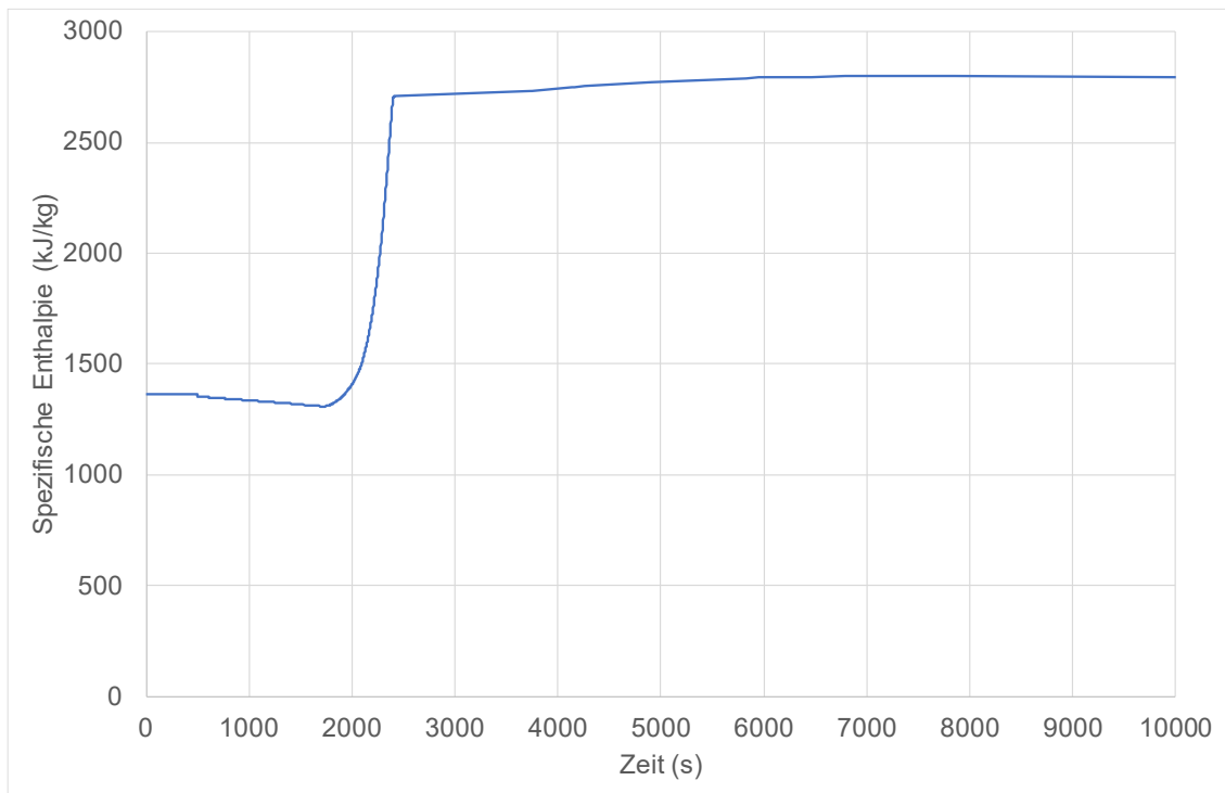
Abb. 3.56 Leckstörfall: Spezifische Enthalpie für die Einspeisung in COCOSYS-Zone C1
