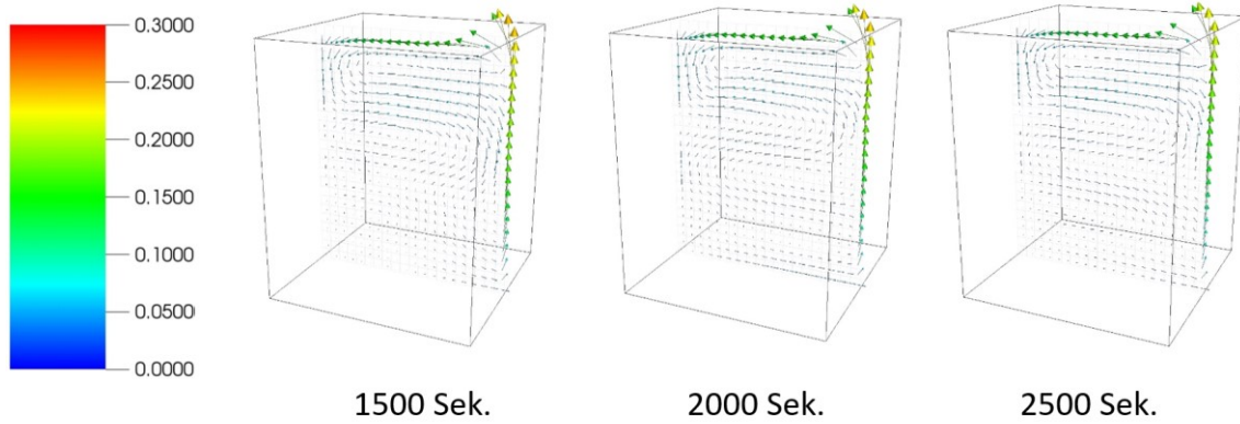
Abb. 3.10 Geschwindigkeitsfeld (in m/s) für y = 10 m bei T = 1500 Sek., T = 2000 Sek. und T = 2500 Sek.
