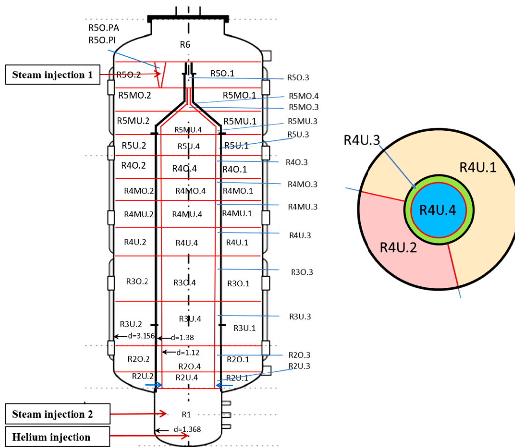
Abb. 2.4 THAI TH-29, COCOSYS Nodalisierung (vertikaler und horizontaler Schnitt)
