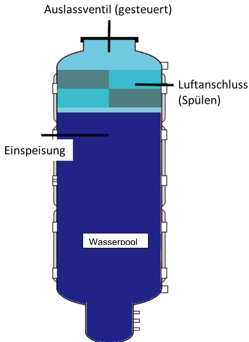
Abb. 2.47 THAI WH-33, COCOSYS-Nodalisierung
