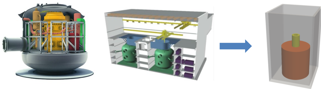
Abb. 3.24 Erstellung einer an den NUWARD™ SMR angelehnten Geometrie für Co-Pool
