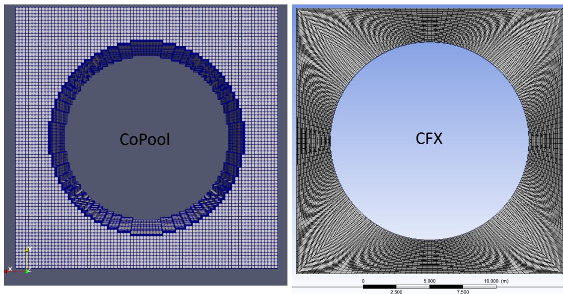
Abb. 3.34 Vergleich der Berechnungsgitter von CoPool und CFX
