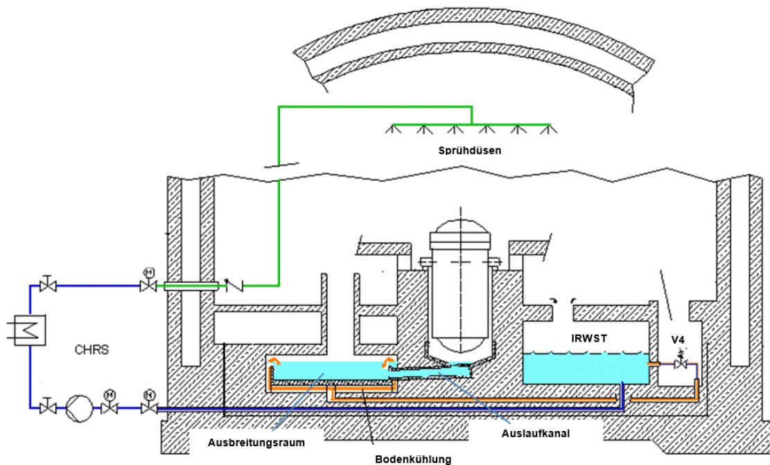
Abb. 2.99 EPR™ Kernfänger, passive Schmelzekühlung durch Wasserüberflutung der Kernschmelze, Areva NP (CC0), via Wikimedia Commons
