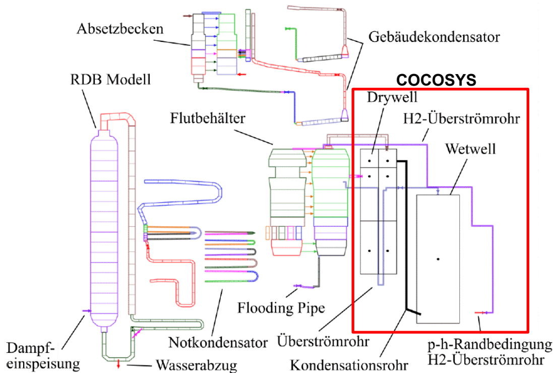
Abb. 3.96 ATHLET/COCOSYS-Nodalisierung der INKA-Versuchsanlage.
