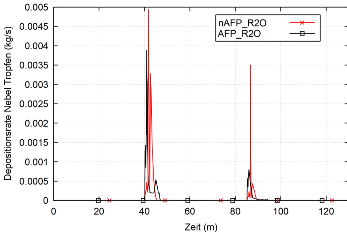
Abb. 2.51 THAI AW-4, Sedimentierungsrate von Nebeltropfen bei AFP und NewAFP
