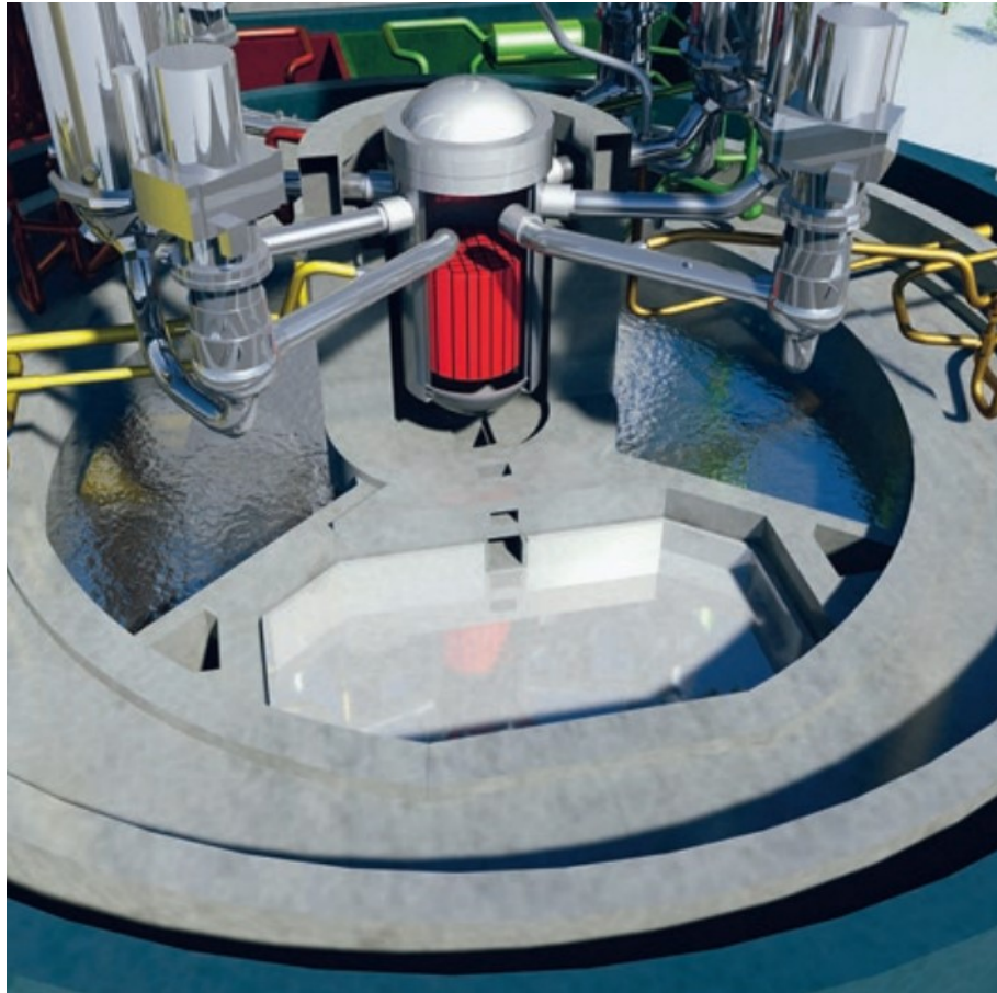
Abb. 2.97 Kernfänger des EPR™-Designs (Blick auf den Ausbreitungsraum) /AHN 15/
