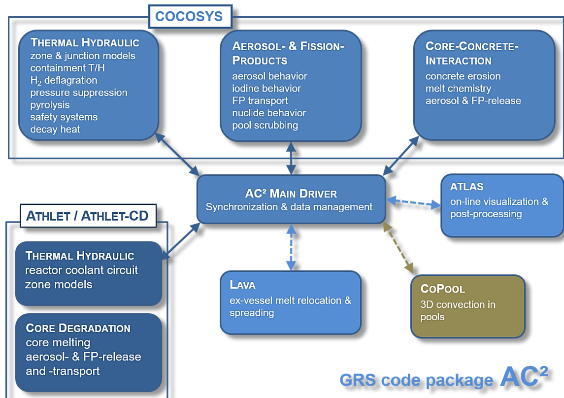
Abb. 1.1 Struktur des Programmsystems AC²
