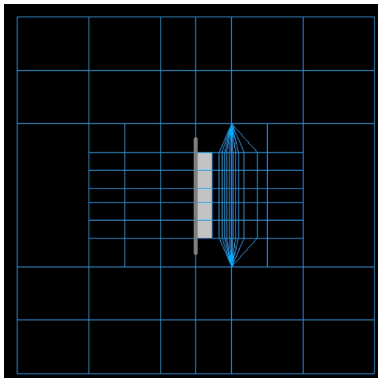
Abb. 2.115 Aufbau der SATURNE-Anlage. Die eingezeichnete Ebene bei 8 m ist die obere Grenze der COCOSYS-Nodalisierung /ZAV 13/
