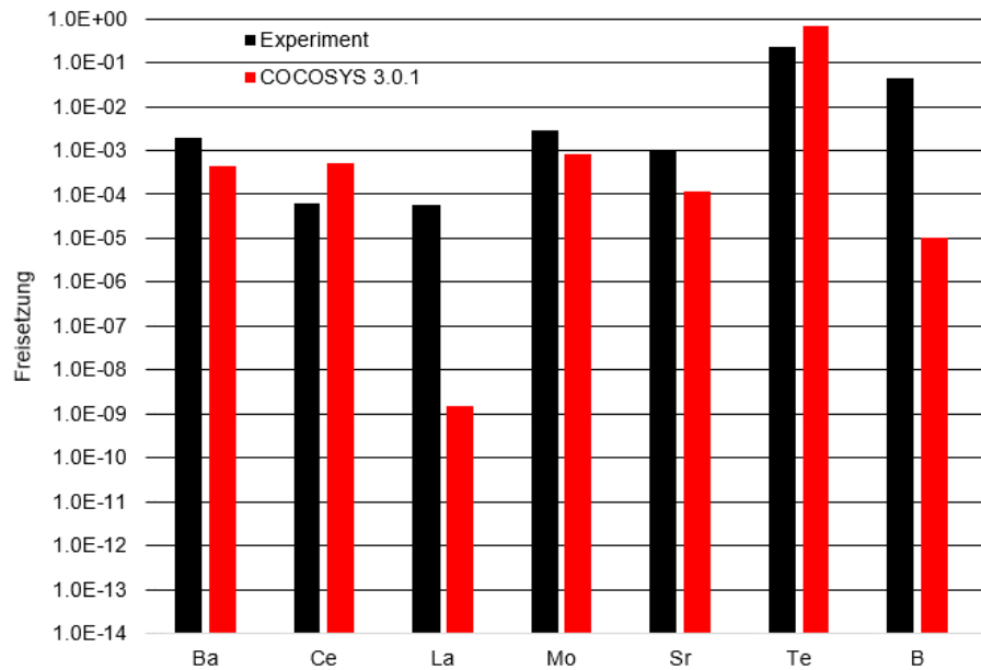
Abb. 2.89 ACE L7, Vergleich der berechneten Anteile der aus der Schmelze freigesetzten Spaltprodukte mit den im Experiment ermittelten Anteilen der freigesetzten Spaltprodukte (bezogen auf das Anfangsinventar)
