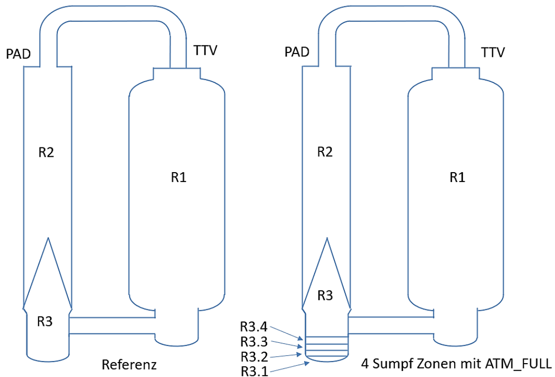
Abb. 2.18 COCOSYS-Nodalisierungen – Referenznodalisierung (links) und Nodalisierung mit vollständig mit Wasser gefüllten Zonen (R3.1 – R3.4) und ATM_FULL-Verbindungen (rechts)
