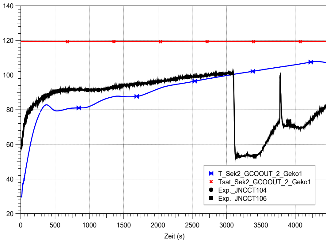
Abb. 3.95 CCC_050_030_20_1, Vergleich der berechneten Austrittstemperaturen (Sektion 2) am Rücklaufrohr mit den im Experiment gemessenen Temperaturen in der Rücklaufleitung (auf Höhe 22,8 m)
