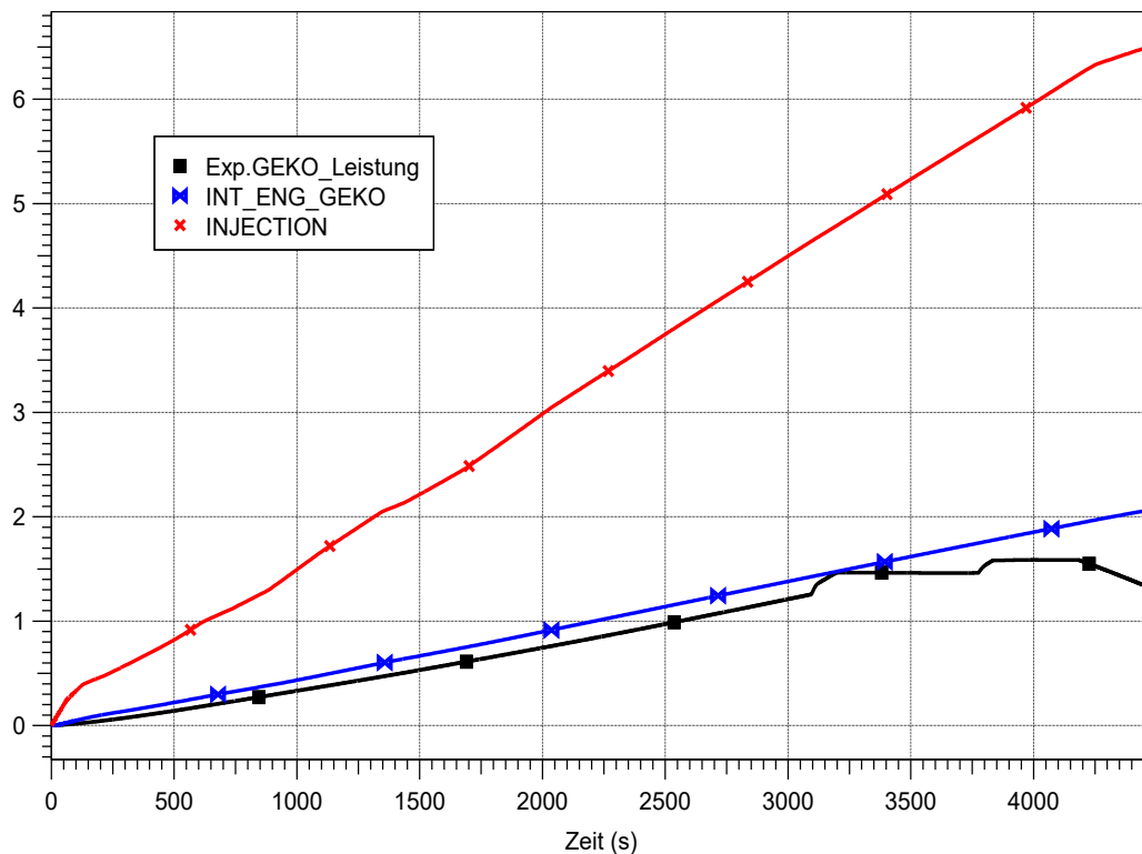
Abb. 3.93 CCC_050_030_20_1, Vergleich des Integrals der vom GEKO berechneten Kühlleistung mit dem Integral der im Experiment ermittelten Kühlleistung des Gebäudekondensators und der in den Flutbehälter eingespeisten Dampfernergie
