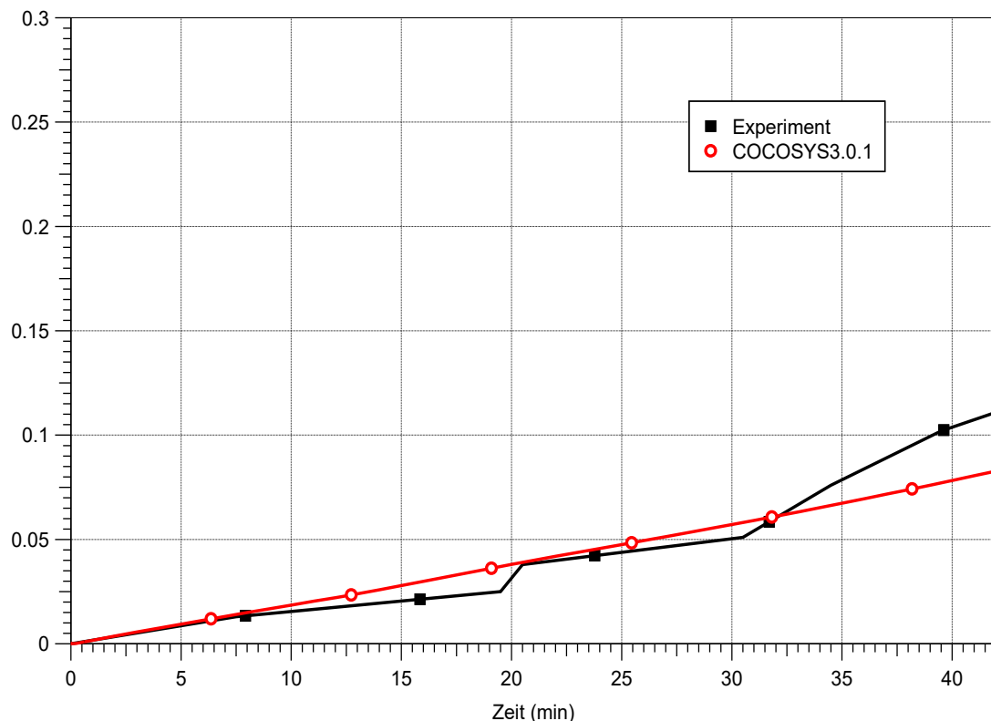
Abb. 2.82 ACE L6, Vergleich der berechneten Betonerosionstiefe in axialer Richtung mit dem im Experiment durch Thermoelemente ermittelten Erosionsfortschritt
