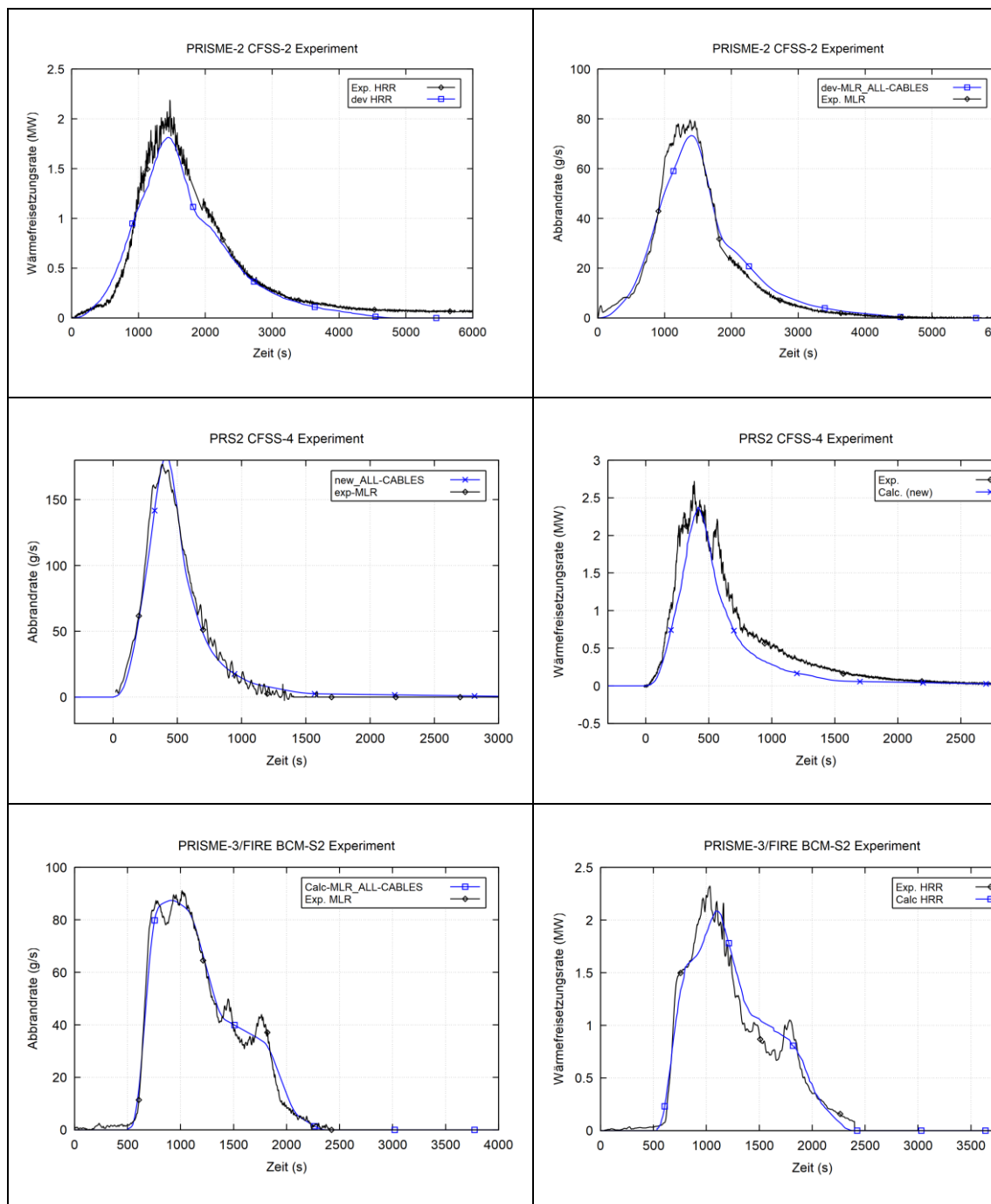
Abb. 2.118 Vergleich der gemessenen und berechneten MLR (links) und HRR (rechts) für den PRS2-CFSS-2, -4 und PRF-BCM-S2 Test
