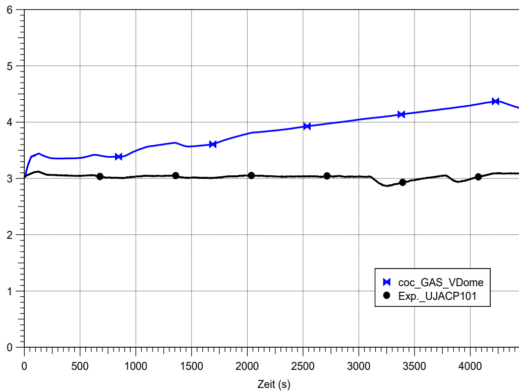
Abb. 3.89 CCC_050_030_20_1, Vergleich des berechneten Druckes mit dem im Experiment gemessenen Druckverlauf im Dom des Flutbehälters
