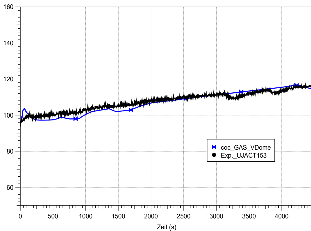
Abb. 3.90 CCC_050_030_20_1, Vergleich der berechneten mit der im Experiment gemessenen Atmosphärentemperatur im Flutbehälter
