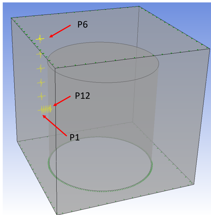
Abb. 3.25 Position der Monitorpunkte im Wasserpool
