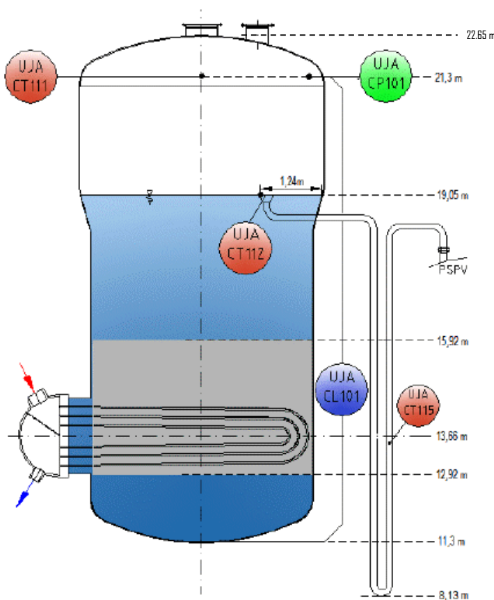
Abb. 3.72 Flutbehälter mit Messstellen für den Druck und die Temperatur /WAG 17/
