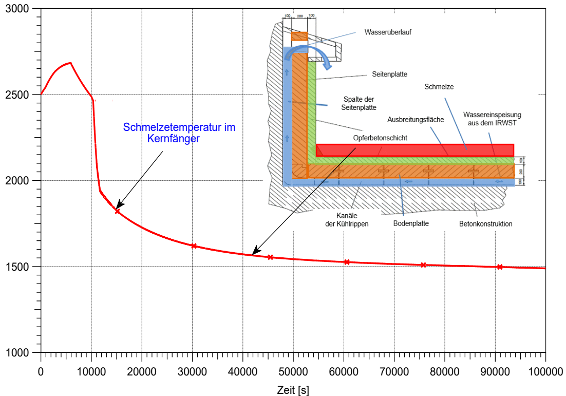
Abb. 2.105 COCOSYS, zeitlicher Verlauf der Schmelzetemperatur im Kernfänger
