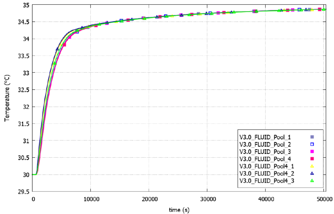
Abb. 3.62 Frühere Rechnung /BEC 18/: Temperaturverlauf im Wasserpool
