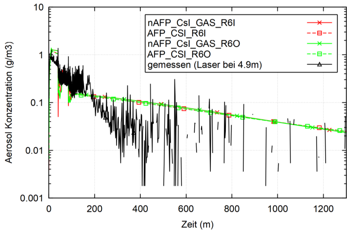
Abb. 2.55 THAI AW-4, Unterschied der Aerosolkonzentrationen auf 4,9 m Höhe (andere Tropfengröße)
