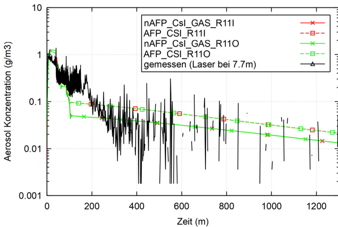
Abb. 2.53 THAI AW-4, Unterschied der Aerosolkonzentrationen auf 7,7 m Höhe
