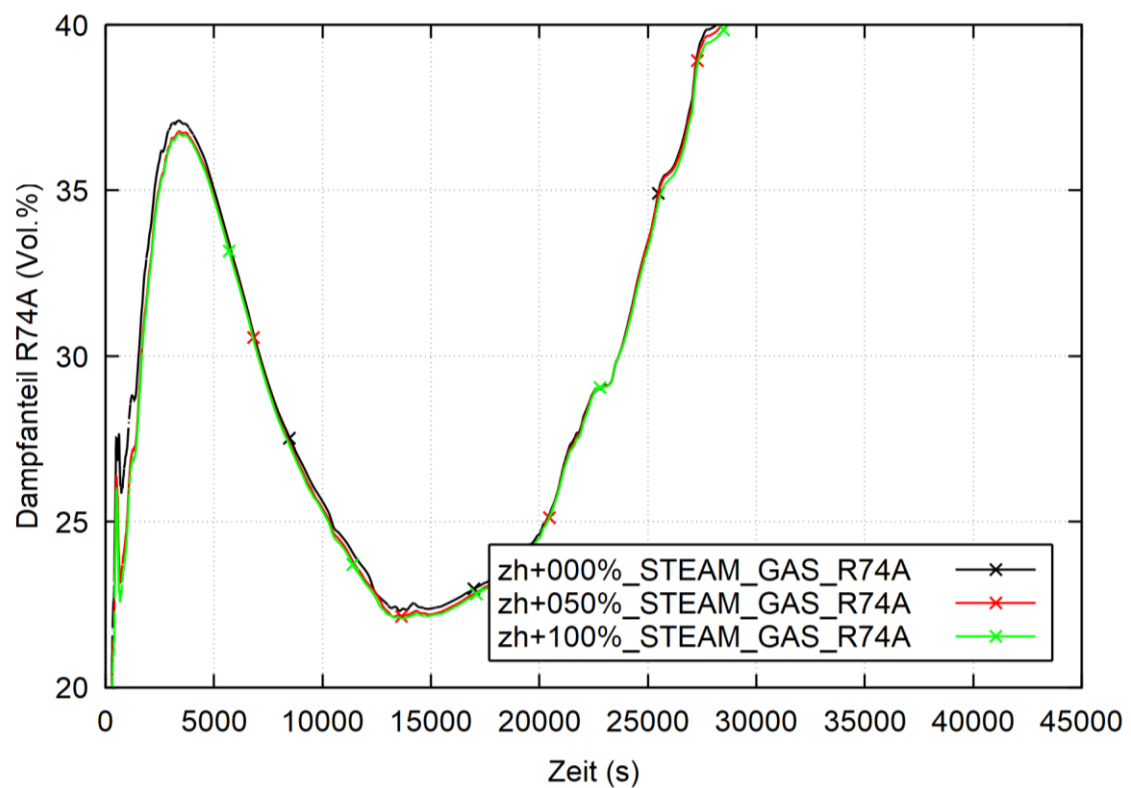
Abb. 4.6 DWR-KONVOI, COCOSYS-Rechnung: Dampfanteil in der äußeren Peripherie unterhalb Beckenflur (MBL-Fall)
