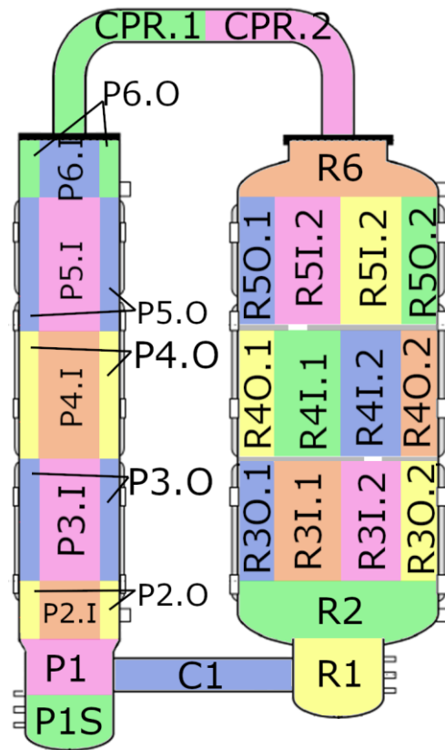
Abb. 2.42 THAI Iod-33, THAI + -Konfiguration (PAD links, TTV rechts) mit COCOSYS-Nodalisierung und Kennzeichnung der Zonen
