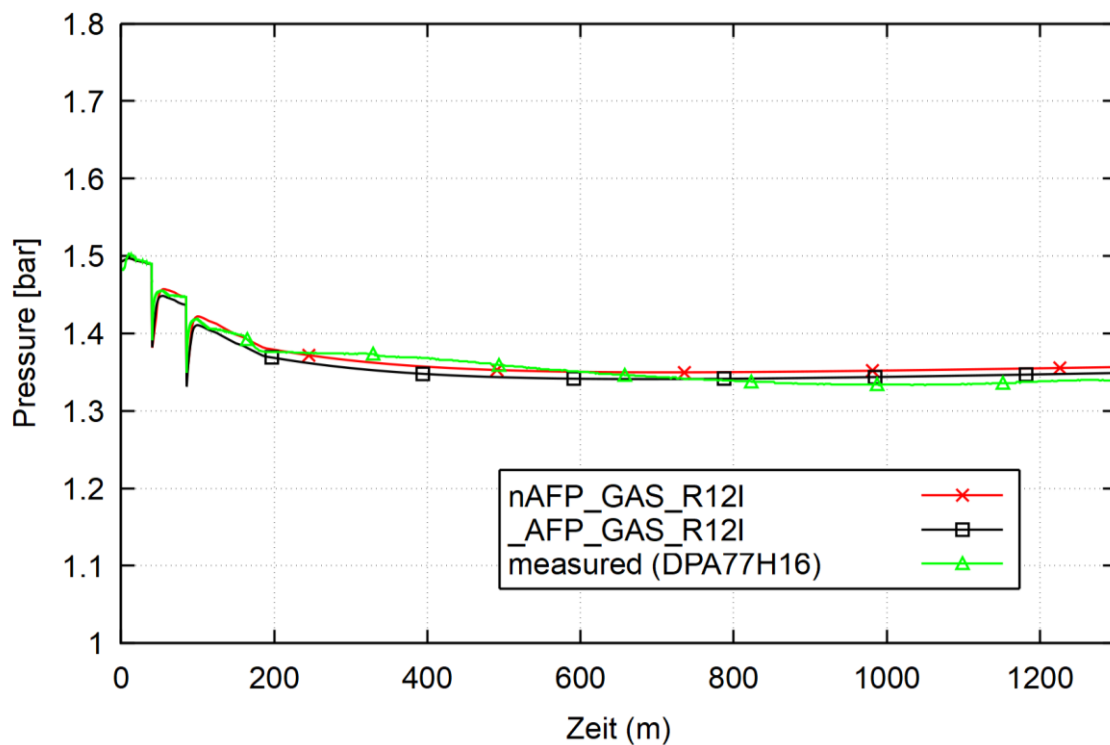
Abb. 2.54 THAI AW-4, Druckverläufe bei Variation der Tropfengröße
