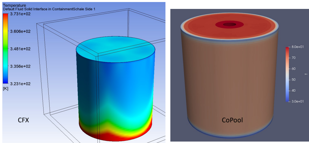
Abb. 3.39 Temperaturen an der Containment-Außenseite bei t = 1.000 s (Farbskala links in K, rechts in °C)
