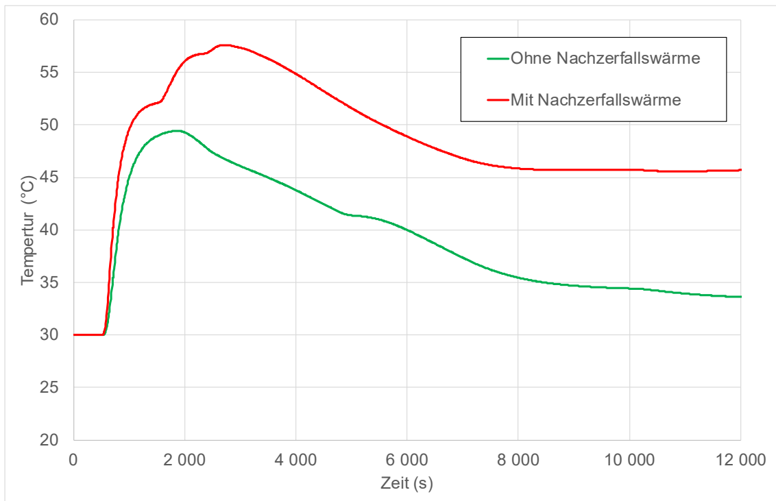
Abb. 3.67 Parameterstudie: Temperatur an der Containment-Wand (Pool-Seite)
