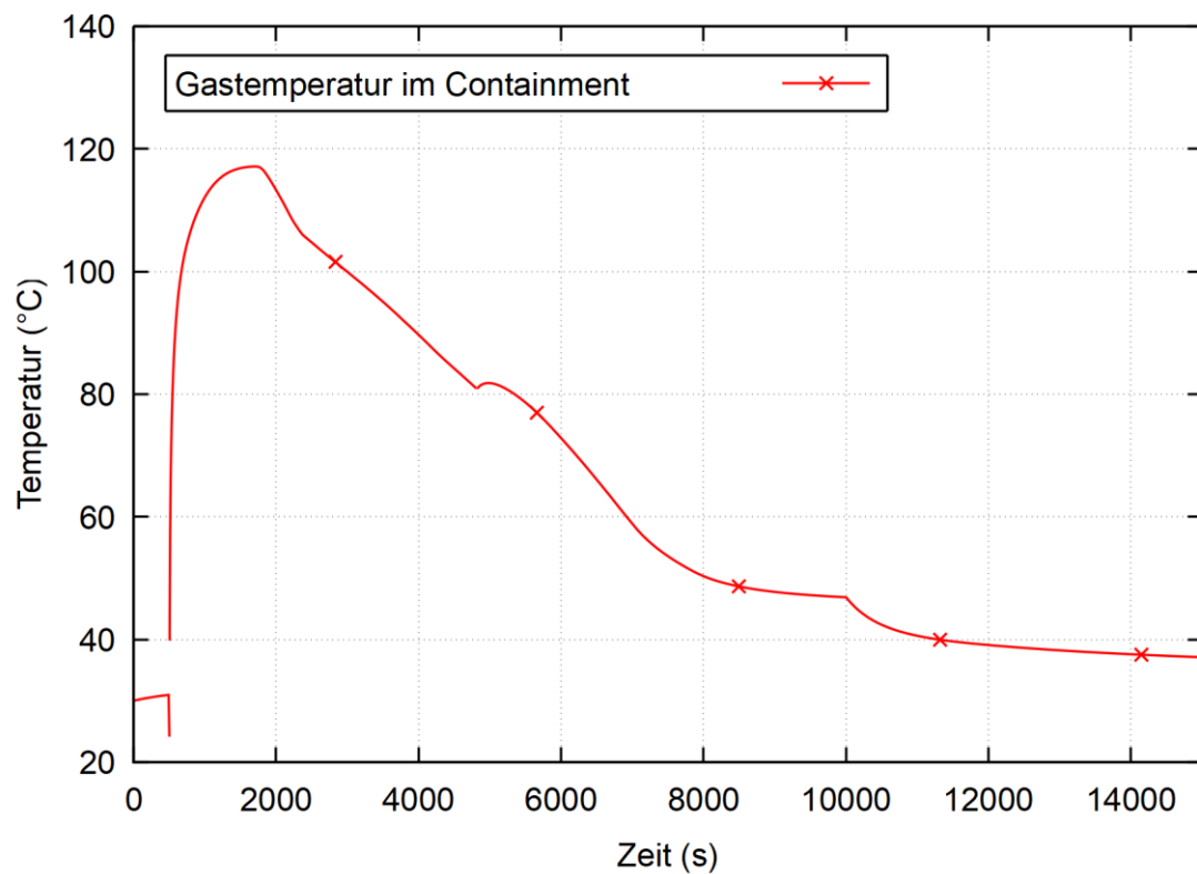
Abb. 3.59 Aktuelle Rechnung: Temperaturverlauf im Containment (COCOSYS-Zone C1)
