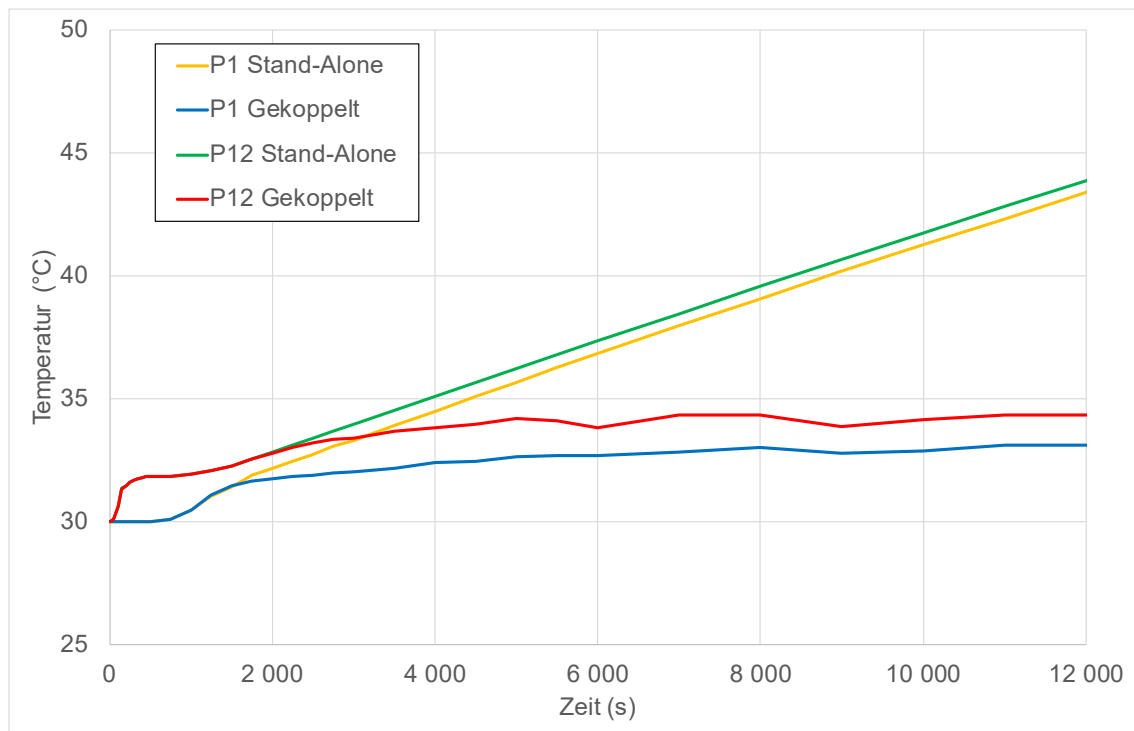
Abb. 3.49 Vergleich der Temperaturen an den Monitorpunkten P1 und P12 für die Stand-alone- und die gekoppelte CoPool/COCOSYS-Rechnung
