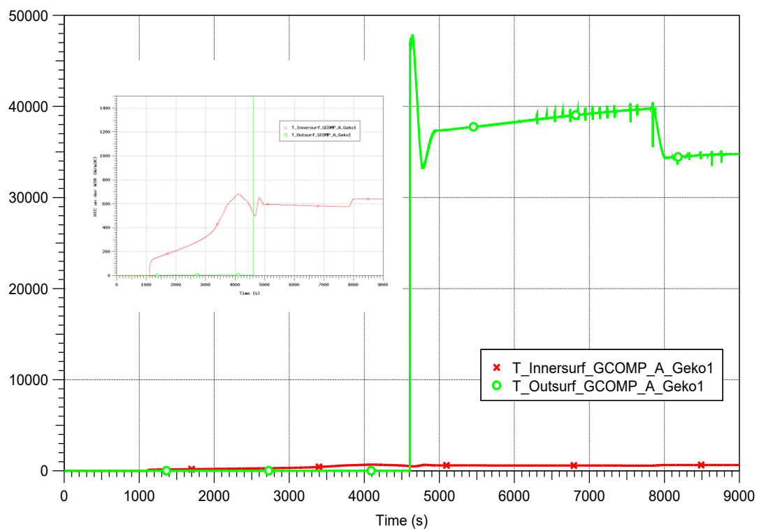
Abb. 3.109 EASY-4, Vergleich des vom GEKO-Modul berechneten Wärmeübergangskoeffizienten an der Außenseite (ALPHA A ) und an der Innenseite (ALPHA) der Wärmetauscherrohre
