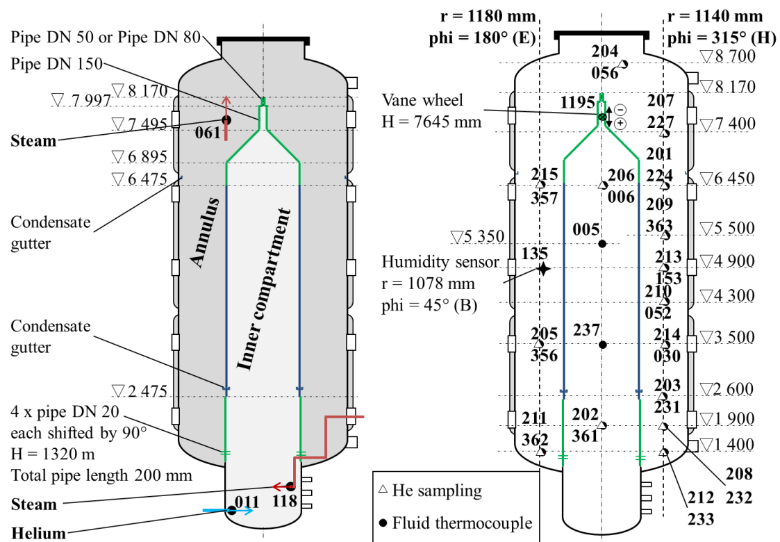
Abb. 2.3 THAI TH-29, Konfiguration des THAI-Behälters. Einbauten und Helium-/Dampfzufuhr (links). Probenahmestellen, Thermoelemente, Schaufelrad und Feuchtigkeitssensor (rechts) /SCH 23/
