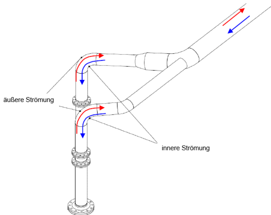
Abb. 3.73 Ausbildung von inneren (Kondensat) und äußeren (Dampf) Strömungsschichten in der Rücklaufleitung des Gebäudekondensators /WAG 17/
