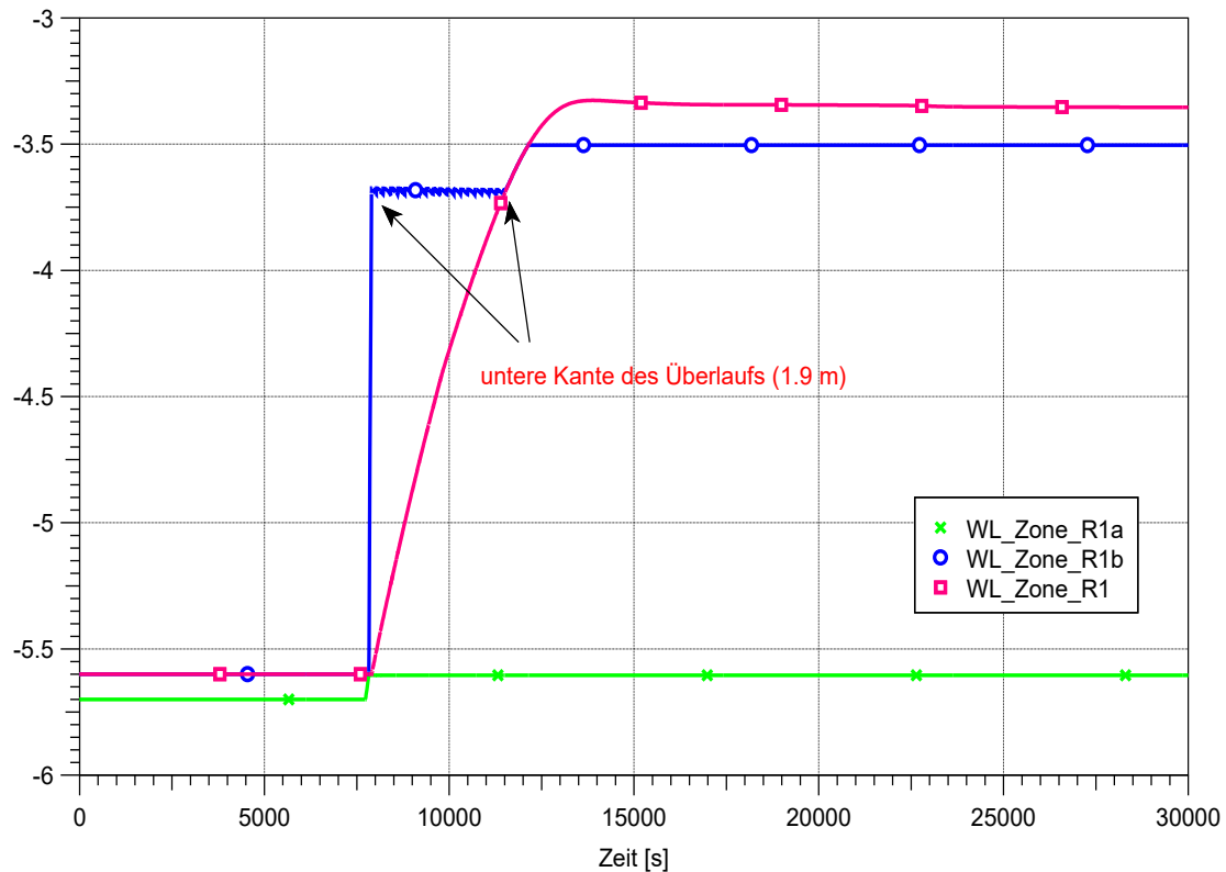
Abb. 2.104 COCOSYS, Wasserspiegel in den Kanälen der Kühlrippen (Zone R1b) und in der Spalte hinter der Seitenplatte (Zone R1b) sowie im Ausbreitungsraum (Zone R1)
