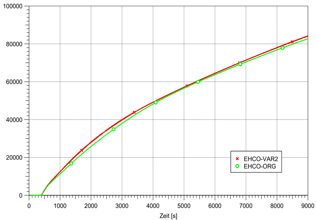
Abb. 3.106 EASY-4, Vergleich der über den NOKO übertragenen Wärme für die gekoppelte Rechnung (VAR2) und die ursprüngliche Simulation (ORG)
