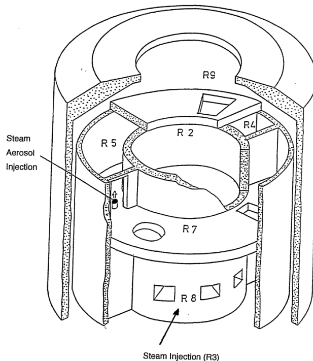
Abb. 2.57 BMC VANAM-M3, Versuchstand /KAN 93/
