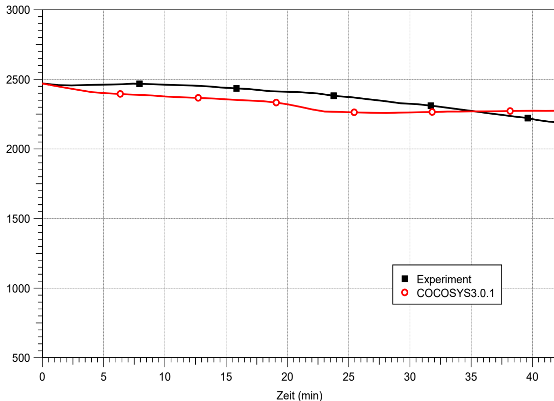
Abb. 2.83 ACE L6, Vergleich der berechneten Schmelztemperatur mit den im Experiment durch Thermolemente ermittelten Temperaturwerten
