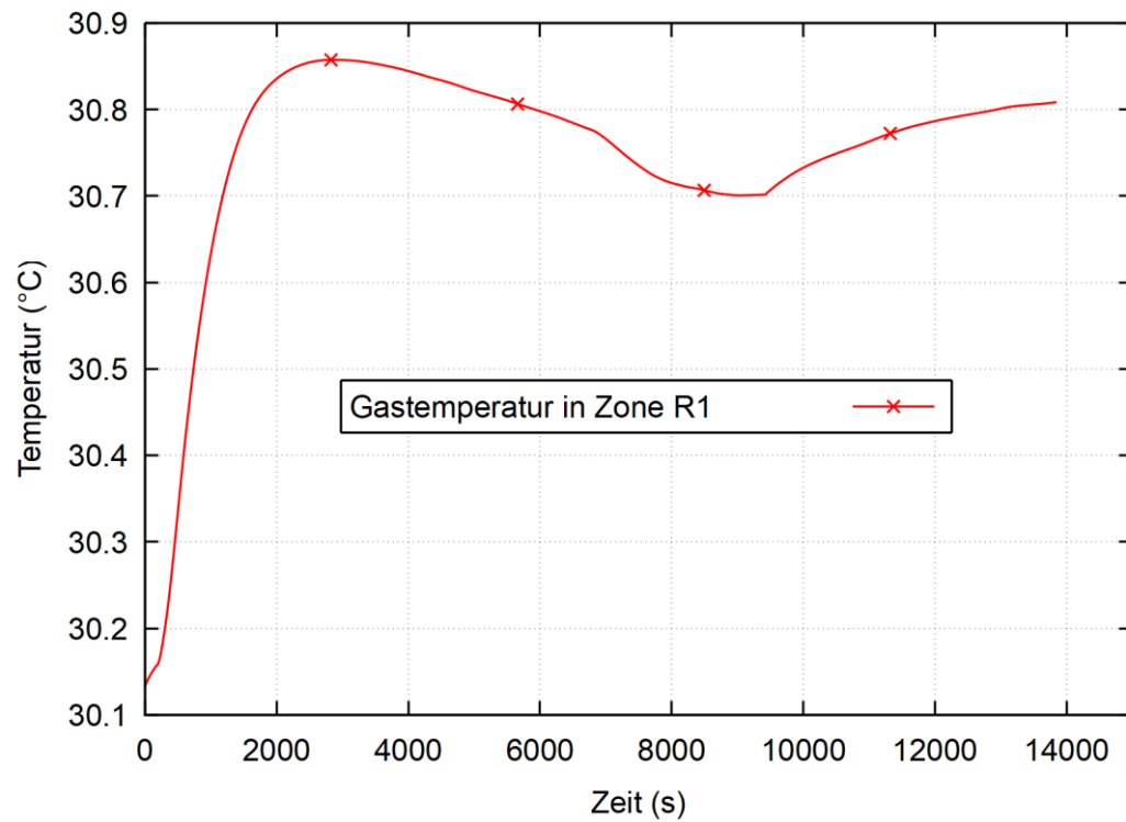
Abb. 3.48 Temperaturverlauf in COCOSYS-Zone R1 (Gasphase)
