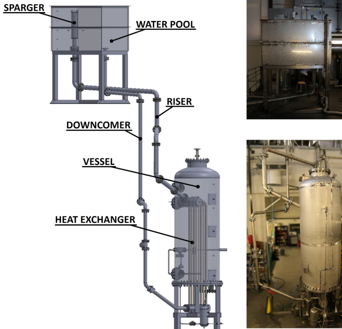
Abb. 3.69 Schema der PASI-Versuchsanlage (Kouhia, Kauppinen et al, DOI: 10.1016/j.nucengdes.2021.111417, CC BY 4.0 DEED /KOU 21/)
