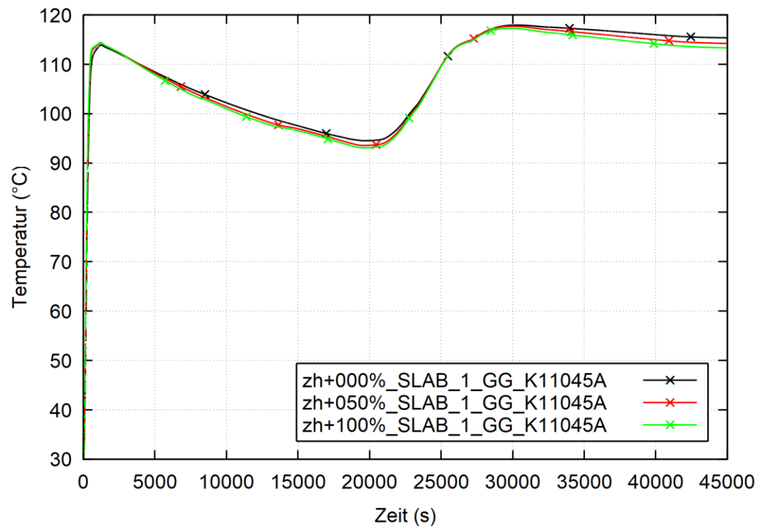
Abb. 4.3 DWR-KONVOI, COCOSYS-Rechnung: Temperatur der Stahlschale im Dom-Bereich (MBL-Fall)
