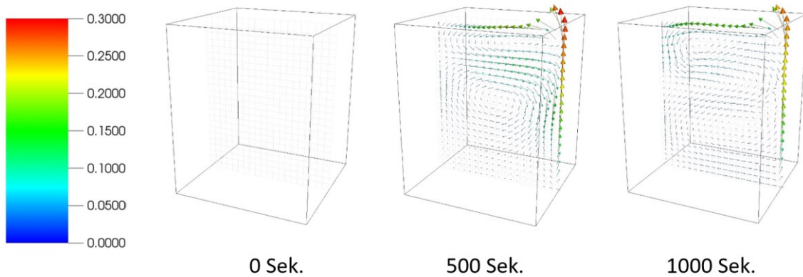
Abb. 3.9 Geschwindigkeitsfeld (in m/s) für y = 10 m bei T = 0 Sek., T = 500 Sek. und T = 1000 Sek.
