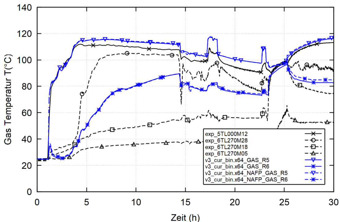
Abb. 2.59 BMC VANAM-M3, Temperaturschichtung in R6
