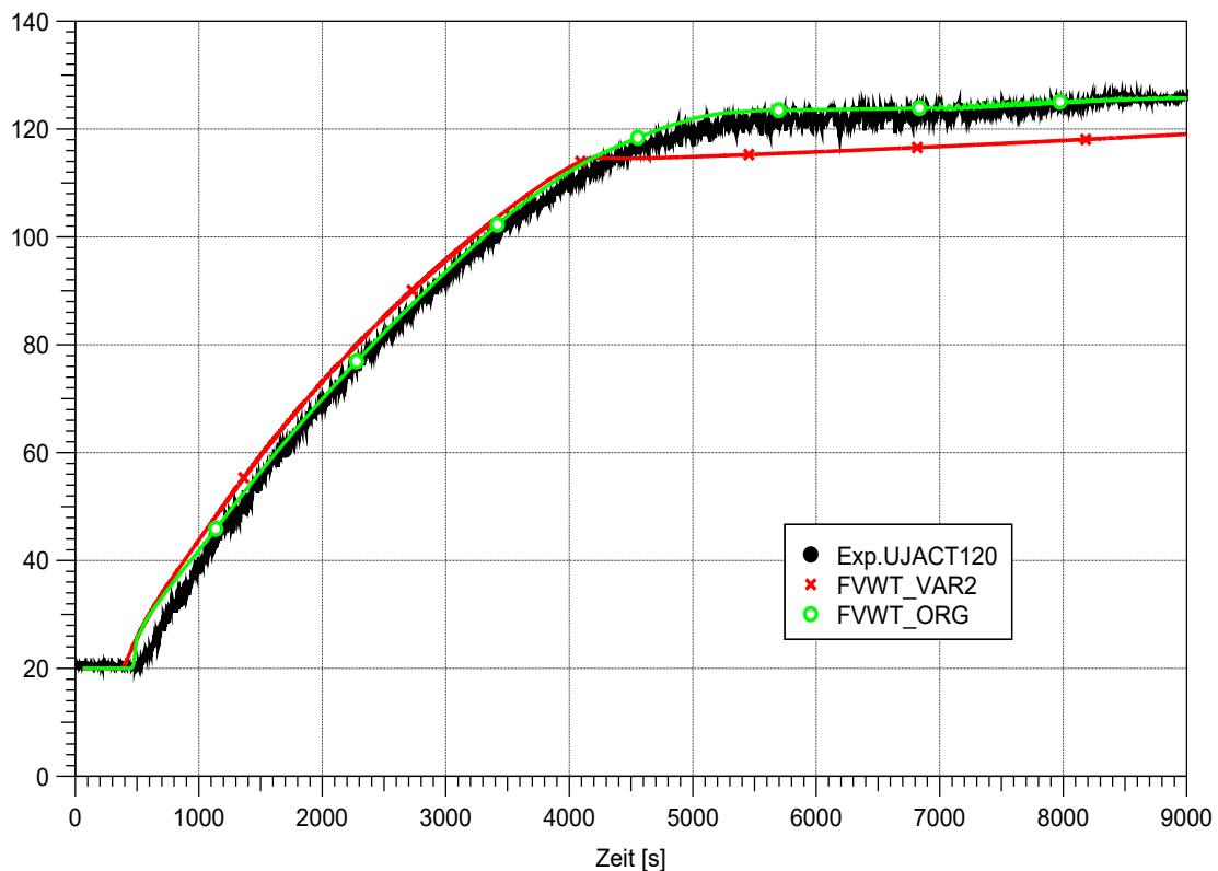
Abb. 3.105 EASY-4, Vergleich der berechneten Wassertemperaturen für die gekoppelte Variantenrechnung (VAR1) und die ursprüngliche Simulation (ORG) mit der im Experiment gemessenen Temperatur im Flutbehälter
