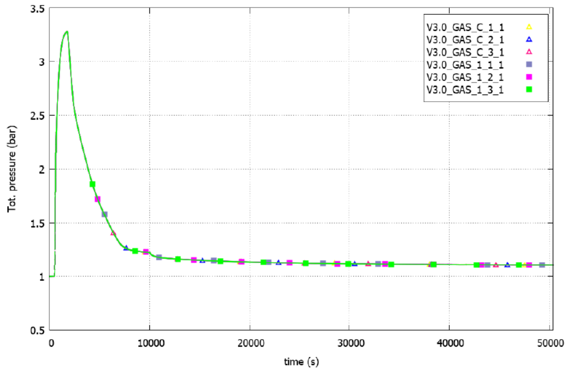
Abb. 3.58 Frühere Rechnung: Druckverlauf im Containment
