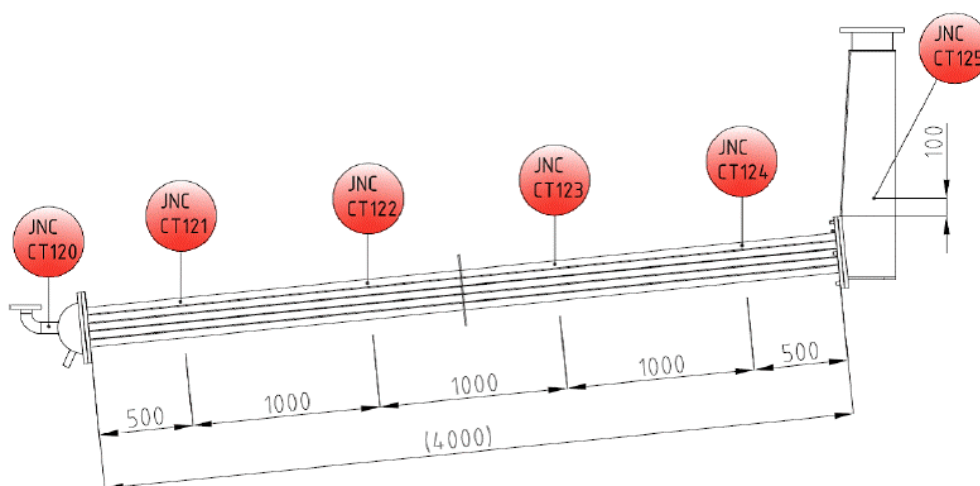
Abb. 3.75 Wärmetauscherrohre des Gebäudekondensators mit Messstellen für die Temperatur des Kühlmittels /WAG 17/
