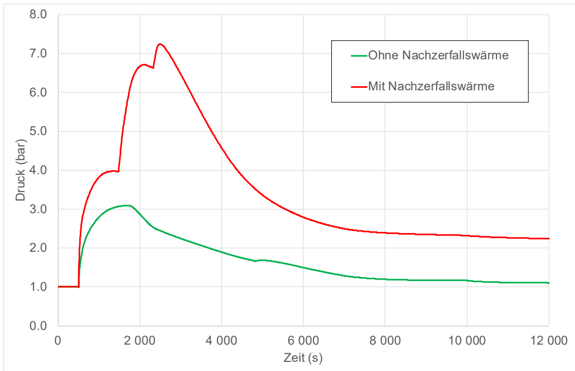
Abb. 3.65 Parameterstudie: Druckverlauf im Containment (COCOSYS-Zone C1)
