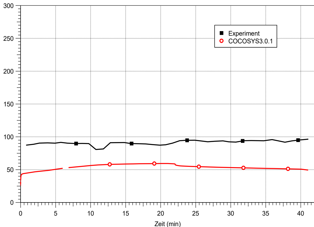
Abb. 2.80 ACE L2, Vergleich der berechneten Oberflächenverluste mit den aus dem Experiment ermittelten Leistungsverlusten durch die Schmelzeoberfläche
