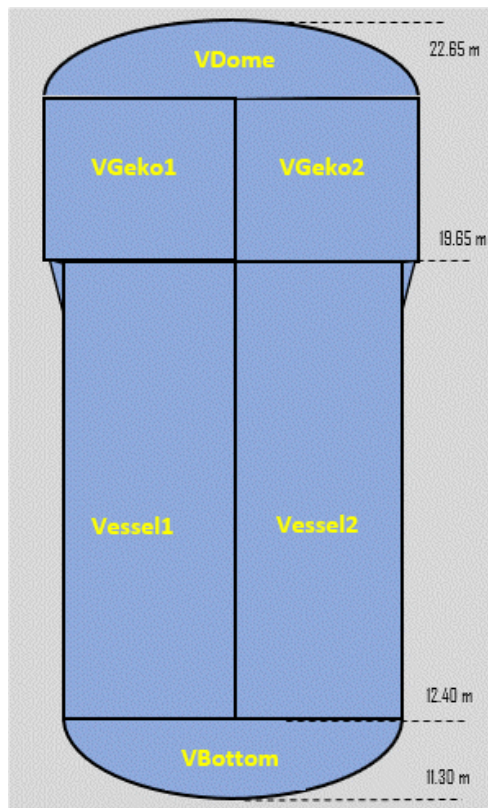
Abb. 3.74 COCOSYS-Nodalisierung des Flutbehälters der INKA-Versuchsanlage
