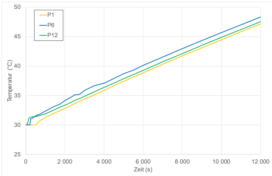
Abb. 3.27 Temperaturverlauf an unterschiedlichen Monitorpunkten (P1, P6, P12, vgl. Abb. 3.25)
