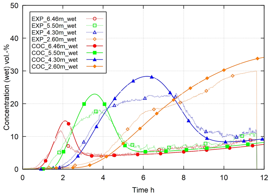
Abb. 2.7 THAI TH-29, Vergleich der gemessenen Heliumkonzentration an unterschiedlichen Messpositionen mit der COCOSYS-Rechnung
