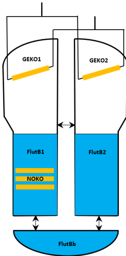
Abb. 3.99 COCOSYS-Nodalisierung des Flutbehälters für die Nachrechnungen des Experiments EASY-4 (Station blackout)
