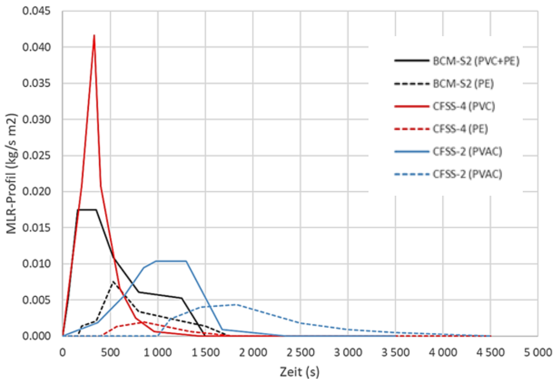
Abb. 2.113 Vergleich der MLR-Profile (PVC: rot, PE/PVC: schwarz, FRNC: blau)
