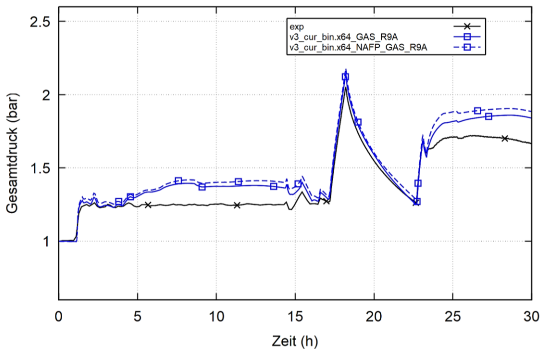
Abb. 2.58 BMC VANAM-M3, Gesamtdruck
