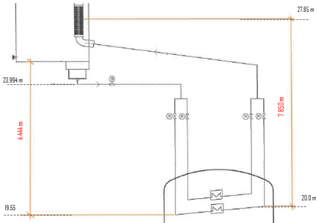
Abb. 3.77 Höhendifferenzen zwischen Gebäudekondensator und Absetzbecken
