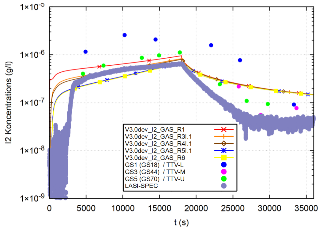
Abb. 2.44 THAI Iod-33, Iodkonzentration in unterschiedlichen Raumbereichen in Rechnung (Linien) und Experiment (Punkte)
