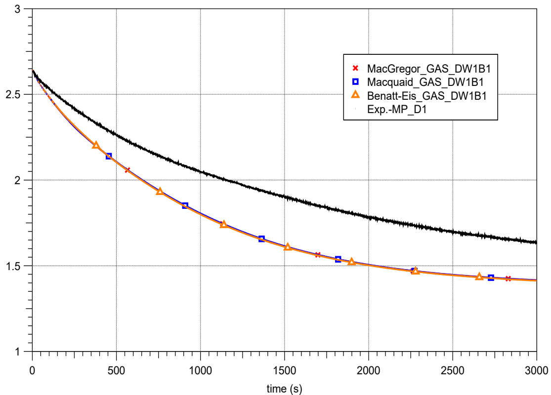
Abb. 2.24 PANDA ST3_2, Vergleich zwischen dem berechneten Druck und dem während des Versuchs gemessenen Druck
