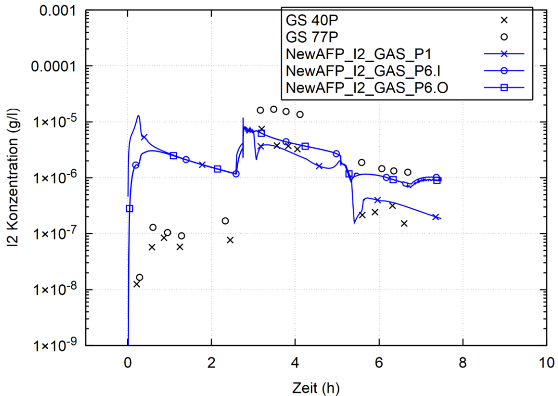
Abb. 2.39 THAI Iod-32, I 2 -Konzentration in der Atmosphäre des PAD
