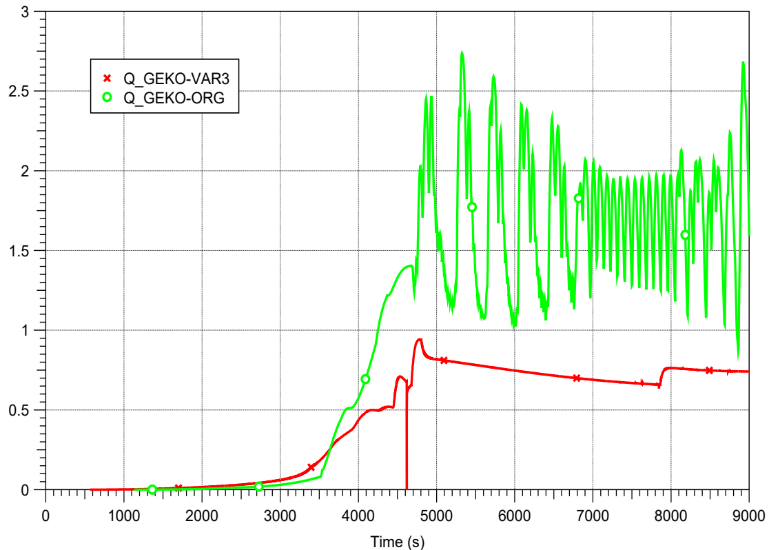
Abb. 3.110 EASY-4, Vergleich der vom GEKO berechneten Kühlleistung mit der in der ursprünglichen ATHLET/COCOSYS-Simulation (ORG) ermittelten Kühlleistung
