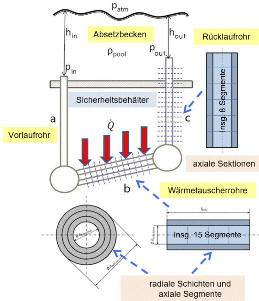
Abb. 3.76 Nodalisierungsschema des Rücklaufrohres und der Wärmetauscherrohre des Gebäudekondensators
