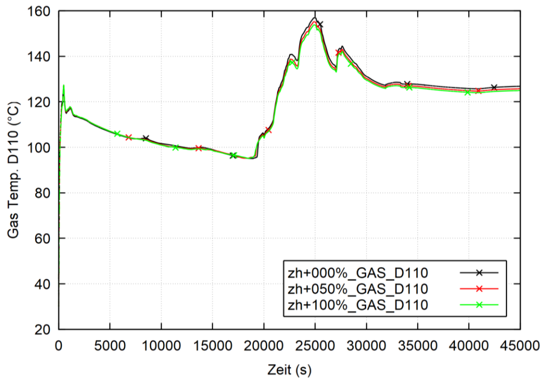
Abb. 4.2 DWR-KONVOI, COCOSYS-Rechnung: Gastemperatur im Dombereich (MBL-Fall)
