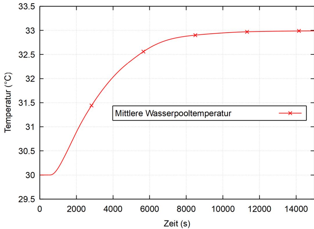
Abb. 3.61 Aktuelle Rechnung: Temperaturverlauf im Wasserpool (COCOSYS-Zone R1)
