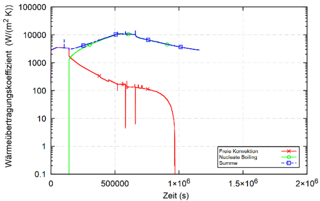
Abb. 3.23 Zeitverlauf der Wärmeübertragungskoeffizienten an der untersten Zone bei feiner Nodalisierung im Fall stark beheizter Struktur (unterste Struktur)
