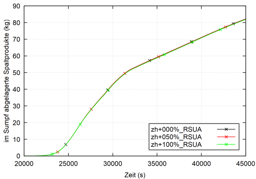
Abb. 4.7 DWR-KONVOI, COCOSYS-Rechnung: Masse abgelagerter Spaltprodukte im Sumpf (MBL-Fall)
