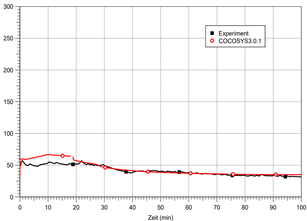
Abb. 2.93 ACE L8, Vergleich der berechneten Oberflächenverluste mit den im Experiment ermittelten Leistungsverlusten durch die Schmelzeoberfläche
