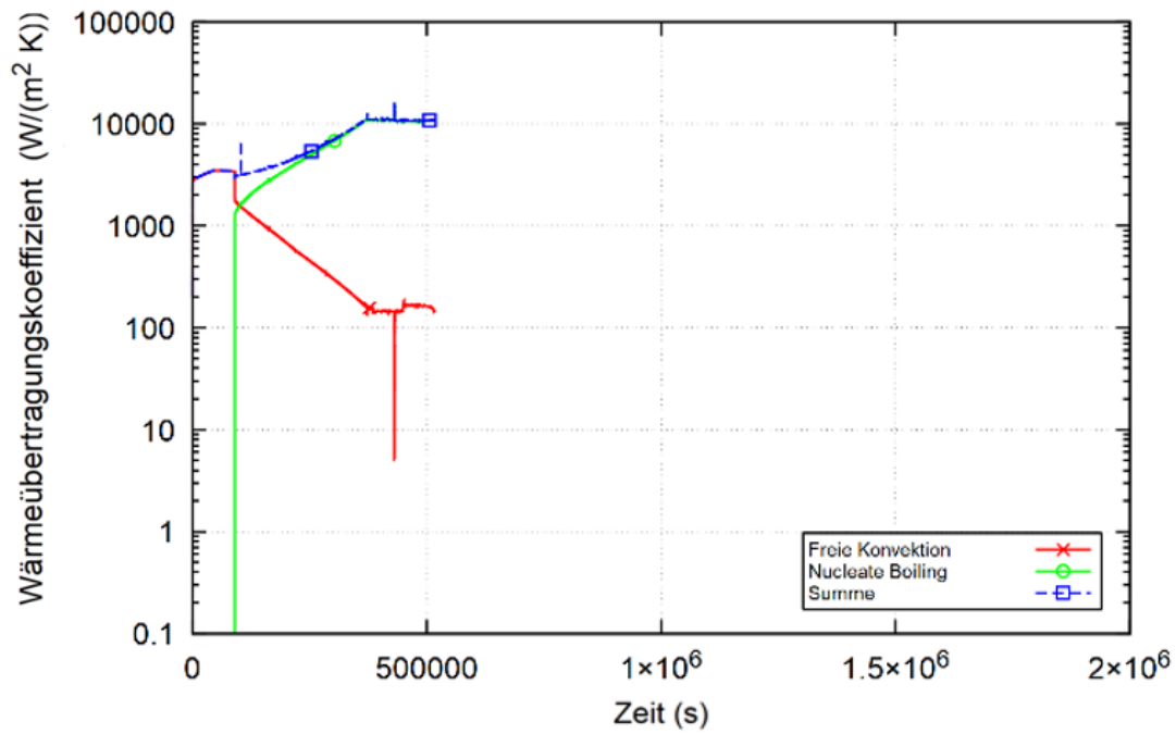
Abb. 3.22 Zeitverlauf der Wärmeübertragungskoeffizienten bei feinere Nodalisierung im Fall stark beheizter Struktur (dritte Struktur von oben)
