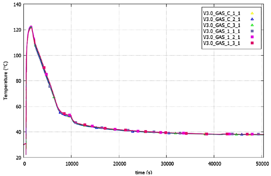
Abb. 3.60 Frühere Rechnung /BEC 18/: Temperaturverlauf im Containment
