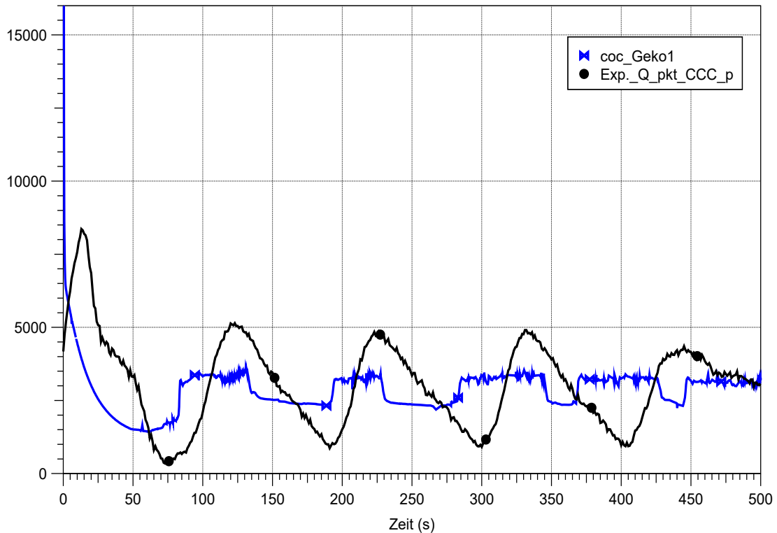
Abb. 3.81 CCC_040_025_100_01, Vergleich der berechneten Kühlleistung mit der im Experiment ermittelten Kühlleistung des Gebäudekondensators
