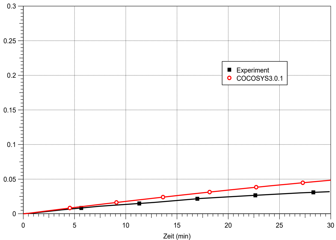
Abb. 2.87 ACE L7, Vergleich der berechneten Betonerosionstiefe in axialer Richtung mit dem im Experiment durch Thermoelemente ermittelten Erosionsfortschritt
