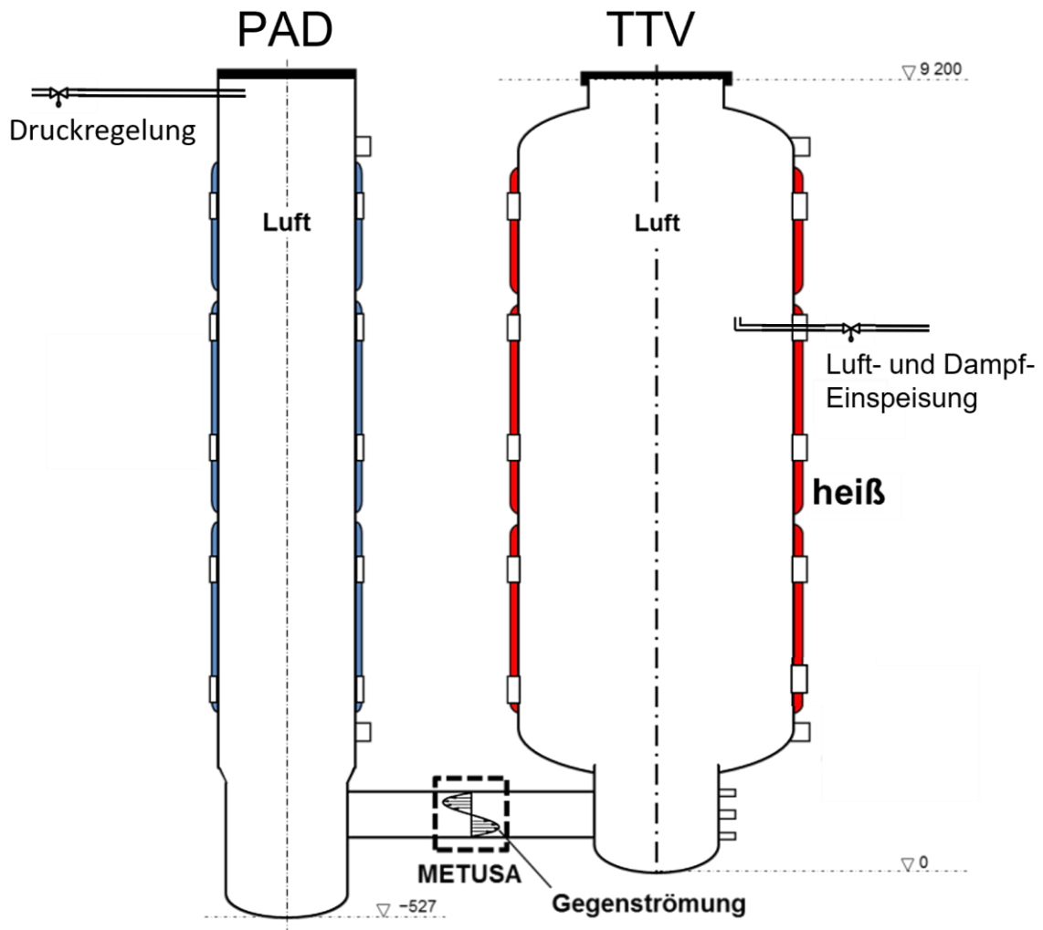
Abb. 2.29 THAI TH-35, Schema der Testkonfiguration der Versuchsanlage THAI +
