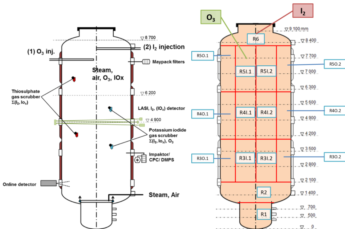
Abb. 2.40 THAI Iod-37, Versuchskonfiguration (links) und COCOSYS-Nodalisierung mit Kennzeichnung der Zonen (rechts)
