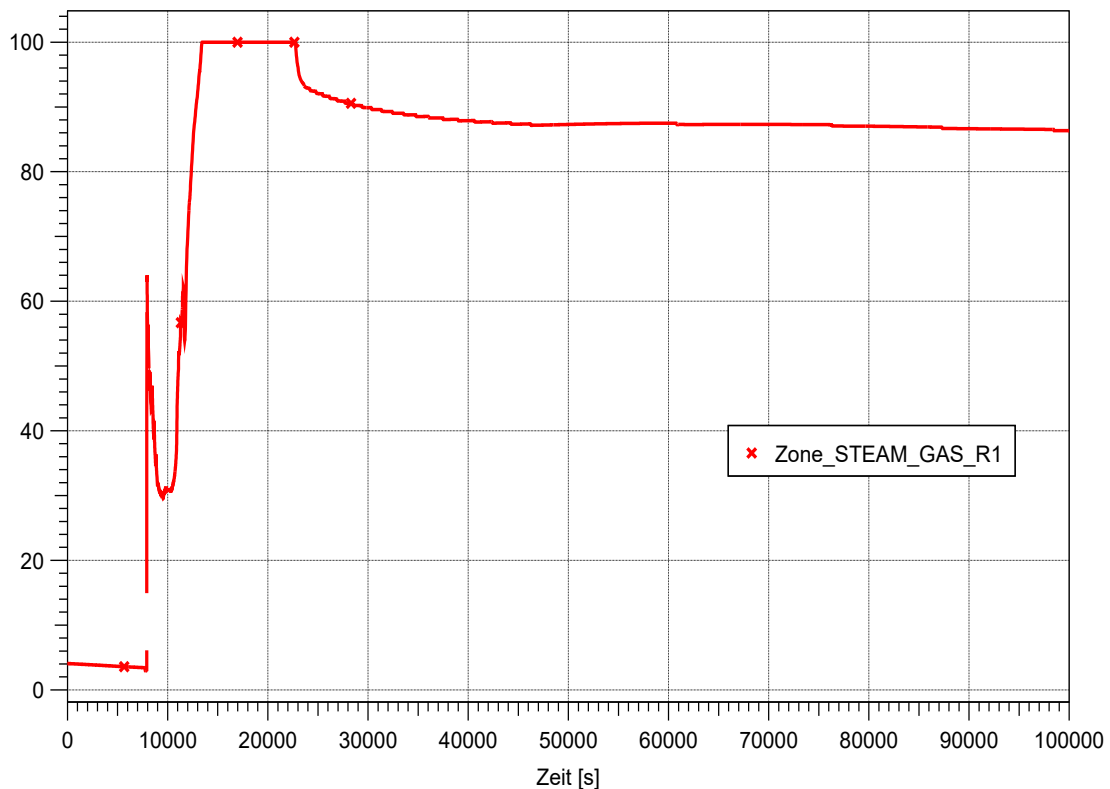
Abb. 2.111 COCOSYS, Dampfkonzentration im Ausbreitungsraum (Zone R1)
