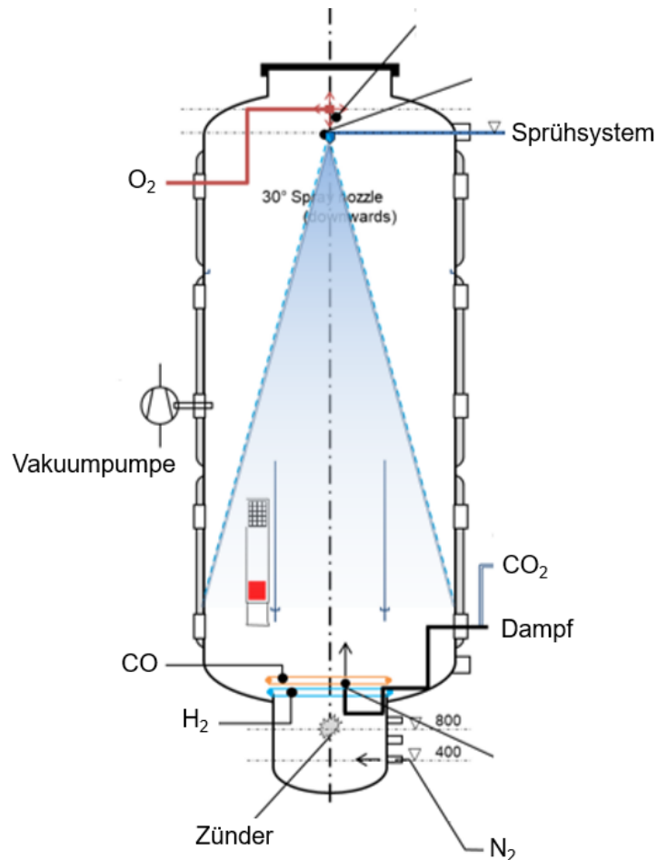
Abb. 2.12 Darstellung der Versuchsanlage THAI für den Versuch THAI HR-57
