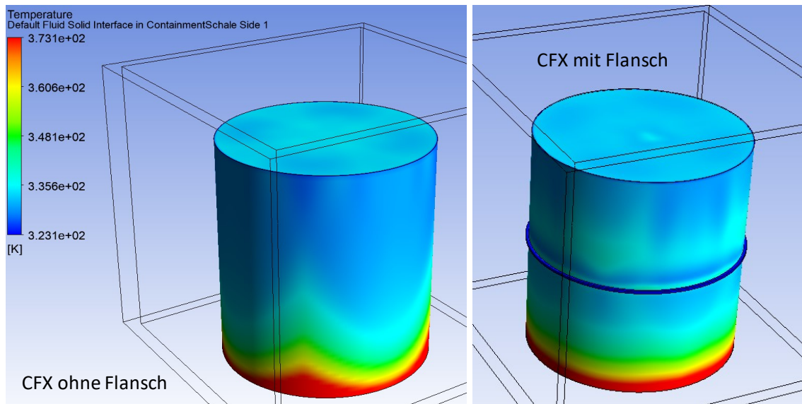
Abb. 3.44 Temperaturen an den Containment-Außenseiten mit und ohne Flansch
