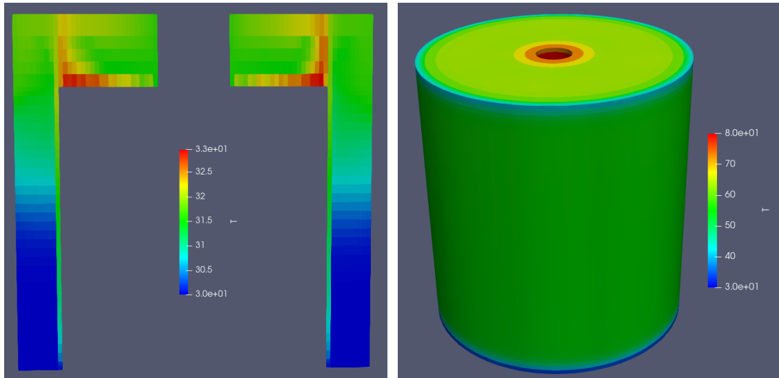
Abb. 3.64 Aktuelle Rechnung: Temperaturen in °C im Wasserpool (links) und an der Containment-Außenseite (rechts) zum Zeitpunkt t = 2.000 \text{ s}
