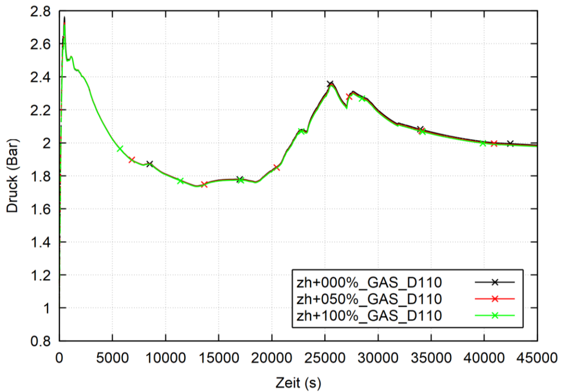
Abb. 4.1 DWR-KONVOI, COCOSYS-Rechnung: zeitlicher Verlauf des SHB-Drucks (MBL-Fall)
