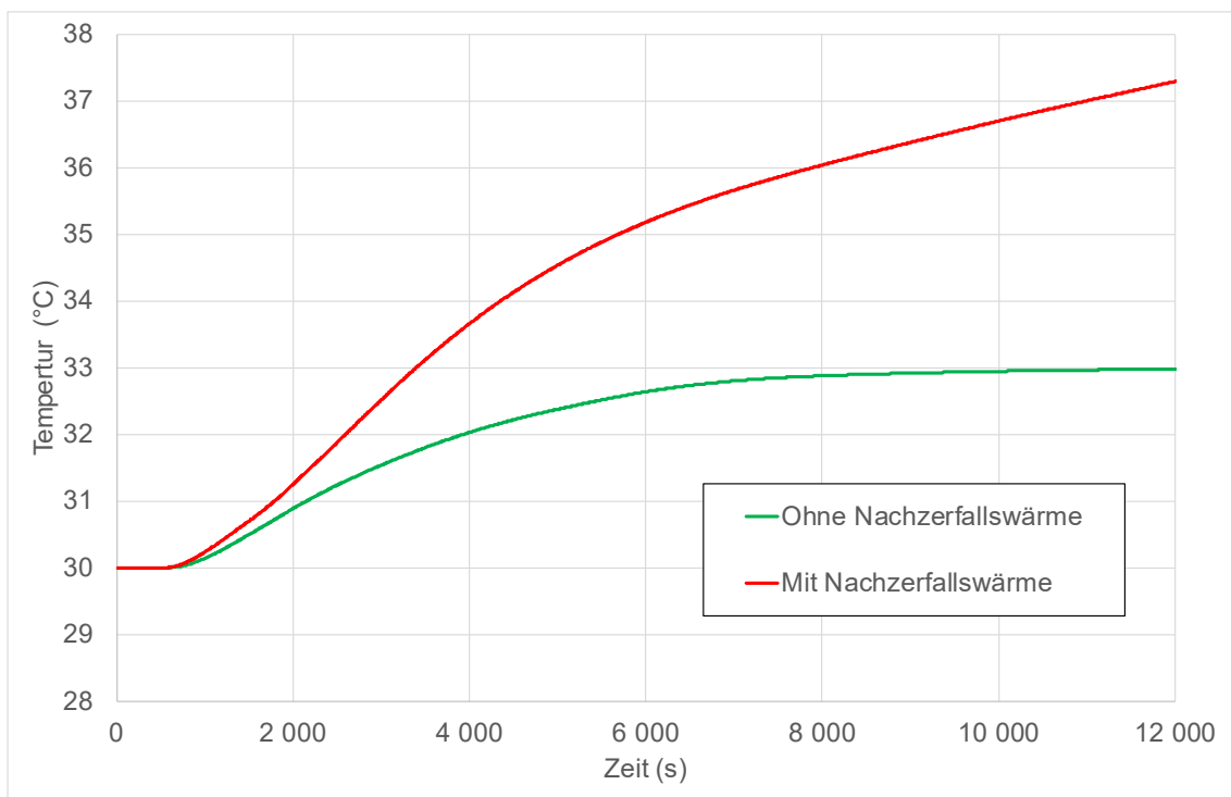
Abb. 3.68 Parameterstudie: Mittlere Pooltemperatur
