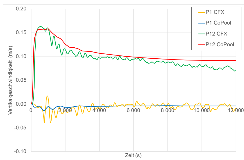
Abb. 3.40 Vergleich der mit CoPool und CFX berechneten vertikalen Strömungsgeschwindigkeiten an den Monitorpunkten P1 und P12
