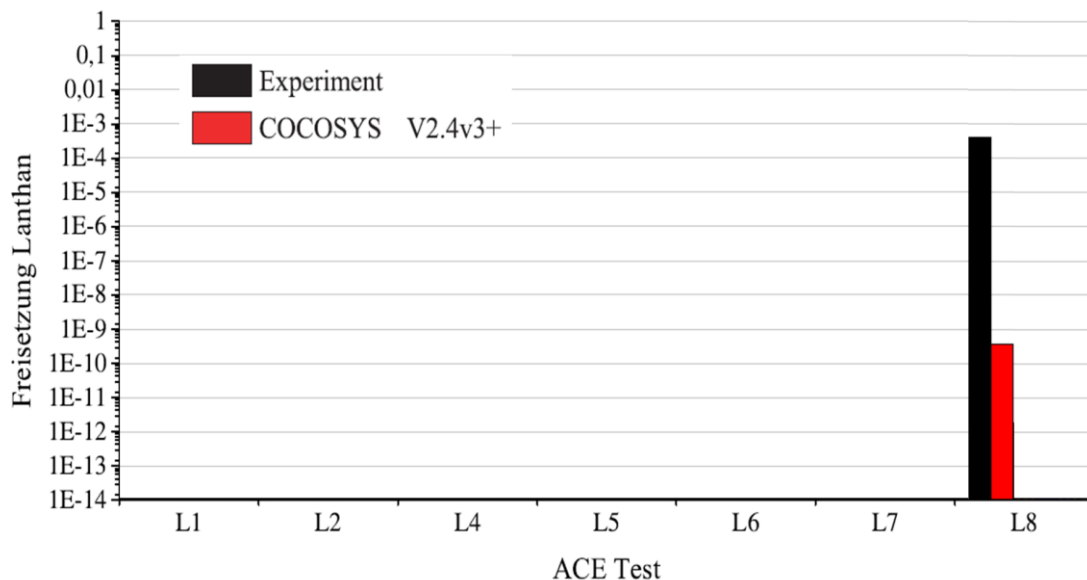
Abb. 2.95 ACE L8, Vergleich der von COCOSYS v2.4v3+ berechneten Freisetzungsrates von Lanthan (roter Balken) mit der im Experiment ermittelten anteiligen Lanthanfreisetzung (schwarzer Balken) /AGE 17/
