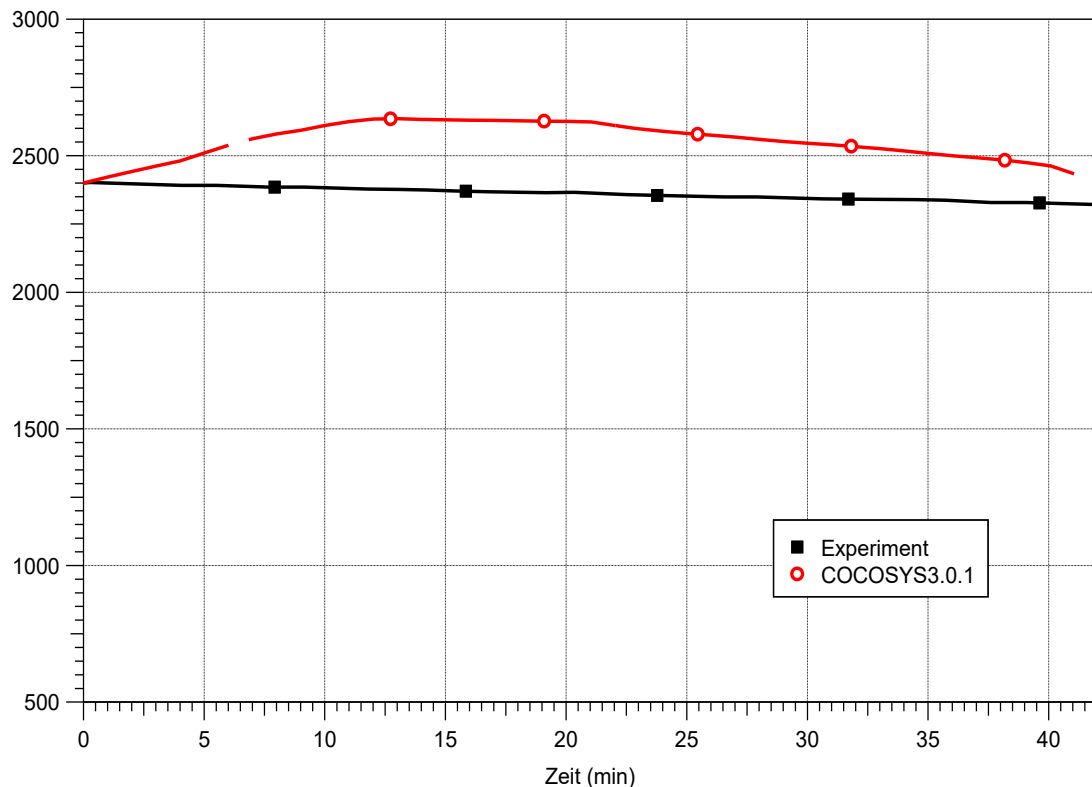
Abb. 2.79 ACE L2, Vergleich der berechneten Schmelztemperatur mit den im Experiment durch Thermoelemente ermittelten Temperaturwerten
