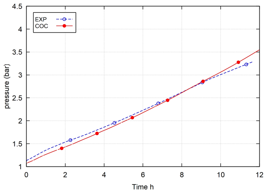
Abb. 2.5 THAI TH-29, Vergleich des gemessenen Drucks mit der COCOSYS-Rechnung
