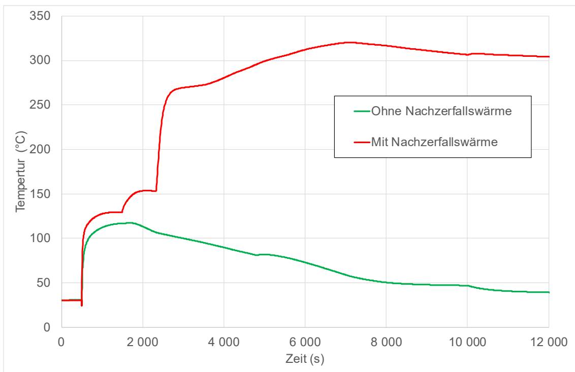
Abb. 3.66 Parameterstudie: Temperaturverlauf im Containment (COCOSYS-Zone C1)
