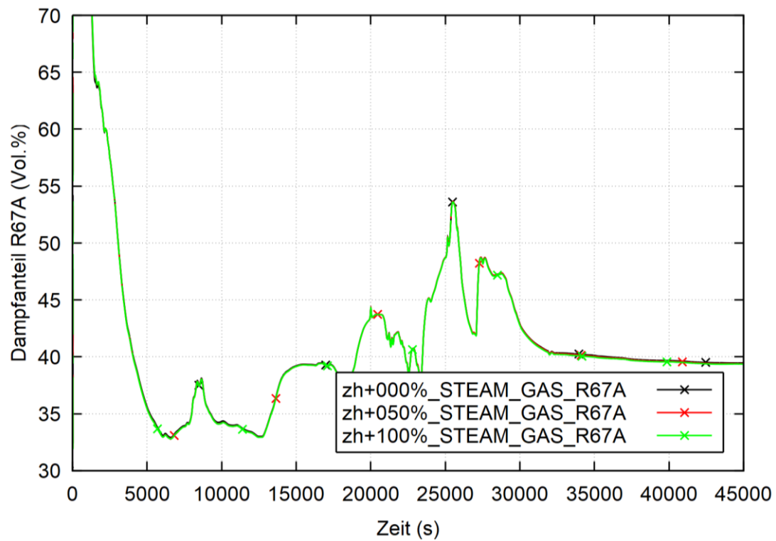
Abb. 4.5 DWR-KONVOI, COCOSYS-Rechnung: zeitlicher Verlauf der Dampfkonzentration in den Anlagenräumen (MBL-Fall)
