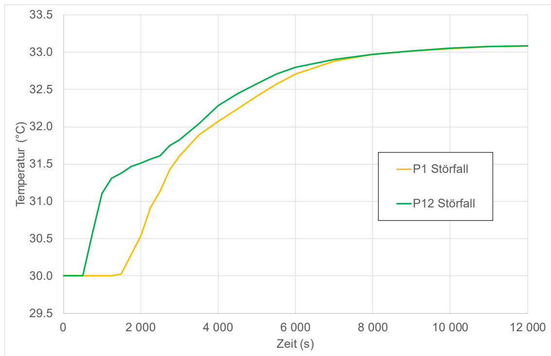
Abb. 3.63 Aktuelle Rechnung: Temperaturverlauf an den Monitorpunkte P1 und P12 im Wasserpool
