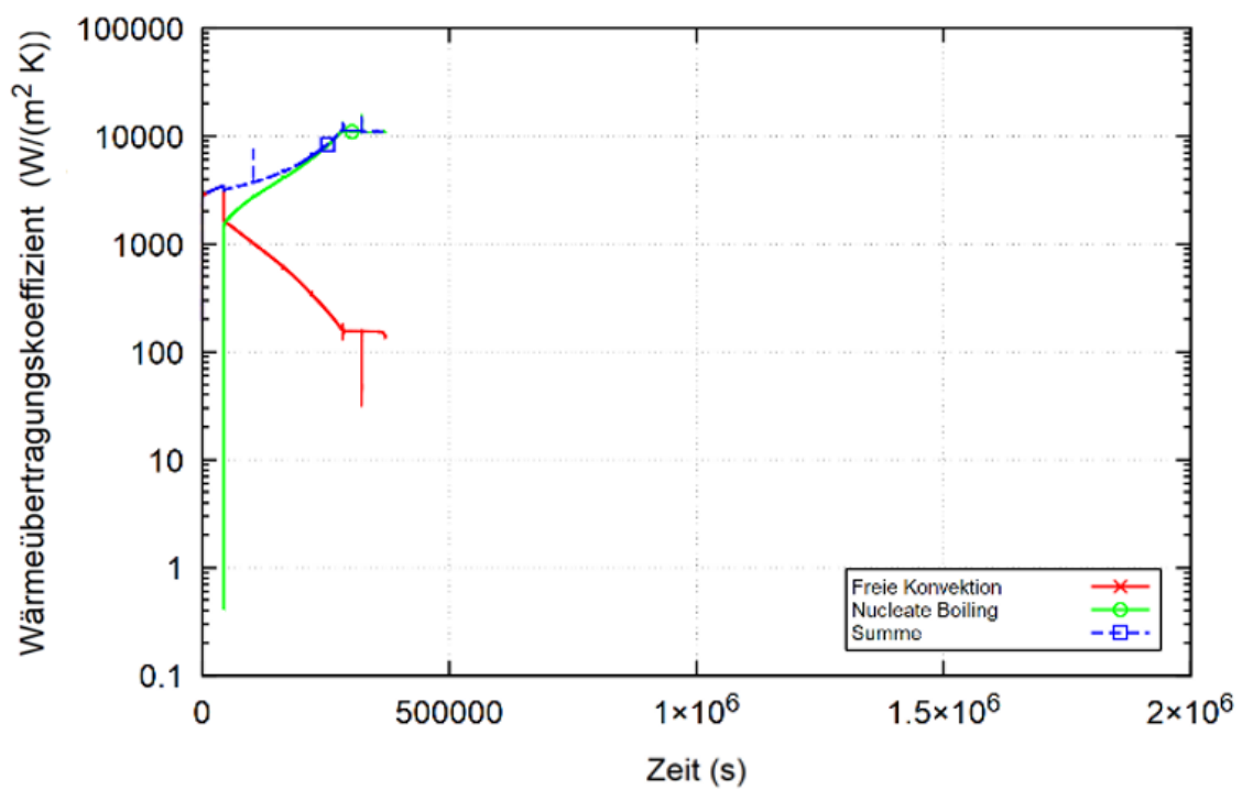
Abb. 3.21 Zeitverlauf der Wärmeübertragungskoeffizienten bei feiner Nodalisierung im Fall stark beheizter Struktur (zweite Struktur von oben)
