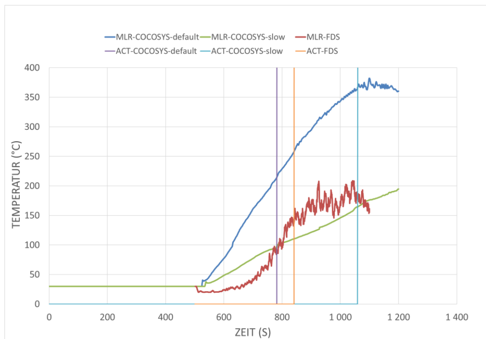
Abb. 2.125 Vergleich der Abbrandrate (oben) und Temperatur in der Nähe des Sprinklers (unten) der COCOSYS- und FDS-Rechnungen
