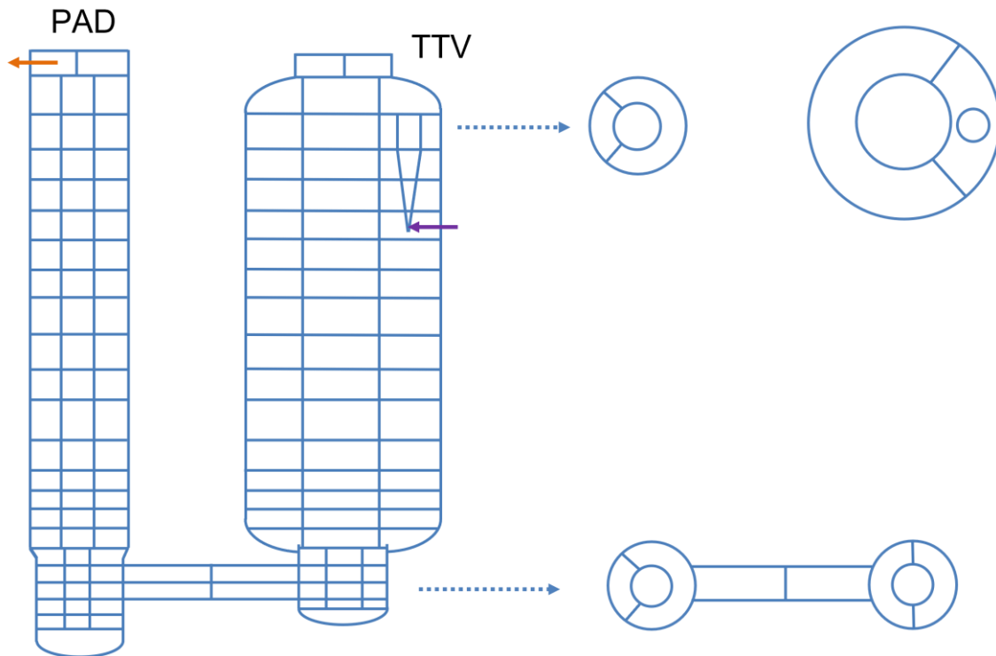
Abb. 2.31 THAI TH-35, COCOSYS-Nodalisierung für die Voruntersuchungen zum Gegenströmungsversuch
