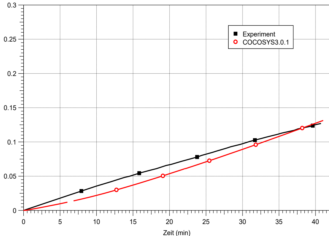
Abb. 2.78 ACE L2, Vergleich der berechneten Betonerosionstiefe in axialer Richtung mit dem im Experiment durch Thermoelemente ermittelten Erosionsfortschritt
