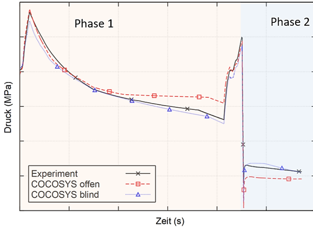
Abb. 2.15 Druckverlauf im TTV im Experiment THAI HR-57, in der blinden Vorausrechnung und offenen Nachrechnung
