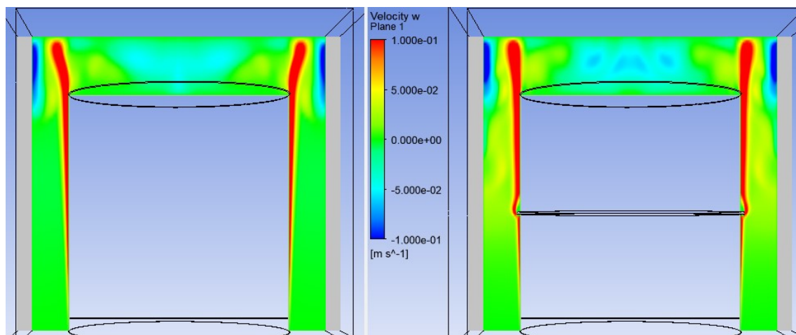
Abb. 3.41 Vergleich der vertikalen Strömungsgeschwindigkeiten zum Zeitpunkt t = 500 s ohne Flansch (links) und mit Flansch (rechts)
