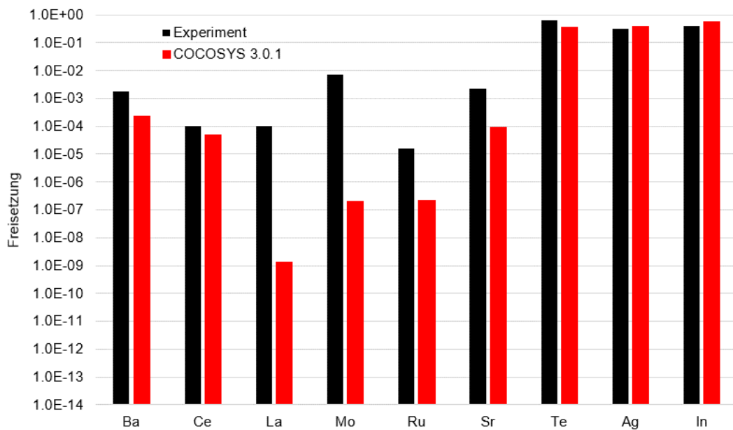
Abb. 2.85 ACE L6, Vergleich der von COCOSYS 3.0.1 berechneten Freisetzung von Spezies (rote Balken) mit der im Experiment ermittelten, anteiligen Freisetzung von Spezies (schwarzer Balken)
