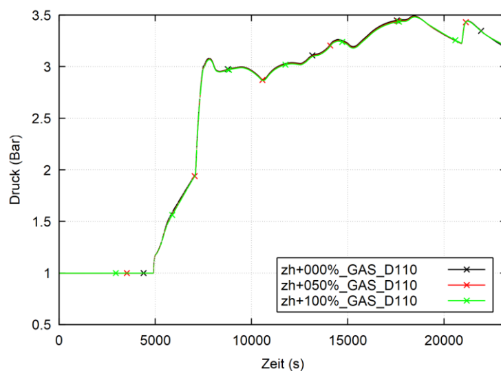
Abb. 4.10 DWR-KONVOI, COCOSYS-Rechnung: Zeitlicher Verlauf des SHB-Drucks
