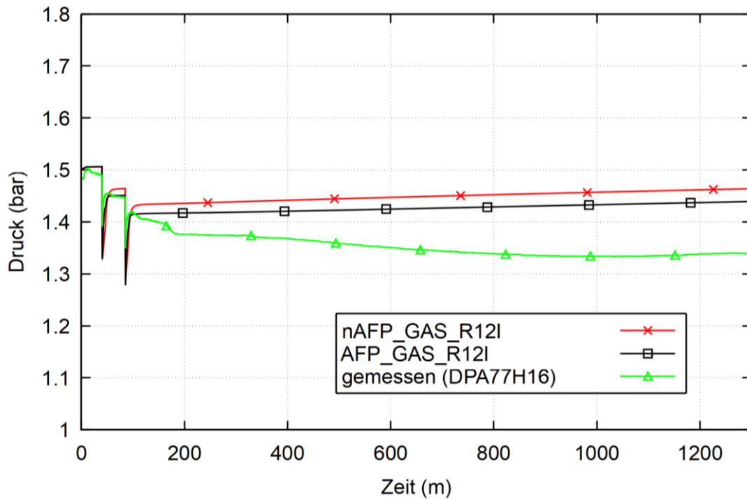
Abb. 2.49 THAI AW-4, berechneter Druckverlauf während der ersten Rechnungen
