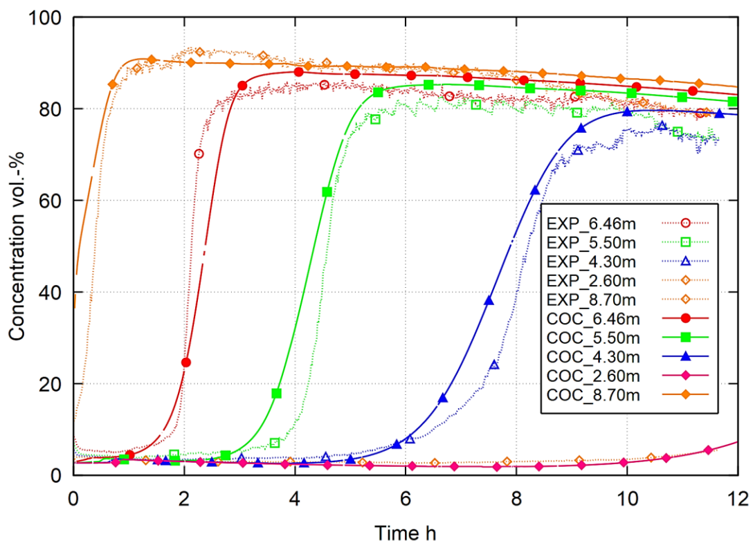
Abb. 2.6 THAI TH-29, Vergleich der gemessenen Dampfkonzentration an unterschiedlichen Messpositionen mit der COCOSYS-Rechnung
