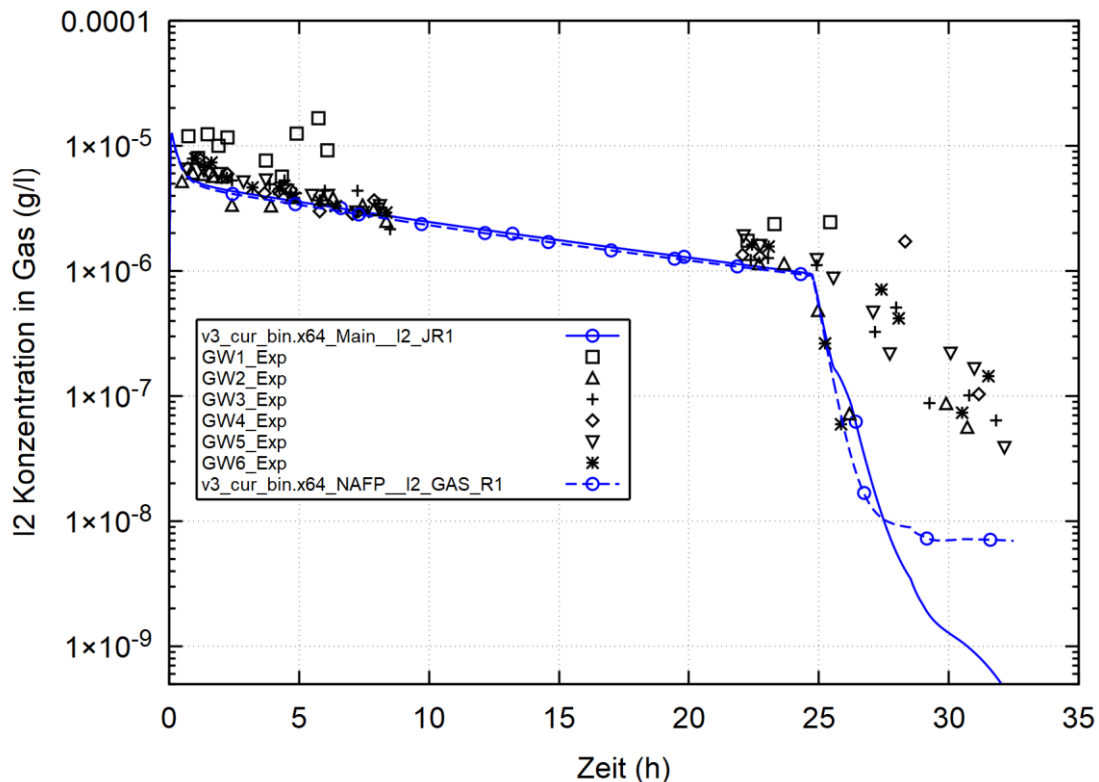
Abb. 2.65 THAI Iod-09, I_2 -Konzentration in der Gasphase
