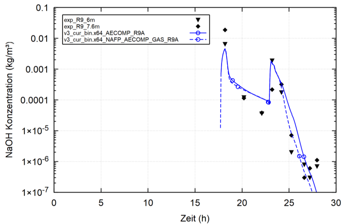
Abb. 2.62 BMC VANAM-M3, Aerosolkonzentration in R9
