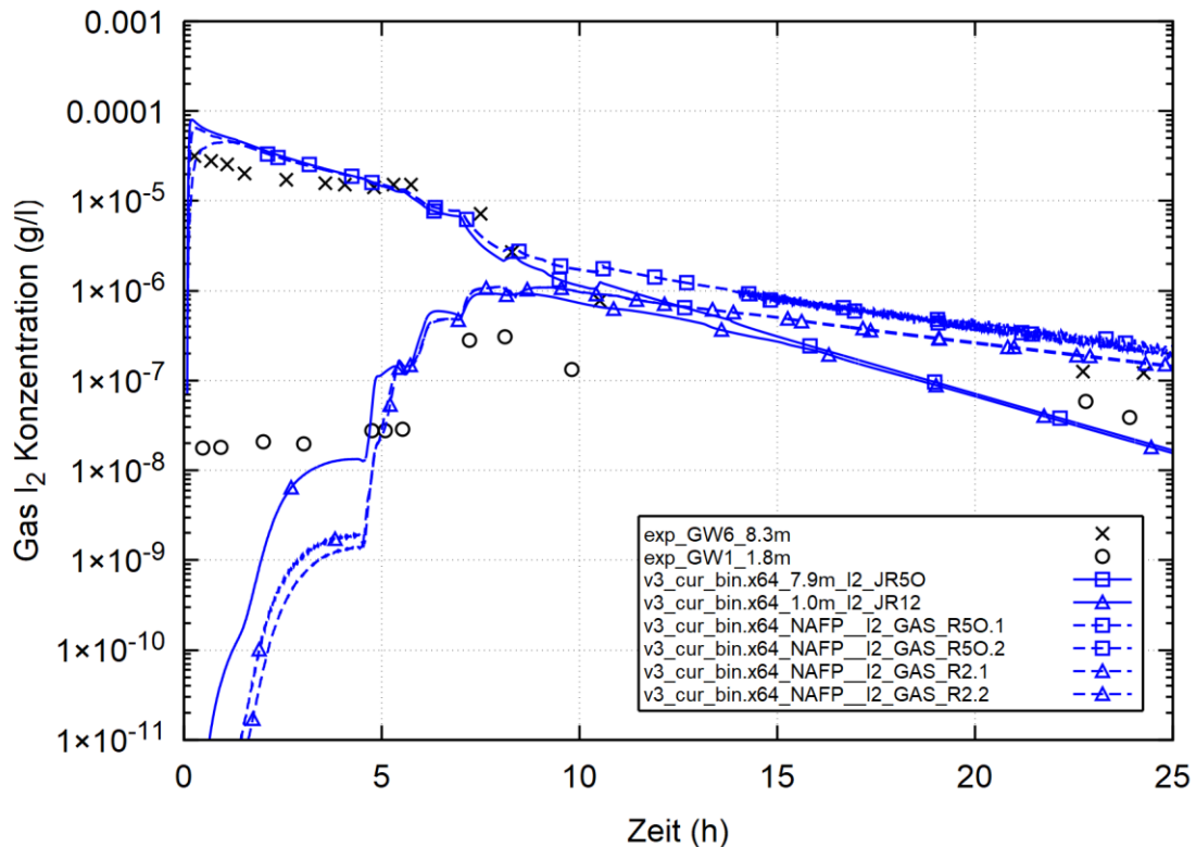
Abb. 2.70 THAI Iod-11, Iodkonzentration auf verschiedenen Höhen des THAI-Behälters
