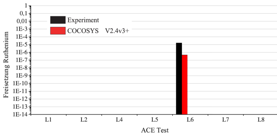
Abb. 2.86 ACE L6, Vergleich der von COCOSYSv2.4v3+ berechneten Freisetzungsrates von Ruthenium (roter Balken) mit der im Experiment ermittelten Freisetzungsrates von Ruthenium (schwarzer Balken) /AGE 17/
