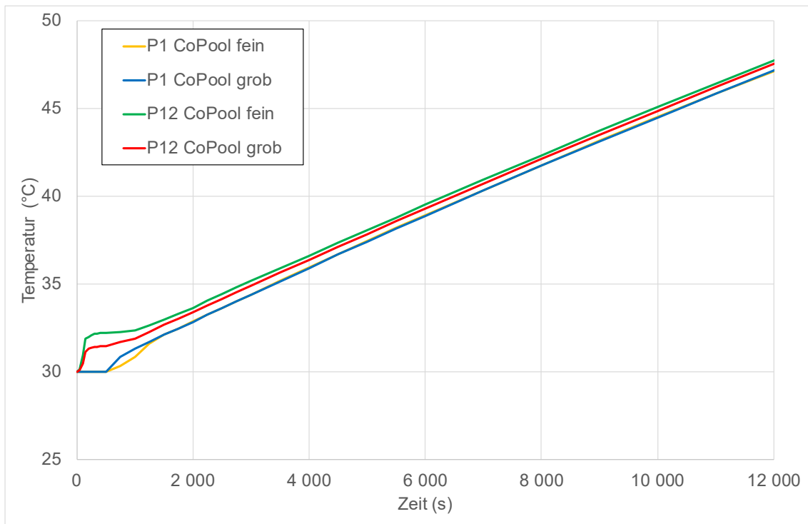
Abb. 3.30 Einfluss der Gitterfeinheit auf den Temperaturverlauf an den Monitorpunkten P1 und P12 (vgl. Abb. 3.25)
