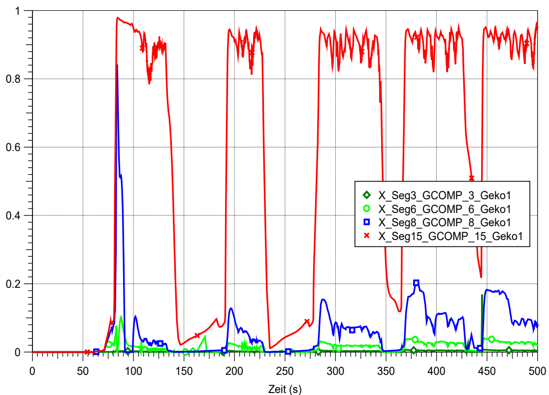
Abb. 3.84 CCC_040_025_100_01, berechneter volumetrischer Dampfgehalt entlang der WTR des Gebäudekondensators
