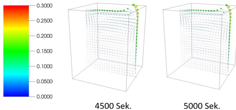
Abb. 3.12 Geschwindigkeitsfeld (in m/s) für y = 10 m bei T = 4500 Sek. und T = 5000 Sek.
