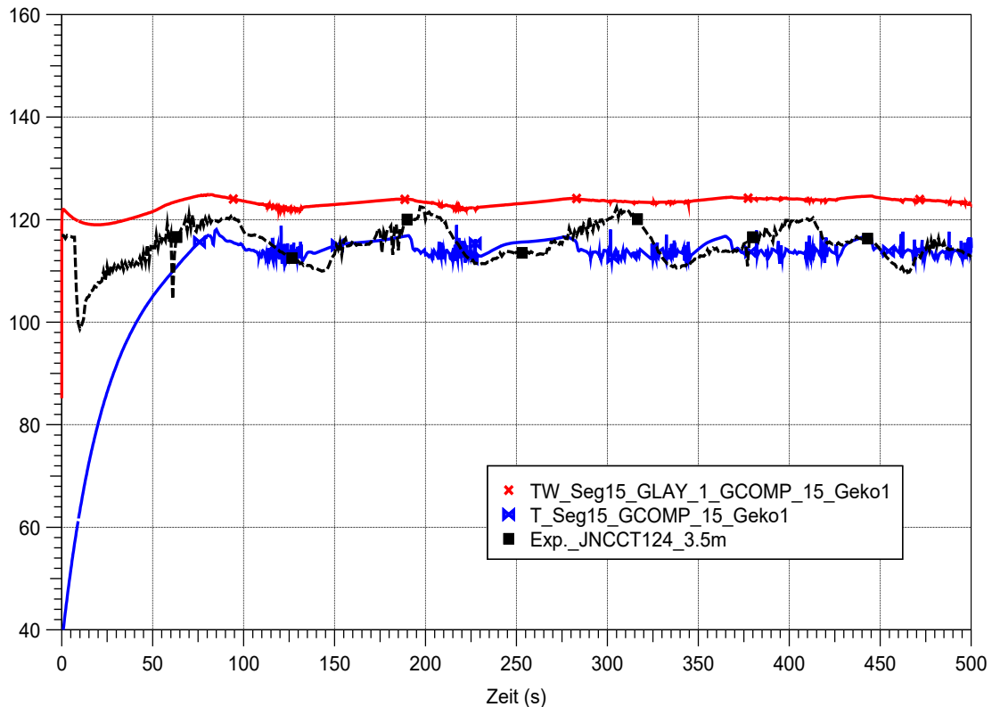
Abb. 3.83 CCC_040_025_100_01, Vergleich der berechneten Kühlmitteltemperatur (Seg_15) mit der im Experiment gemessenen Kühlmitteltemperatur im Wärmetauscherrohr sowie der Wandtemperatur
