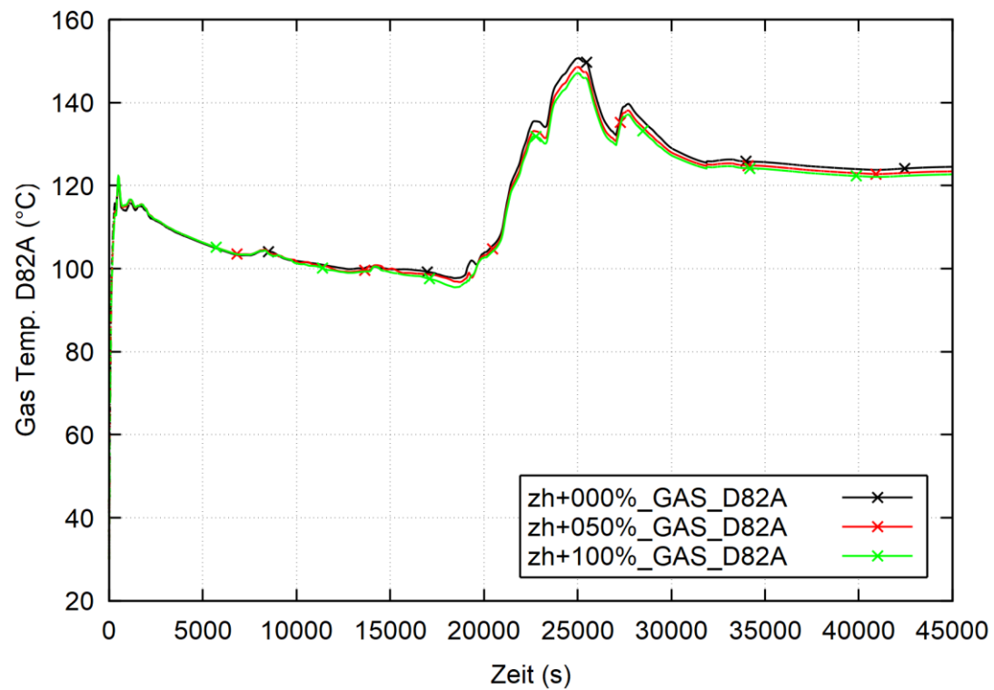
Abb. 4.4 DWR-KONVOI, COCOSYS-Rechnung: Gastemperatur im Dom bei 41 m
