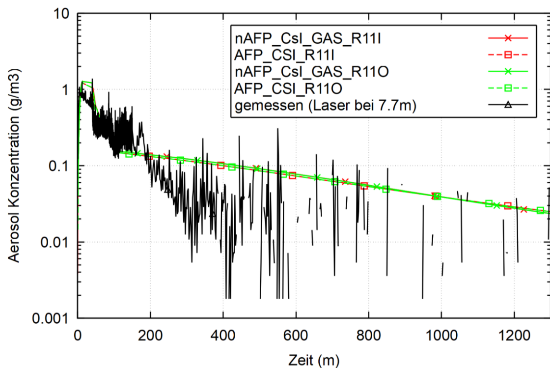
Abb. 2.56 THAI AW-4, Unterschied der Aerosolkonzentrationen auf 4,9 m Höhe (andere Tropfengröße)
