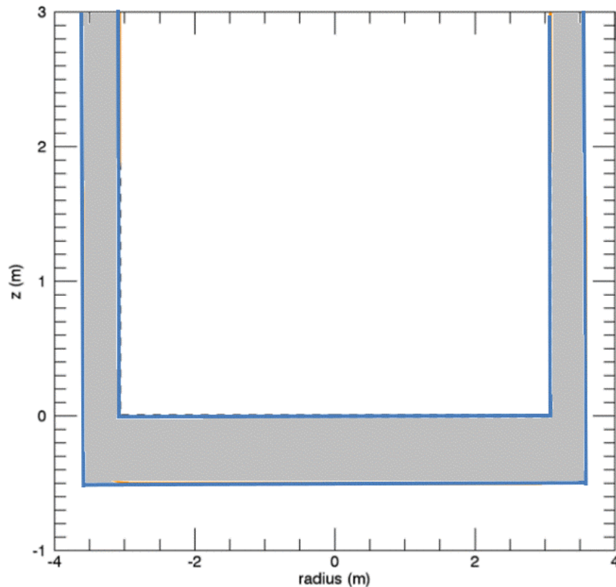
Abb. 2.102 COCOSYS, Definition der inneren Kontur zwischen Kernschmelze und Opfermaterial in Form einer 2D-Punkteschar ( r , z -Koordinaten)
