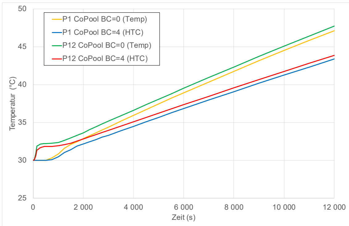
Abb. 3.32 Einfluss der Randbedingung auf den Temperaturverlauf an den Monitorpunkten P1 und P12
