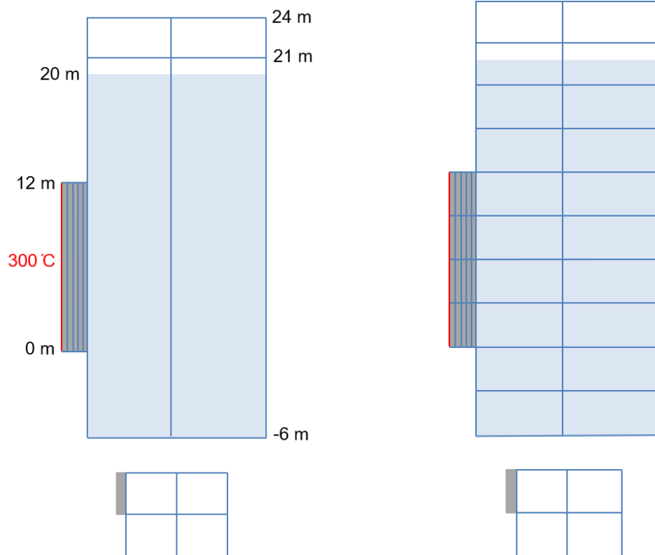
Abb. 3.15 1-Zonen-Nodalisierung (links) und 10-Zonen-Nodalisierung (rechts)
