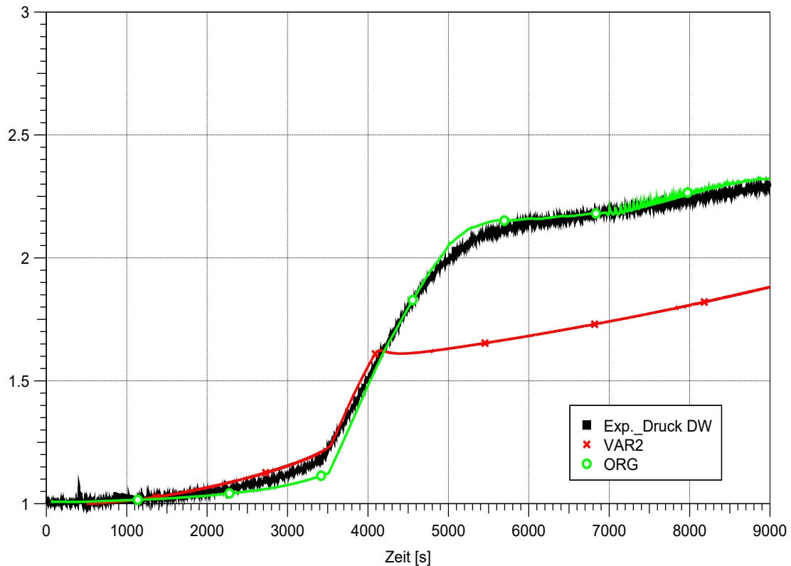
Abb. 3.104 EASY-4, Vergleich des berechneten Druckes für die gekoppelte Variantenrechnung (VAR2) und die ursprüngliche Simulation (ORG) mit dem im Experiment gemessenen Druckverlauf im DW-Behälter
