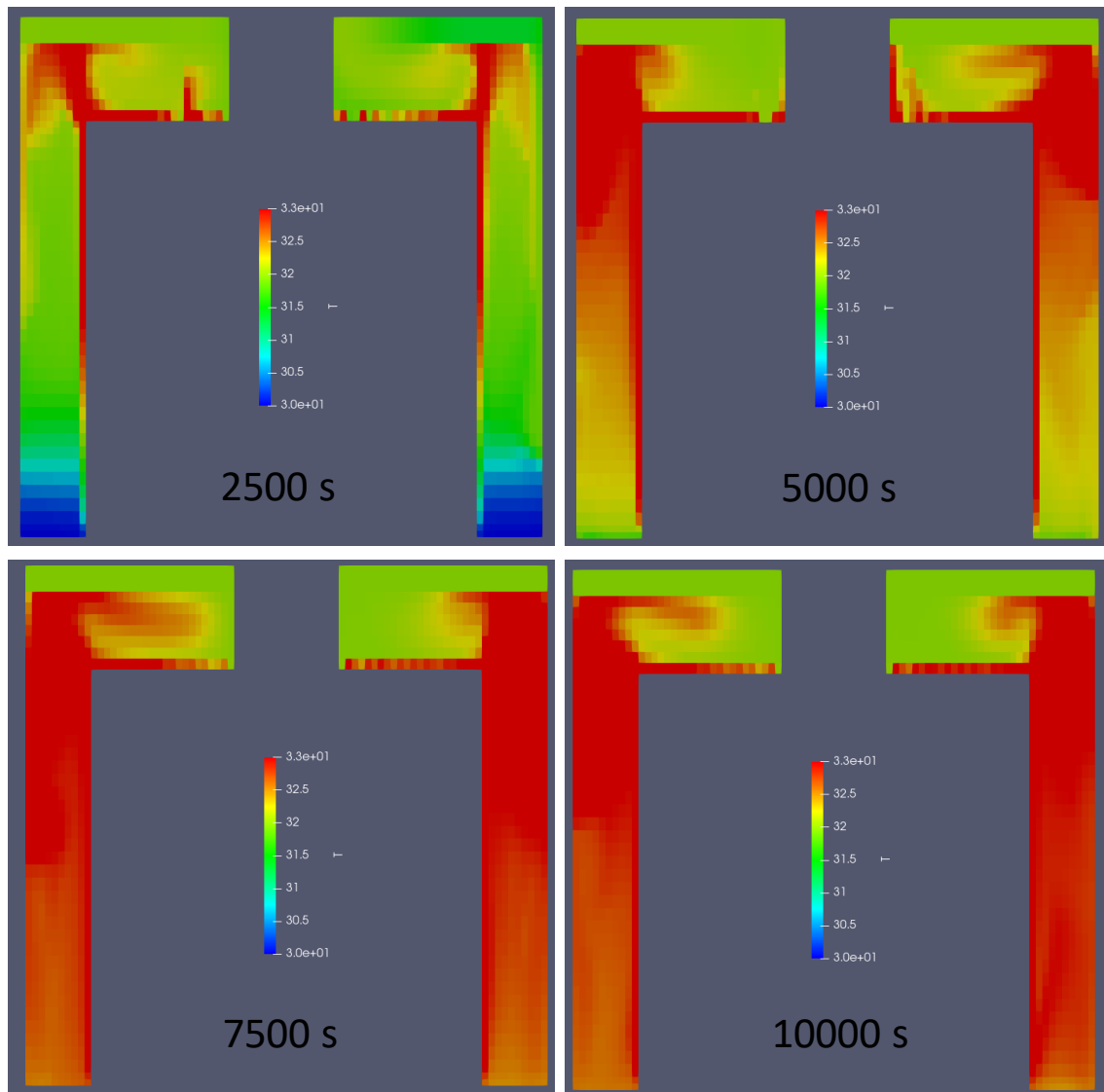
Abb. 3.47 CoPool mit gekoppeltem Datensatz: Temperaturverteilungen in °C
