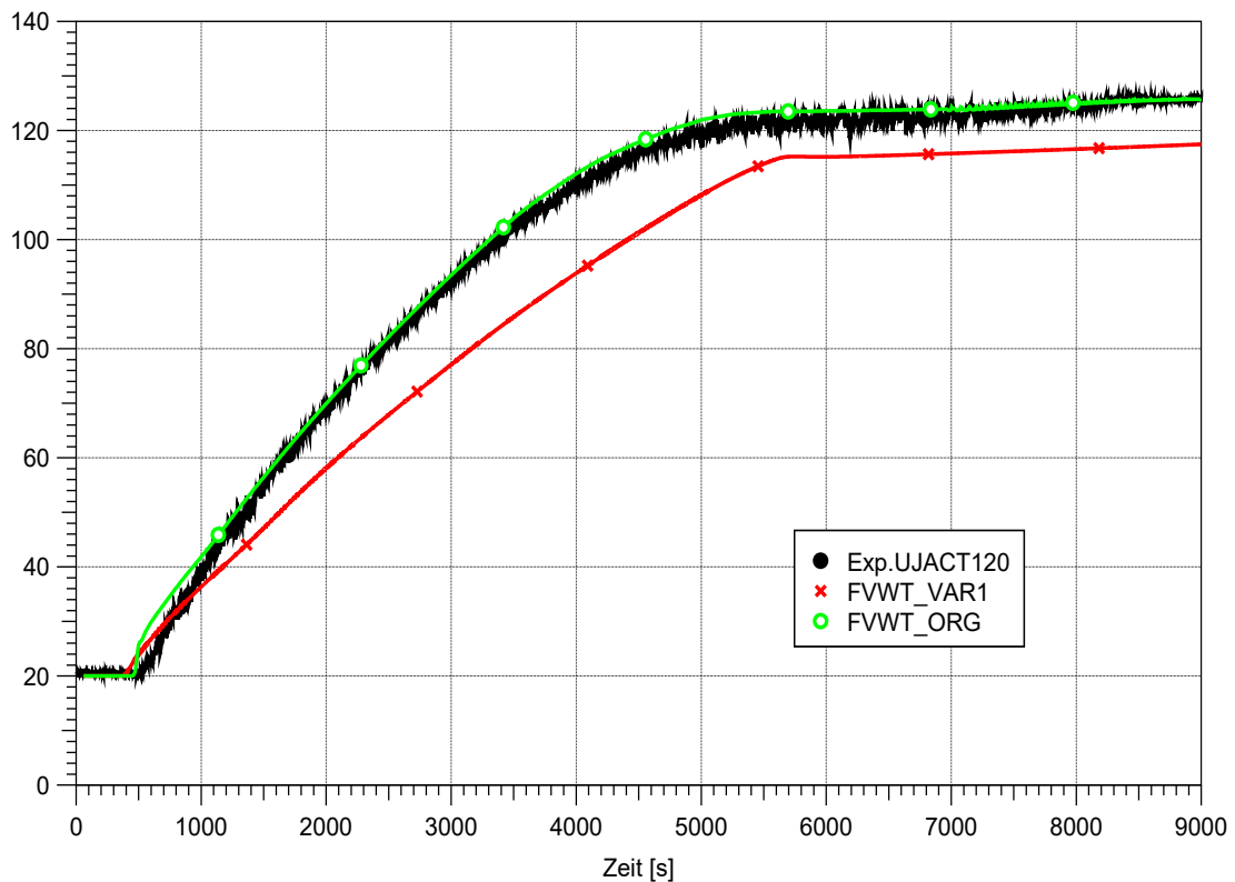
Abb. 3.102 EASY-4, Vergleich der berechneten Wassertemperaturen für die gekoppelte Variantenrechnung (VAR1) und die ursprüngliche Simulation (ORG) mit der im Experiment gemessenen Temperatur im Flutbehälter
