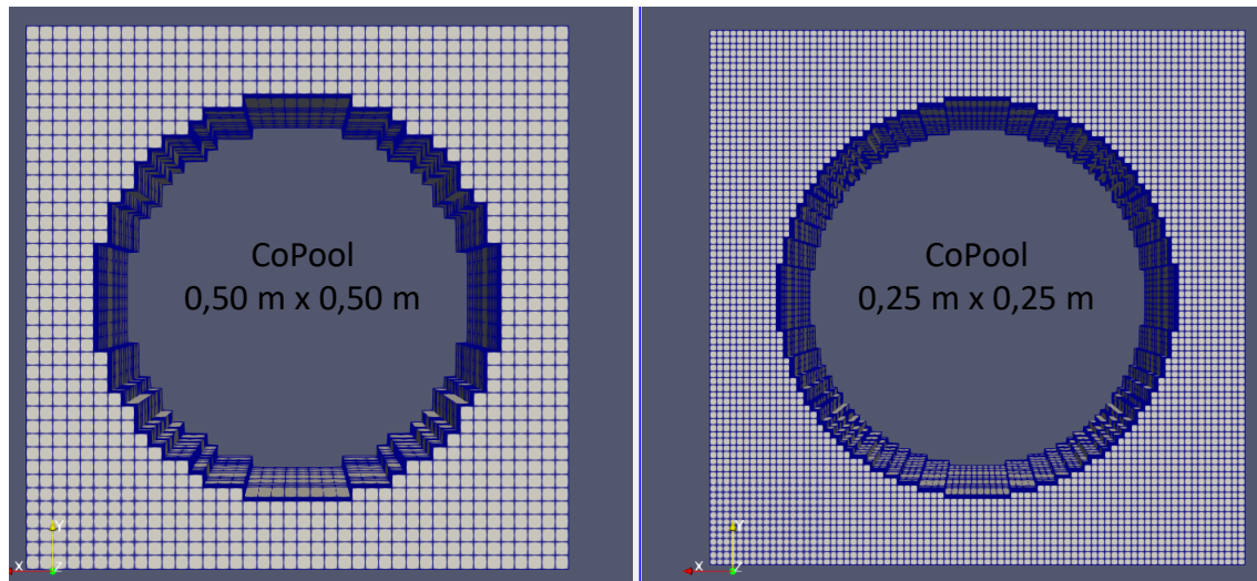
Abb. 3.29 Verfeinerung des CoPool-Gitters im Fluid (Schnitt / Ansicht von oben)
