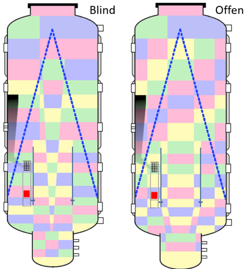
Abb. 2.13 COCOYS Nodalisierungen für den Test THAI HR-57 – blinde Rechnungsphase (links) und offene (rechts)
