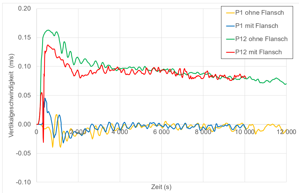
Abb. 3.45 Vertikale Strömungsgeschwindigkeiten bei den Rechnungen ohne und mit Flansch an den Monitorpunkten P1 und P12
