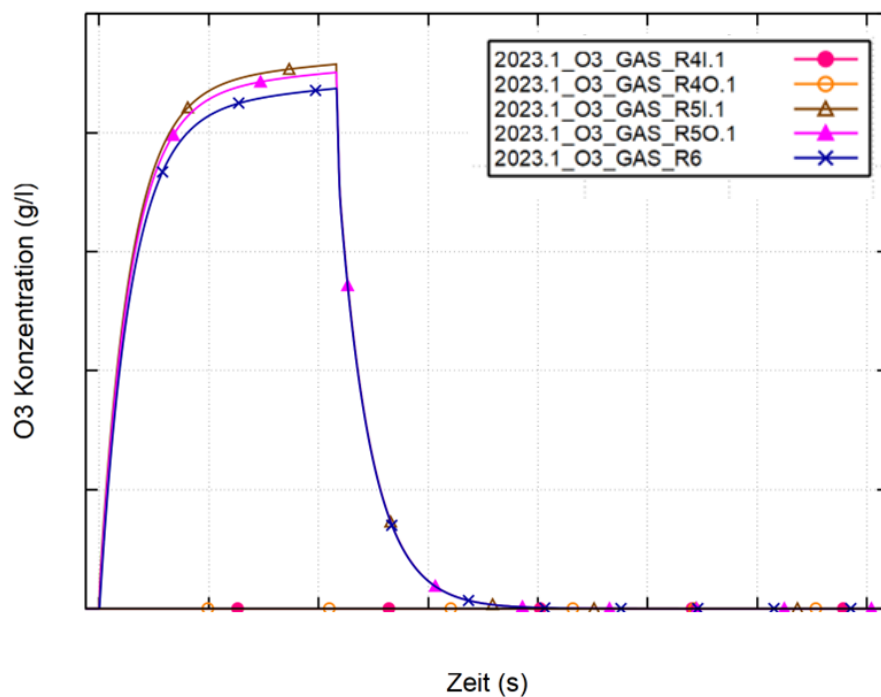
Abb. 2.41 THAI Iod-37, O 3 -Konzentration im THAI-Behälter (anonymisierte Darstellung)
