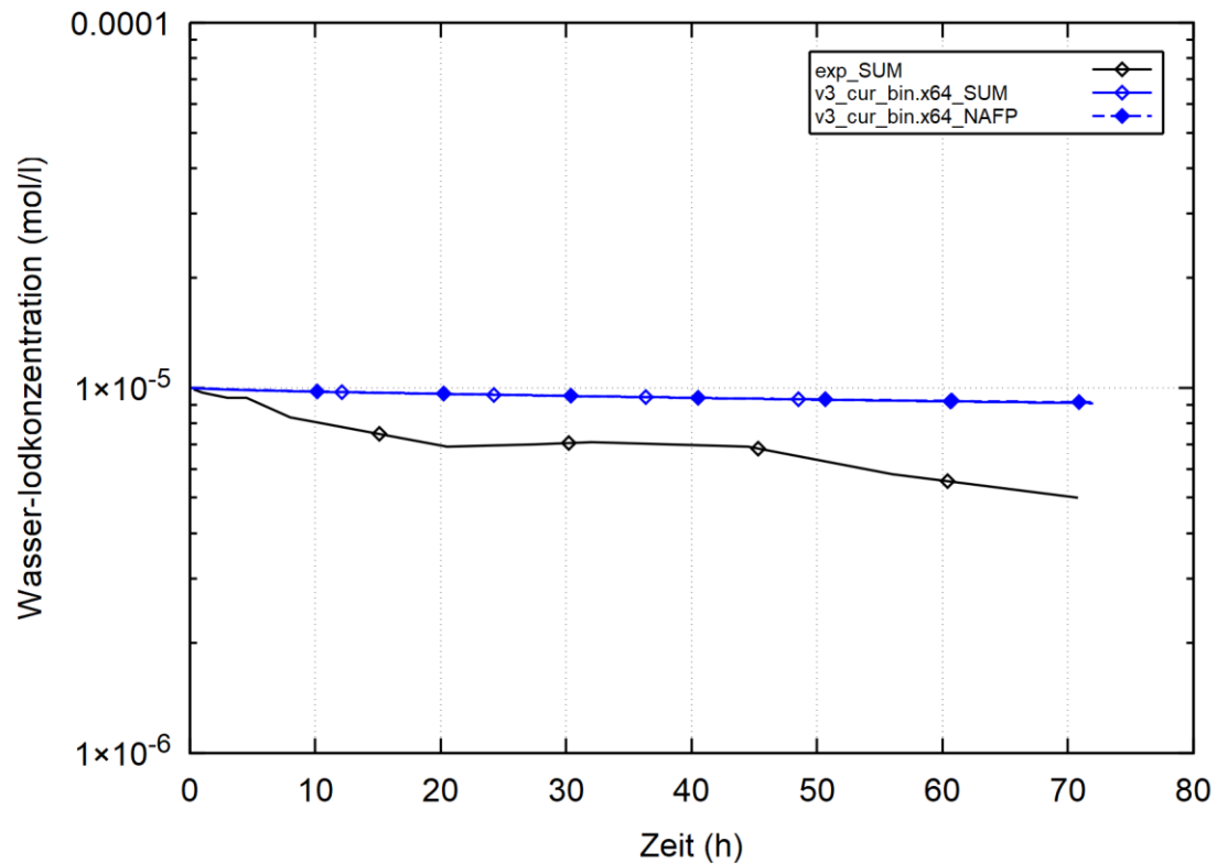
Abb. 2.73 RTF Phebus 1, Iodkonzentration im Wasser gelöst
