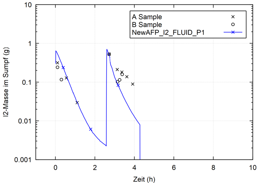
Abb. 2.38 THAI Iod-32, I 2 -Masse im Sumpfwasser
