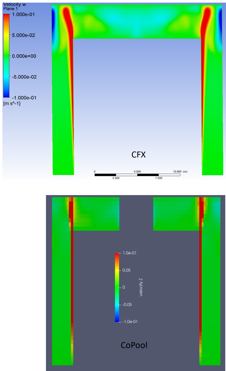
Abb. 3.37 Vertikalgeschwindigkeiten in m/s, CFX (oben) und CoPool (unten), bei t = 500 s
