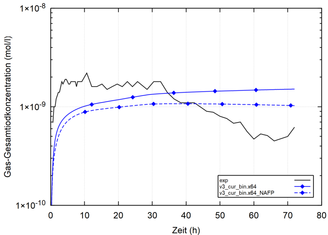
Abb. 2.72 RTF Phebus1, Gesamtiodykonzentration in der Gasphase
