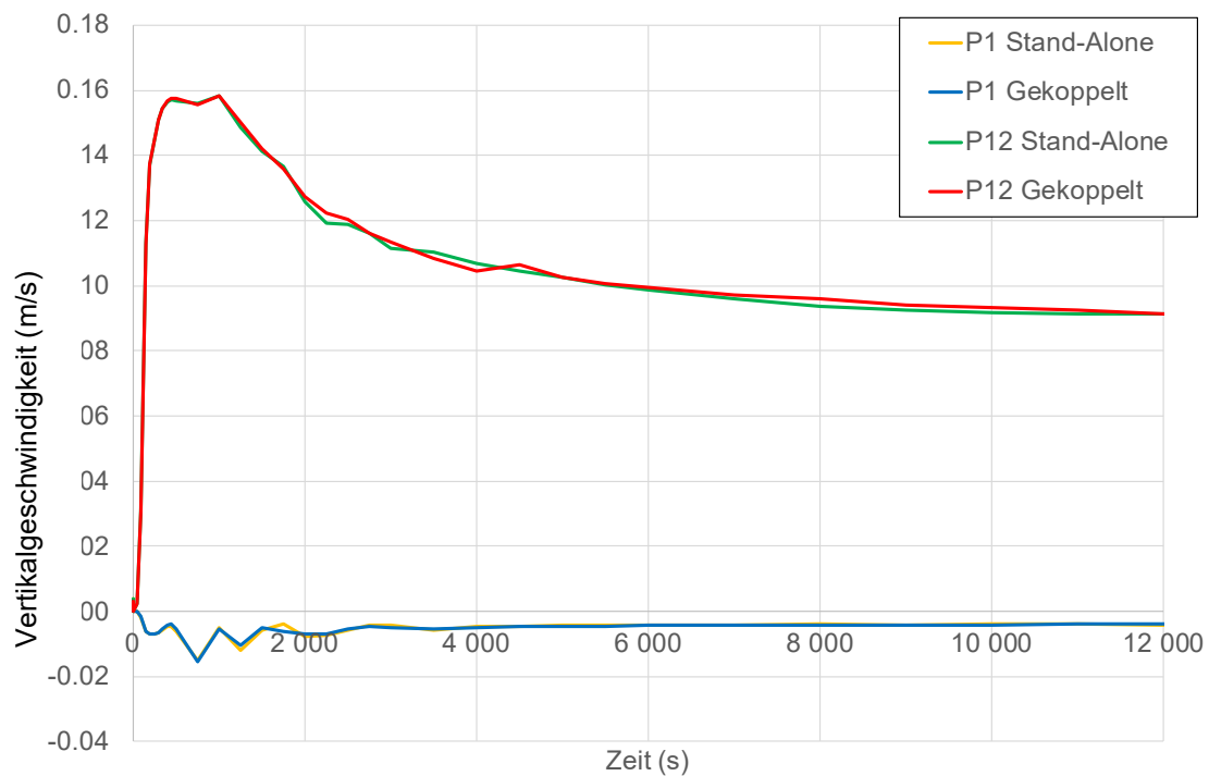
Abb. 3.54 Vergleich der vertikalen Strömungsgeschwindigkeiten an den Monitorpunkten P1 und P12 für die Stand-alone- und die gekoppelte Co-Pool/COCOSYS-Rechnung (neues Gitter)
