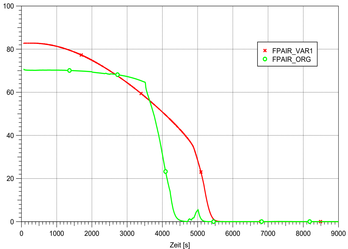
Abb. 3.103 EASY-4, Vergleich der berechneten Luftanteile im Flutbehälter für die gekoppelte Variantenrechnung (VAR1) und die ursprüngliche Simulation (ORG)
