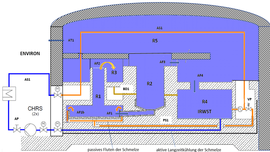
Abb. 2.100 COCOSYS-Nodalisierung des Sicherheitsbehälter einer EPR™-Anlage
