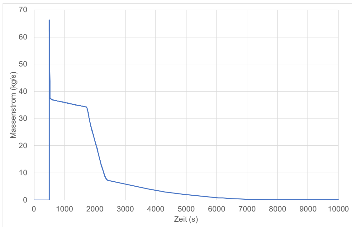
Abb. 3.55 Leckstörfall: Massenstrom für die Einspeisung in COCOSYS-Zone C1
