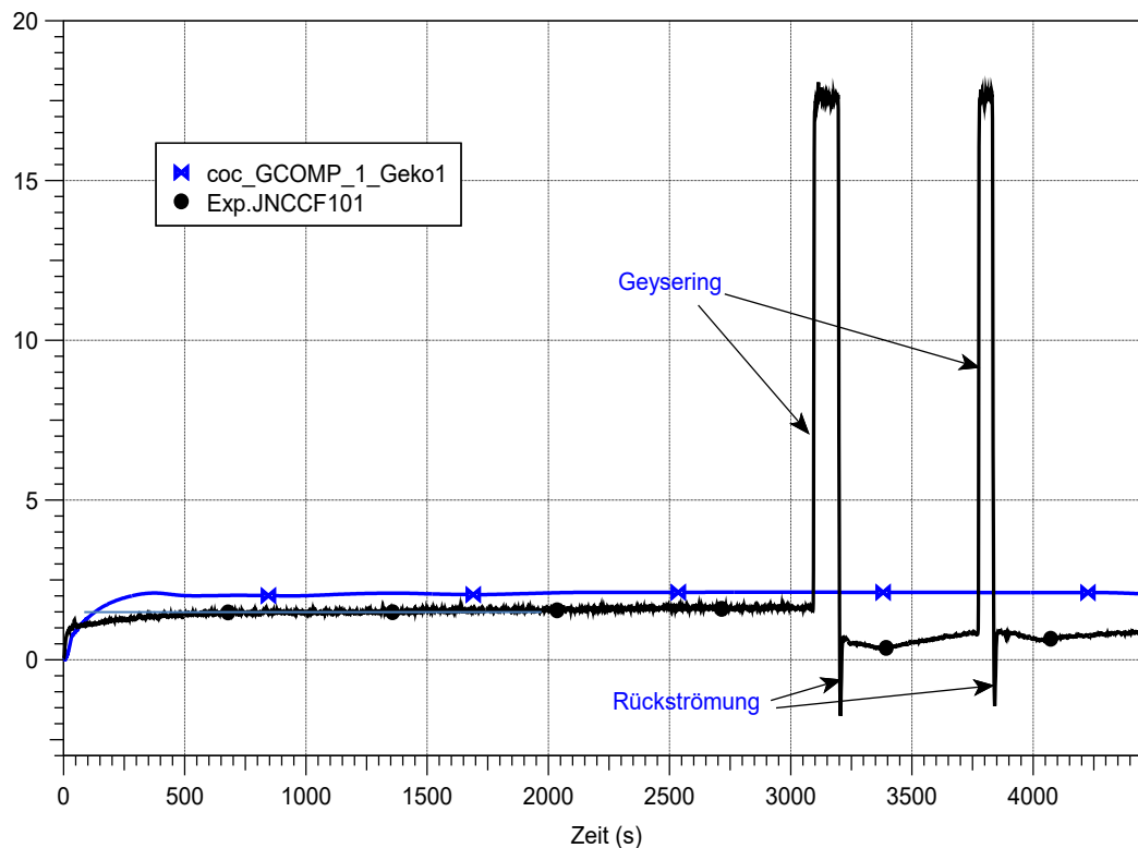
Abb. 3.91 CCC_050_030_20_1, Vergleich des berechneten Massenstroms durch den Gebäudekondensator mit dem im Experiment ermittelten Massenstrom
