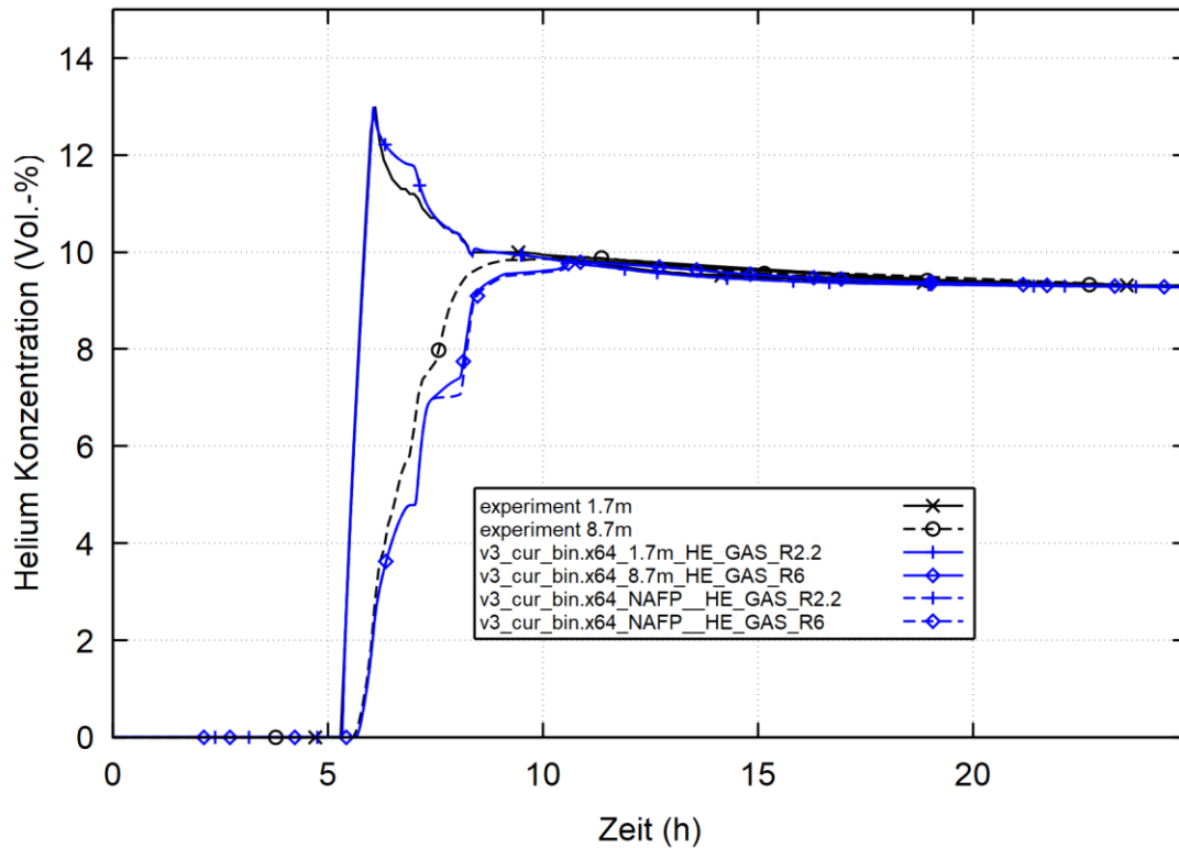
Abb. 2.69 THAI Iod-11, He-Konzentration in einer unteren und einer oberen Zone
