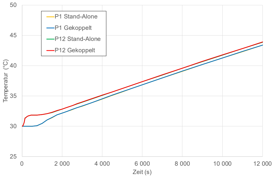
Abb. 3.53 Vergleich der Temperaturen an den Monitorpunkten P1 und P12 für die Stand-alone- und die gekoppelte CoPool/COCOSYS-Rechnung (neues Gitter)
