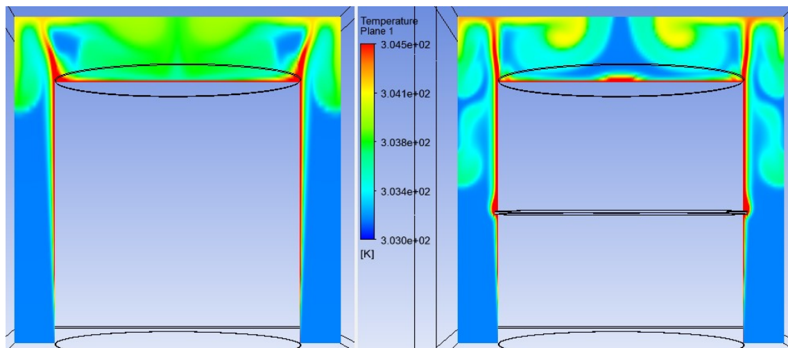
Abb. 3.42 Vergleich der Temperaturen zum Zeitpunkt t = 500 s ohne Flansch (links) und mit Flansch (rechts)
