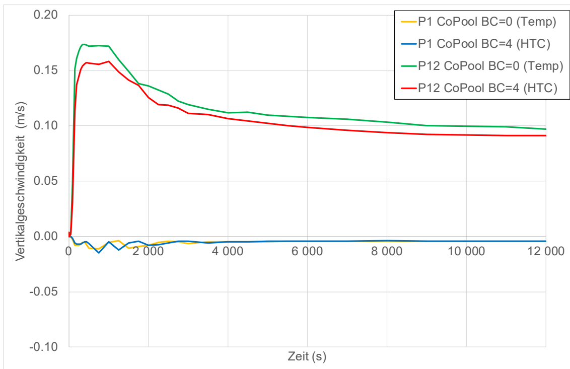
Abb. 3.33 Einfluss der Randbedingung auf die vertikale Strömungsgeschwindigkeit an den Monitorpunkten P1 und P12
