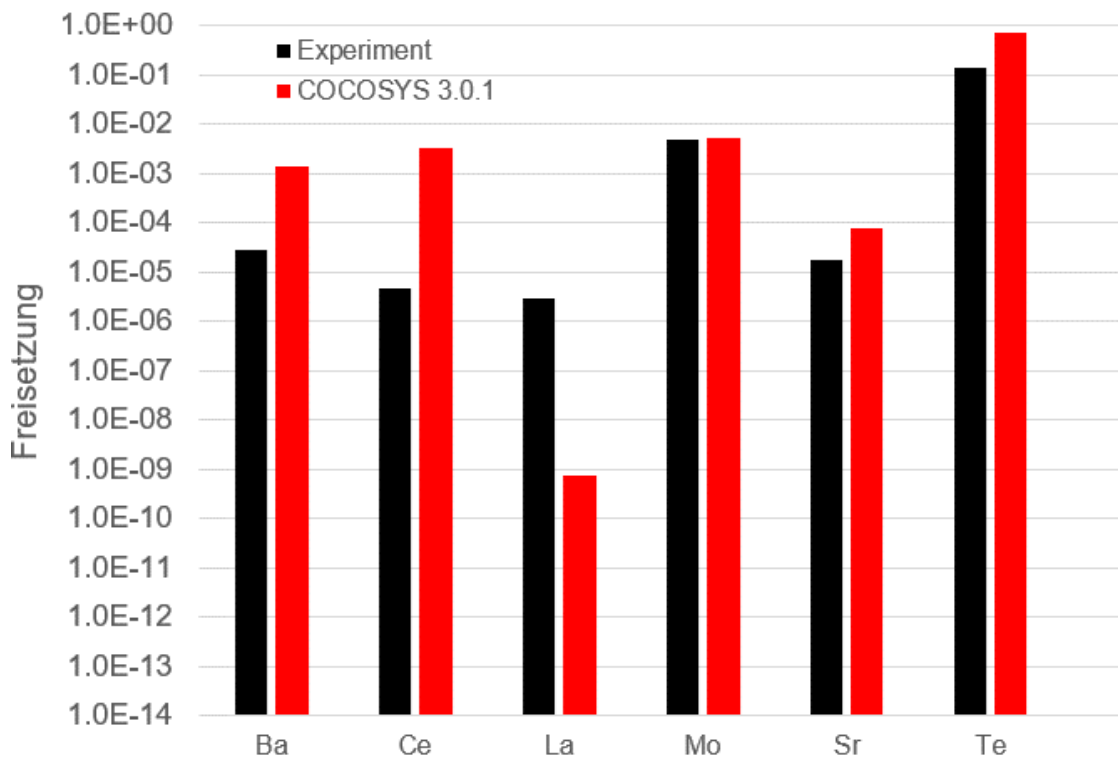
Abb. 2.81 ACE L2, Vergleich der von COCOSYS 3.0.1 berechneten Freisetzung von Spezies (rote Balken) mit der im Experiment ermittelten, anteiligen Freisetzung von Spezies (schwarze Balken)
