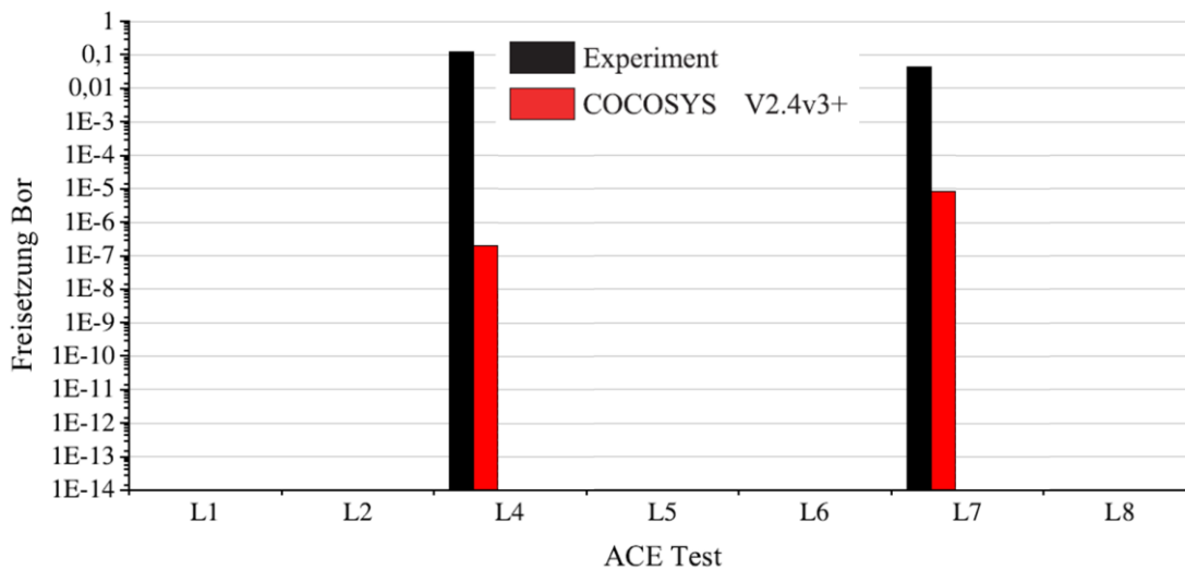
Abb. 2.90 ACE L7, Vergleich der von COCOSYSv2.4v3+ berechneten Freisetzungsrates von Bor (roter Balken) mit der im Experiment ermittelten, anteiligen Borfreisetzung (schwarzer Balken) /AGE 17/
