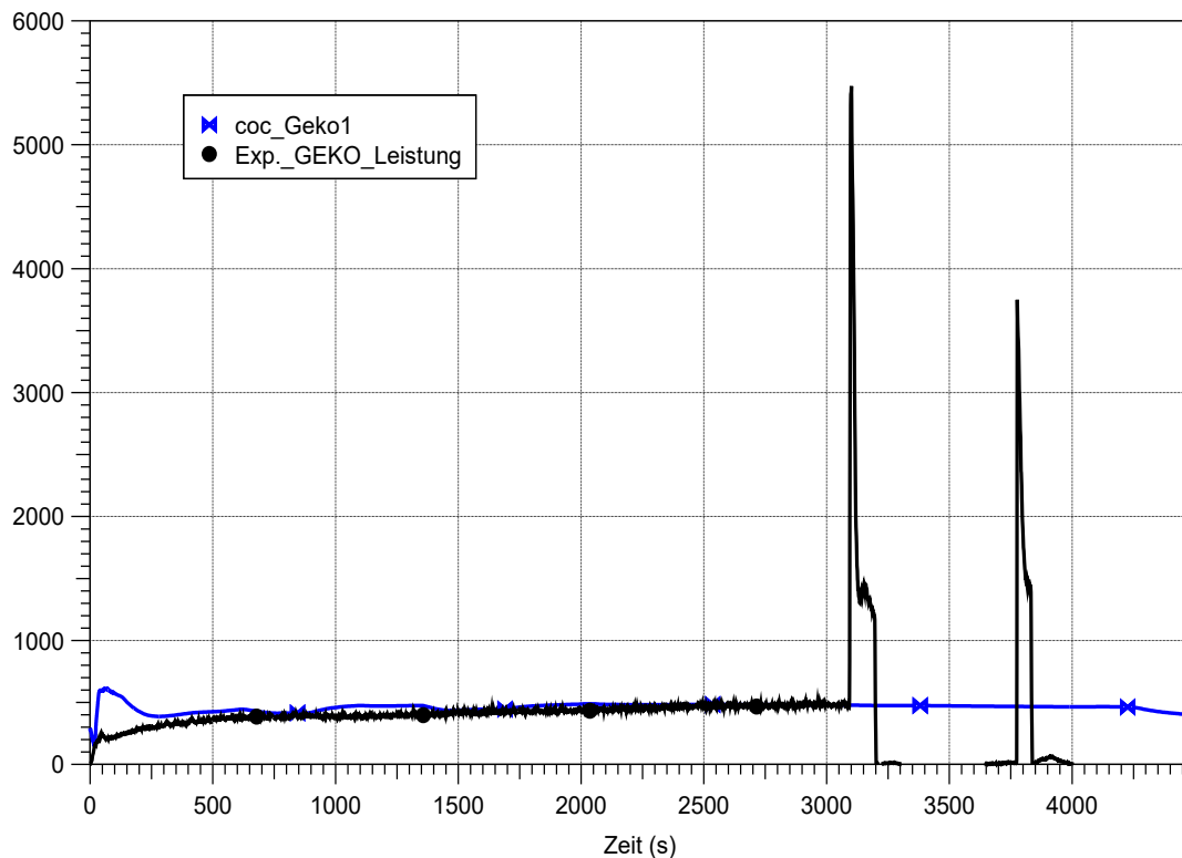
Abb. 3.92 CCC_050_030_20_1, Vergleich der berechneten Kühlleistung mit der im Experiment ermittelten Kühlleistung des Gebäudekondensators
