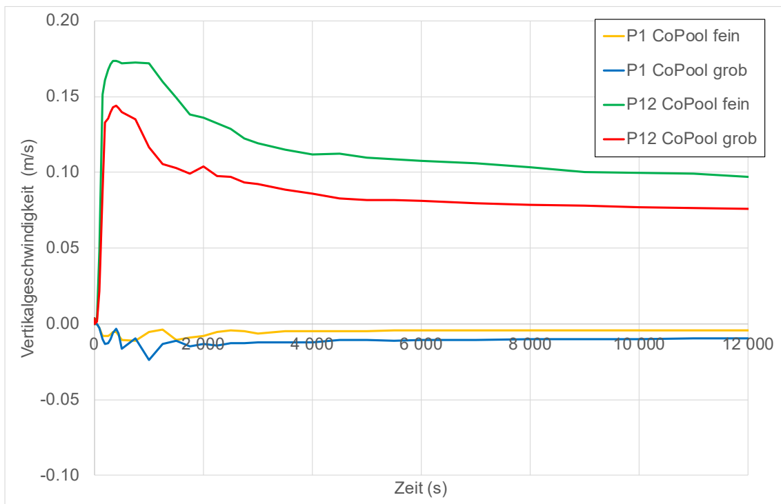
Abb. 3.31 Einfluss der Gitterfeinheit auf die vertikale Strömungsgeschwindigkeit an den Monitorpunkten P1 und P12
