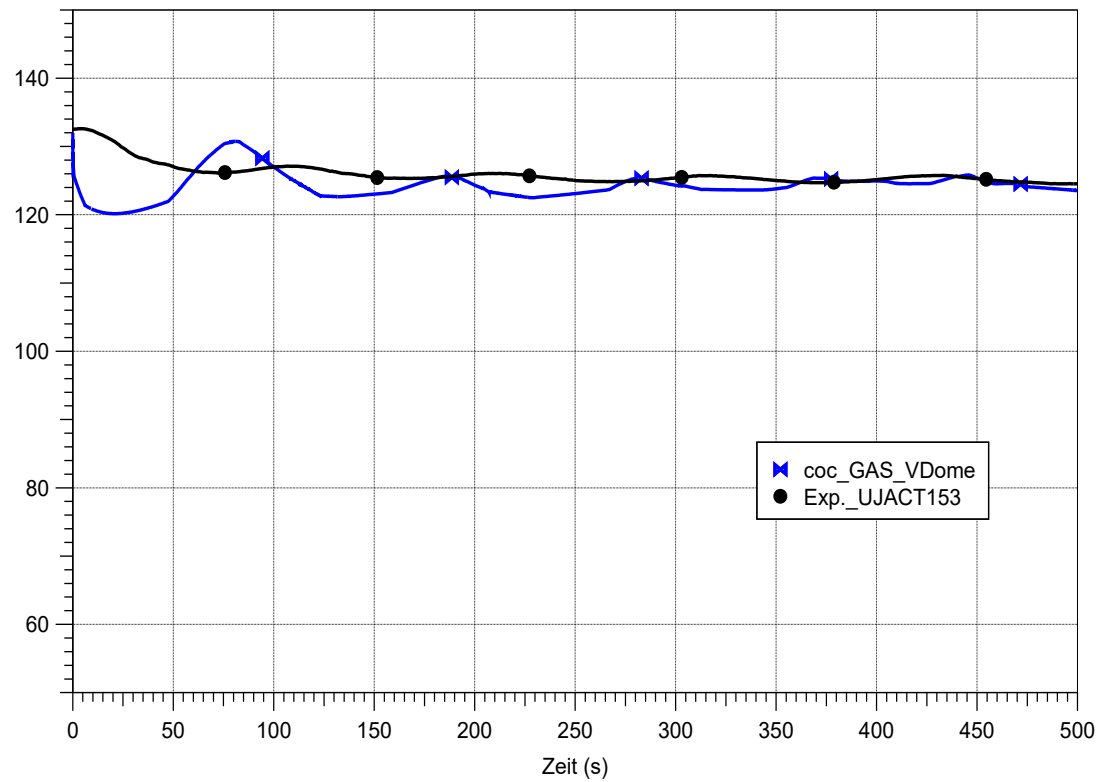
Abb. 3.79 CCC_040_025_100_01, Vergleich der berechneten Atmosphärentemperatur mit der im Experiment gemessenen Temperatur im Flutbehälter
