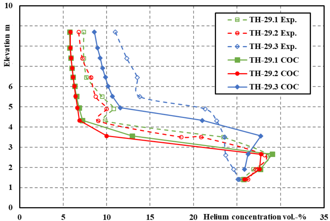
Abb. 2.9 THAI TH-29.1 - 29.3, Vergleich der Heliumkonzentration entlang des Ringraums nach 10,5 h
