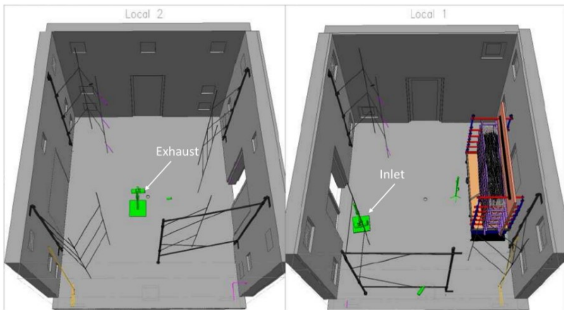
Abb. 2.119 Draufsicht auf die verwendeten Räume in der DIVA-Anlage für die PRS2-CFS-Tests /ZAV 15/
