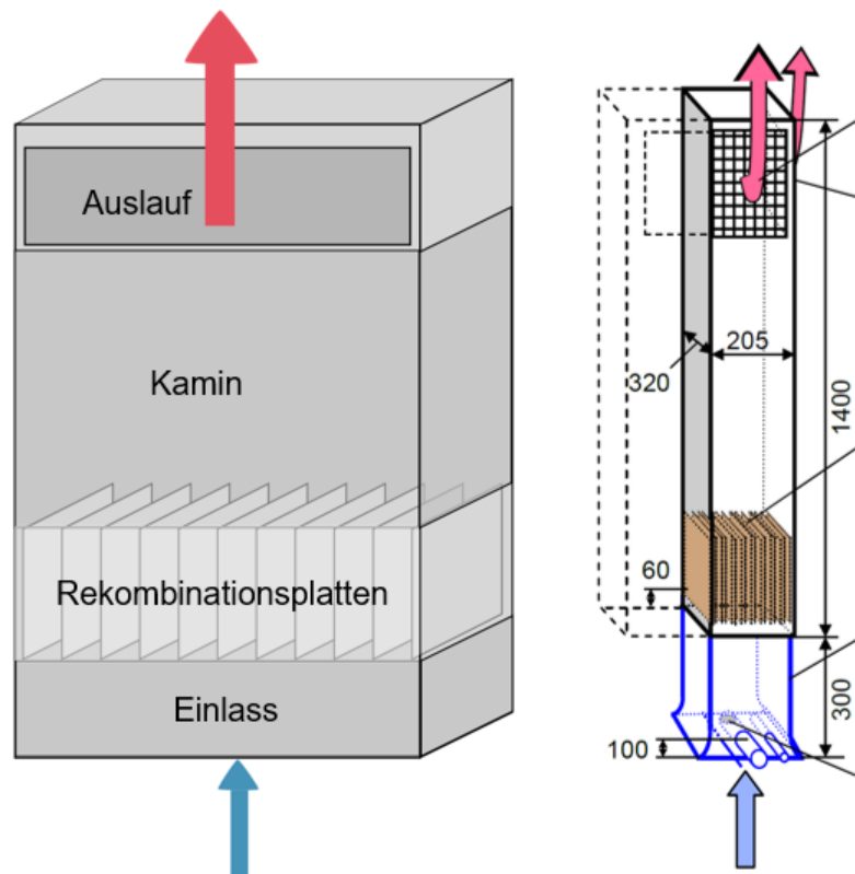
Abb. 2.14 Schema der PAR-Modellierung in COCOSYS (links) und im THAI-Behälter implementierte PAR-Einheit (rechts) /ARN 21a/
