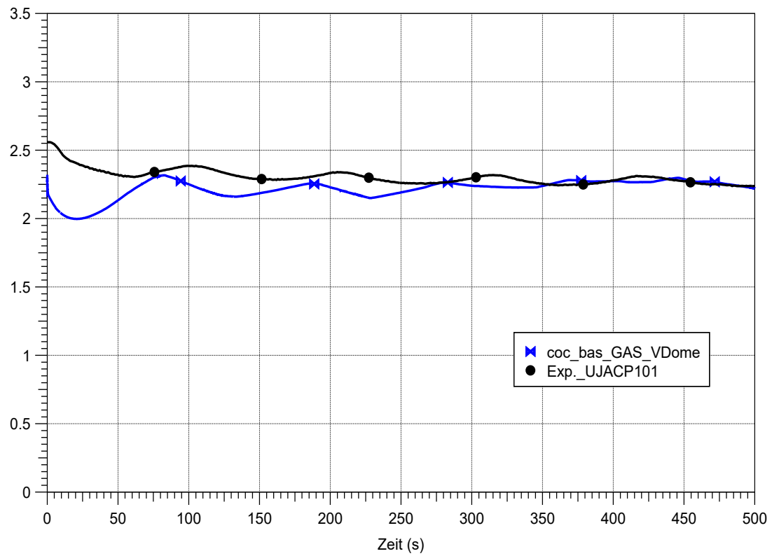
Abb. 3.78 CCC_040_025_100_01, Vergleich des berechneten Druckes mit dem im Experiment gemessenen Druckverlauf im Dom des Flutbehälters.
