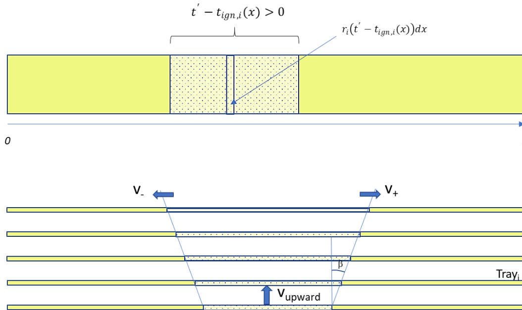
Abb. 2.112 Konzept des erweiterten vereinfachten Kabelbrandmodells in COCOSYS
