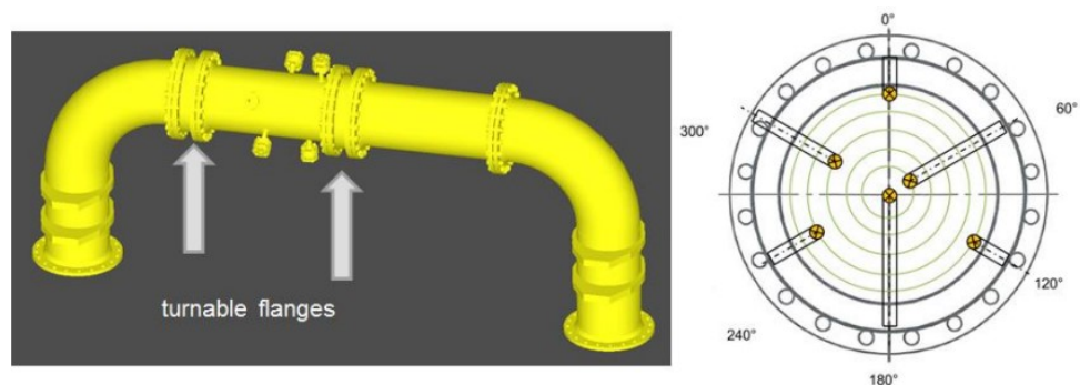
Abb. 2.45 METUSA-Messaufnahme im oberen Verbindungsrohr der THAI-Versuchsanlage /GUP 16/
