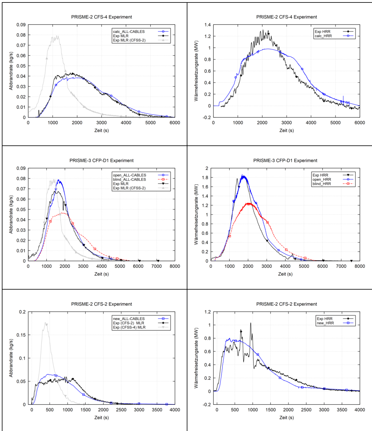
Abb. 2.121 Vergleich der gemessenen und berechneten MLR (links) und HRR (rechts) für die Tests PRS2-CFS-4, PRS3-CFP-D1 und PRS2-CFS-2
