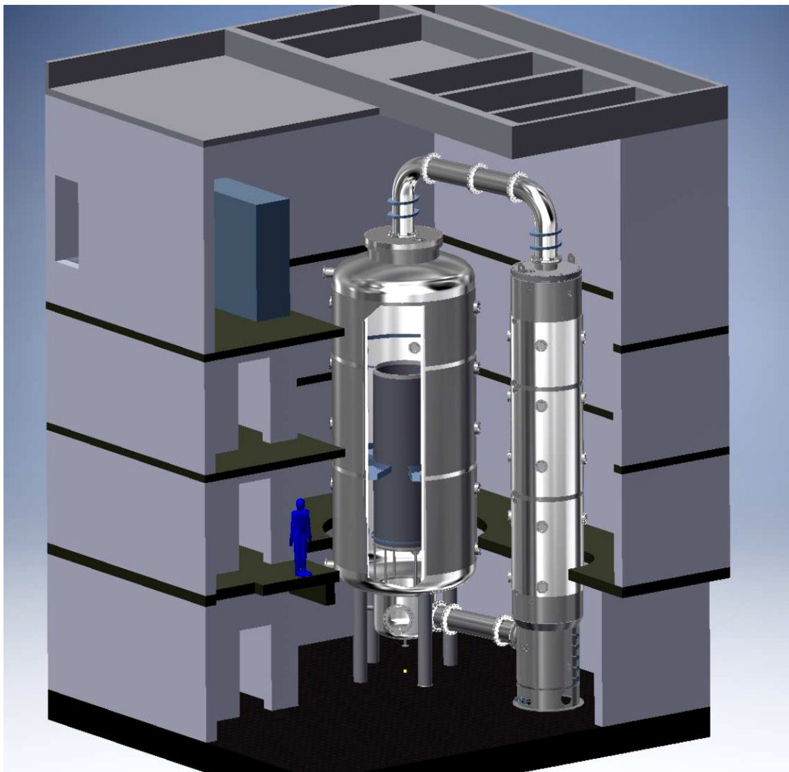
Abb. 1.2 THAI + -Anlage /GUP 19/
