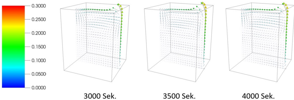
Abb. 3.11 Geschwindigkeitsfeld (in m/s) für y = 10 m bei T = 3000 Sek., T = 3500 Sek. und T = 4000 Sek.
