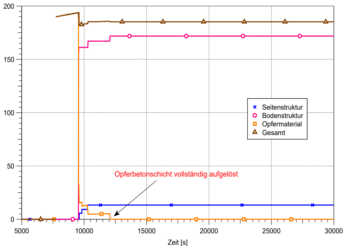
Abb. 2.107 COCOSYS, zeitlicher Verlauf der Kontaktflächen zwischen Schmelze und Boden- und Seitenstrukturen
