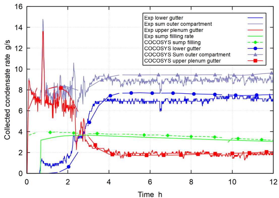
Abb. 2.11 THAI TH-29.3, Vergleich der Kondensatmassenströme
