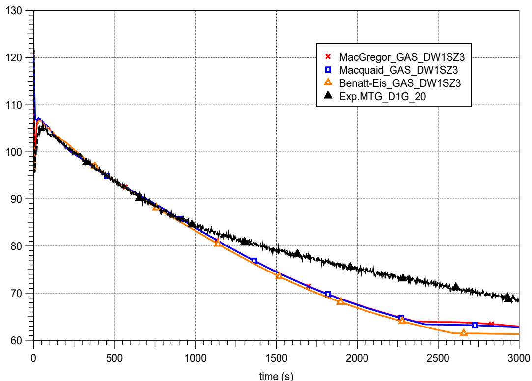
Abb. 2.28 PANDA ST3_2, Vergleich der von den drei COCOSYS-Entrainment-Korrelationen berechneten atmosphärischen Temperatur in Zone mit der im oberen Bereich (Kuppel) von Behälter 1
