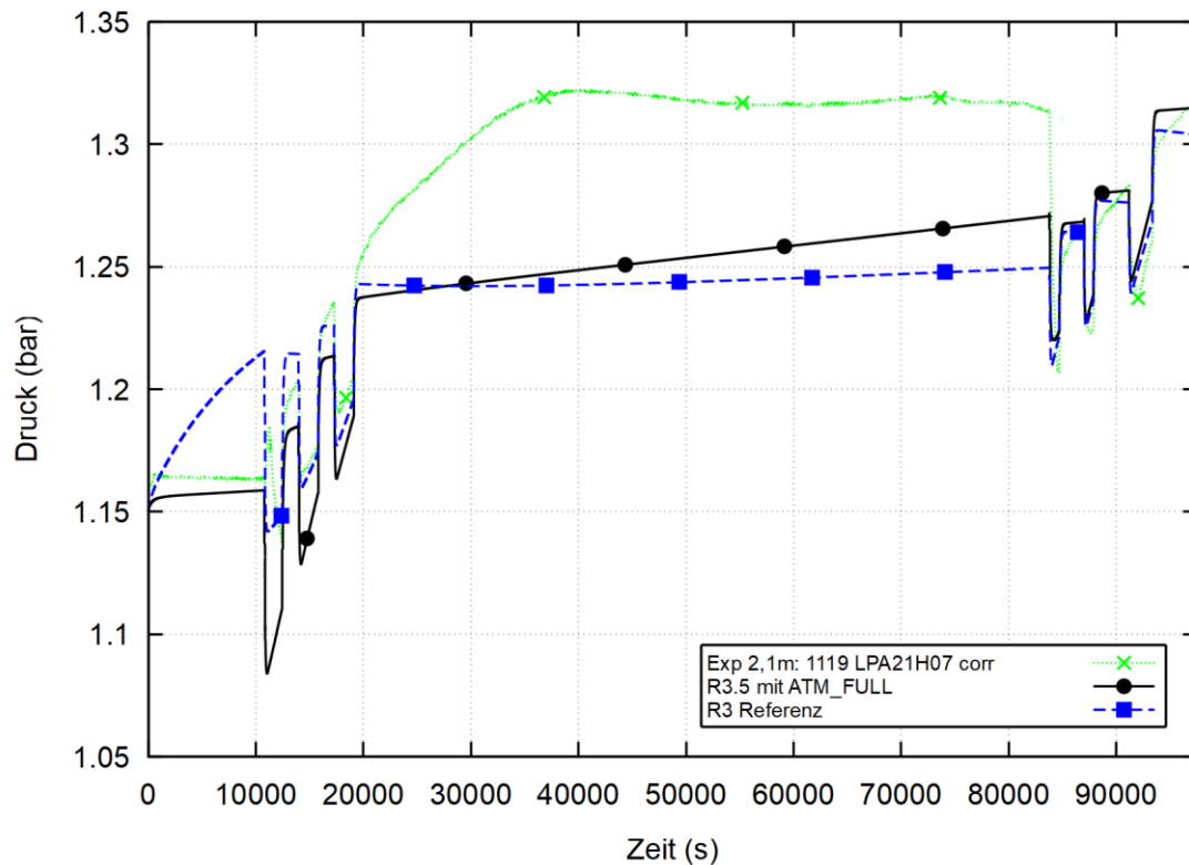
Abb. 2.19 Druckverlauf im PAD
