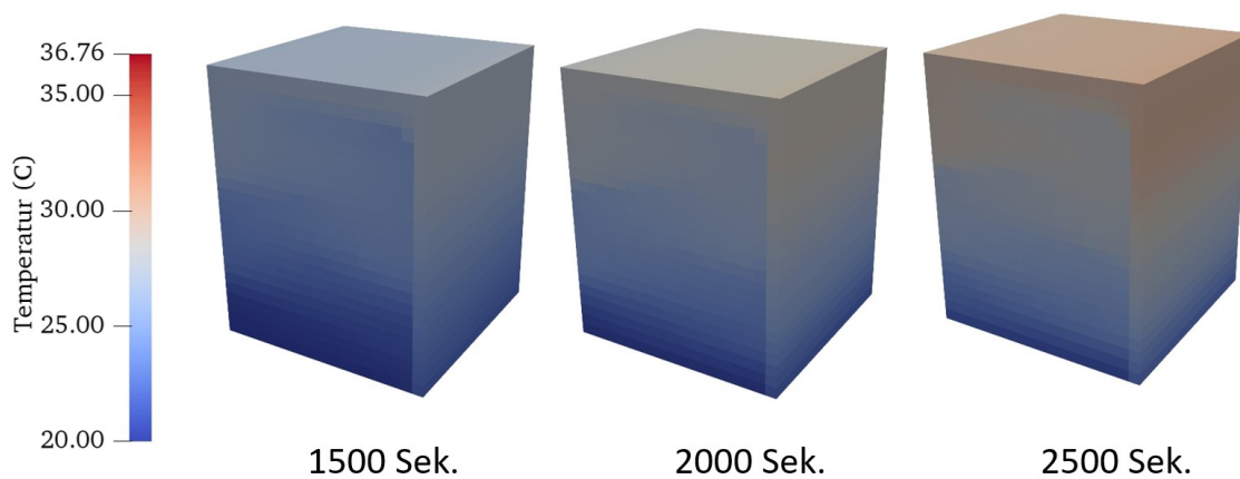
Abb. 3.5 Temperaturverteilung bei T = 1500 Sek., T = 2000 Sek. und T = 2500 Sek
