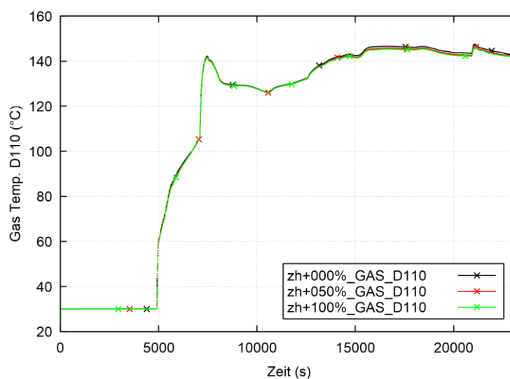
Abb. 4.11 DWR-KONVOI, COCOSYS-Rechnung: Temperaturen im SHB-Dom
