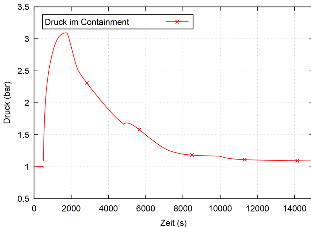
Abb. 3.57 Aktuelle Rechnung: Druckverlauf im Containment (COCOSYS-Zone C1)
