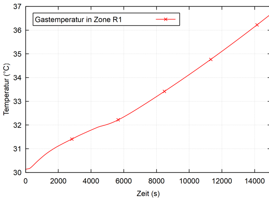
Abb. 3.52 Temperaturverlauf in COCOSYS-Zone R1 (Gasphase / neues Gitter)
