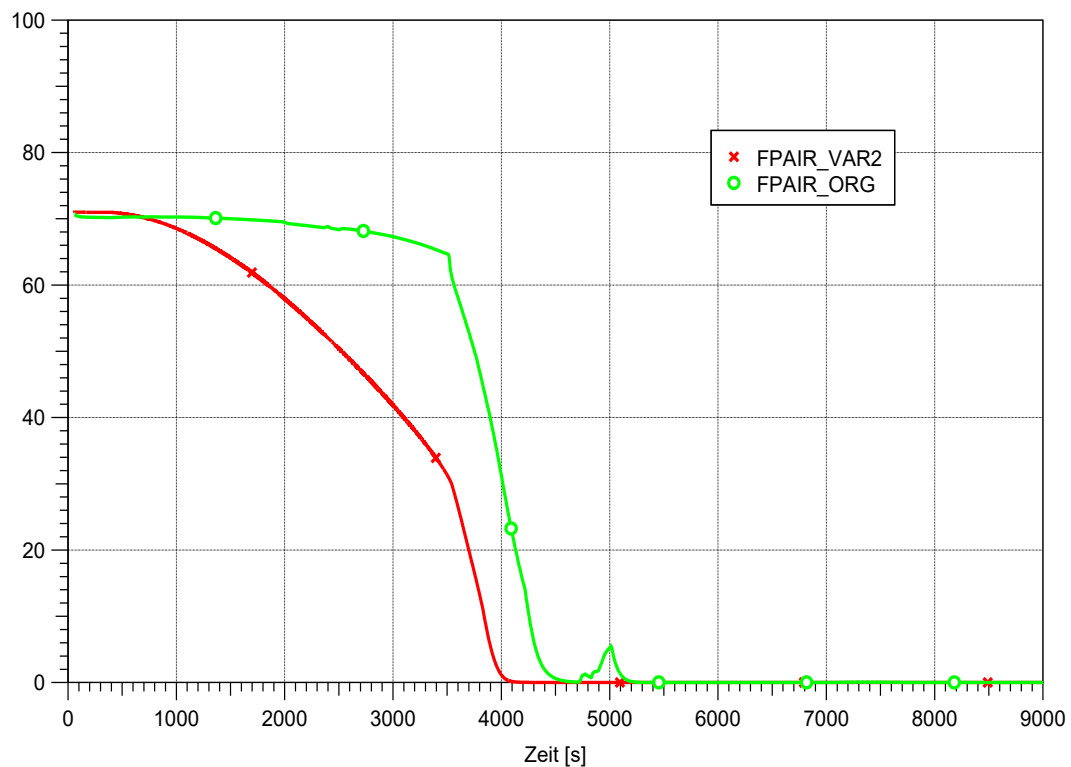
Abb. 3.107 EASY-4, Vergleich der berechneten Luftanteile im Flutbehälter für die vorliegende, gekoppelte Variantenrechnung (VAR1) und die ursprüngliche Simulation (ORG)
