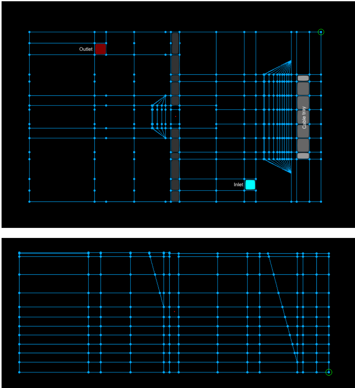
Abb. 2.120 Darstellung der COCOSYS-Nodalisierung (Aufsicht: oben, Seitenansicht: unten)
