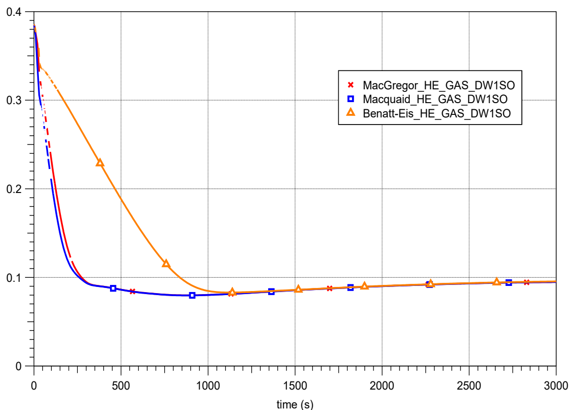
Abb. 2.25 PANDA ST3_2, Vergleich der He-Konzentration in der DW1SO-Zone (Kuppel von Behälter 1), berechnet mit drei verschiedenen COCOSYS-Entrainment-Korrelationen
