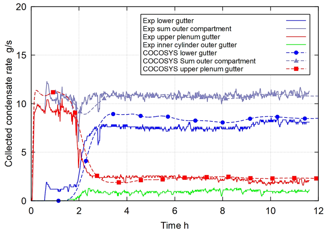
Abb. 2.10 THAI TH-29.1, Vergleich der Kondensatmassenströme
