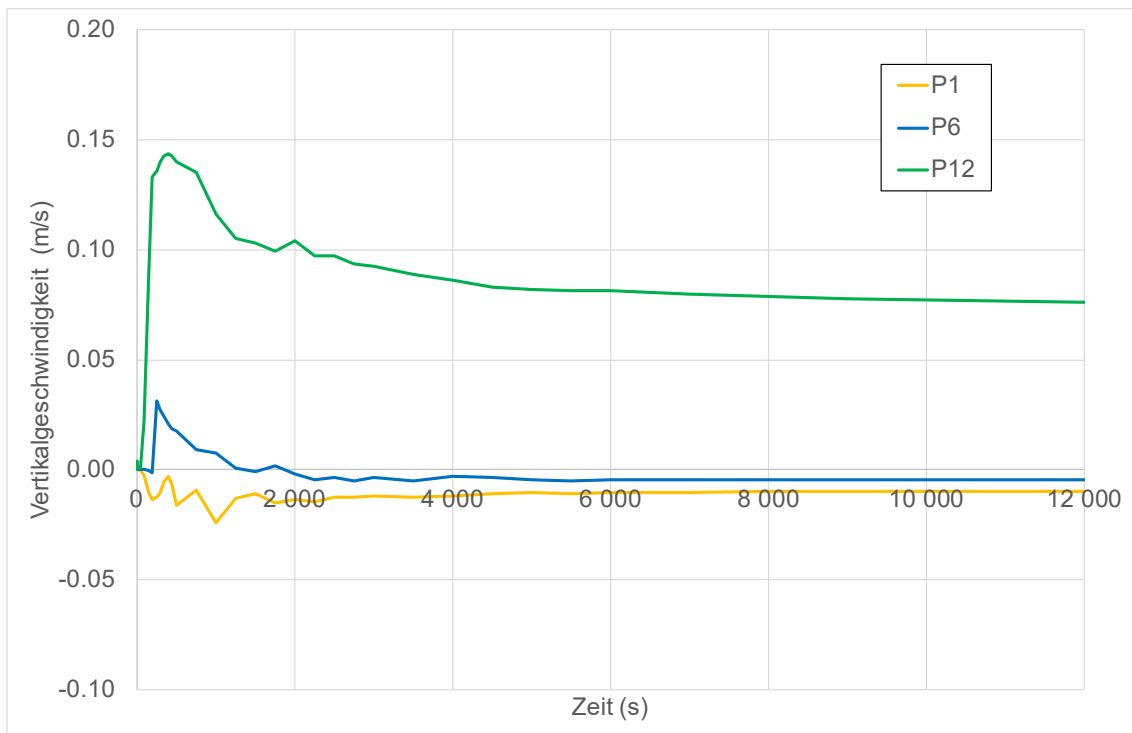
Abb. 3.28 Vertikale Strömungsgeschwindigkeiten an unterschiedlichen Monitorpunkten (P1, P6, P12, vgl. Abb. 3.25)
