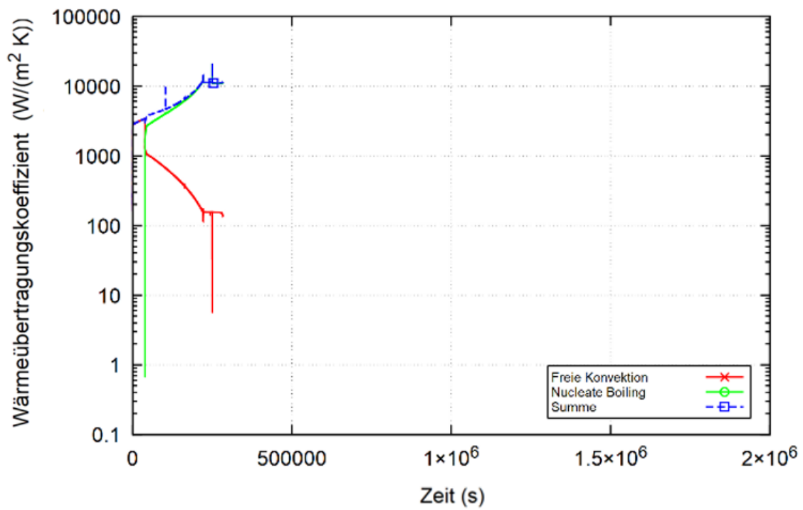
Abb. 3.20 Zeitverlauf der Wärmeübertragungskoeffizienten bei feiner Nodalisierung im Fall stark beheizter Struktur (oberste Struktur)
