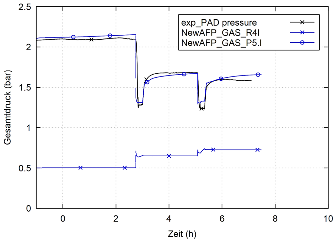
Abb. 2.35 THAI Iod-32, Gesamtdruck
