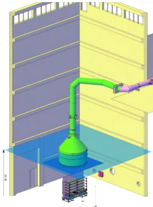
Abb. 2.115 Aufbau der SATURNE-Anlage. Die eingezeichnete Ebene bei 8 m ist die obere Grenze der COCOSYS-Nodalisierung /ZAV 13/
