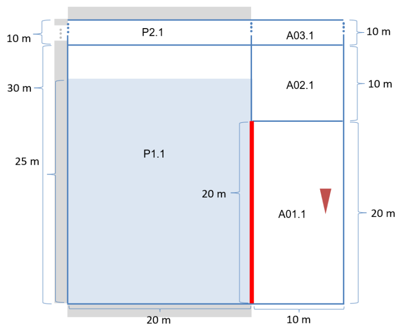
Abb. 3.3 COCOSYS-Schema der Nodalisation – Seitenansicht
