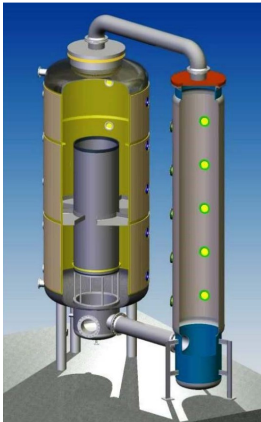
Abb. 2.2 THAI + -Anlage mit THAI Test Vessel (TTV) links und Parallel Attachable Drum (PAD) rechts /REI 19a/
