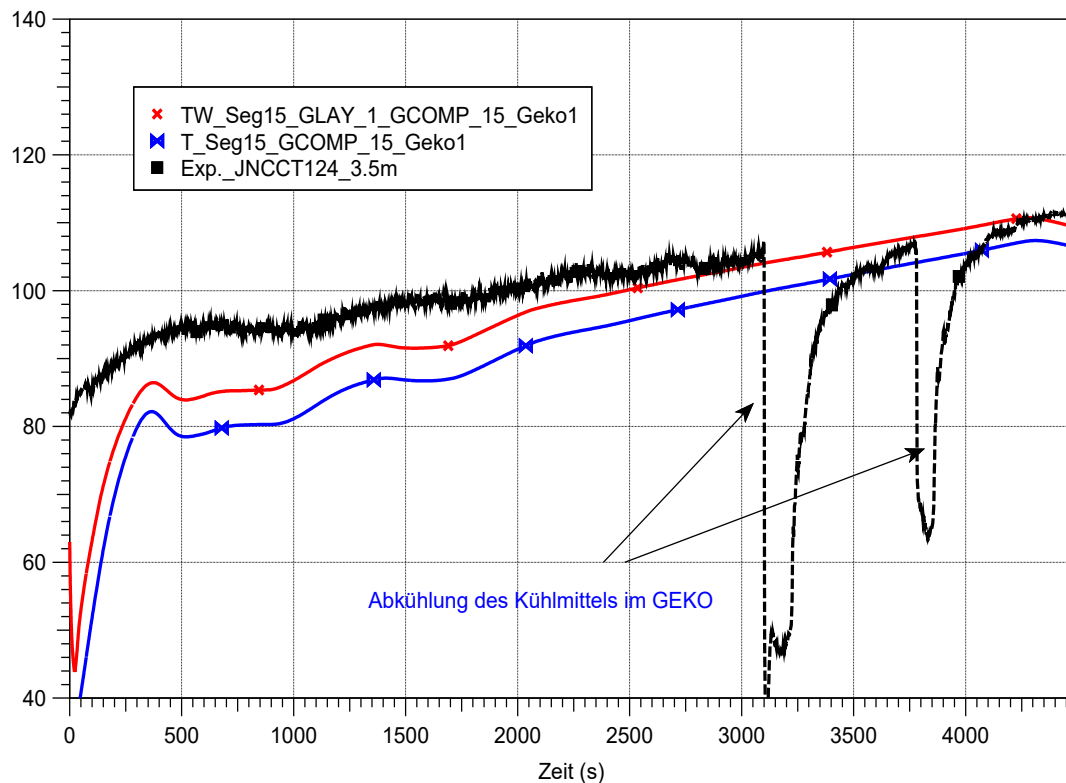
Abb. 3.94 CCC_050_030_20_1, Vergleich der berechneten Kühlmitteltemperatur (Seg_15) mit der im Experiment gemessenen Kühlmitteltemperatur im Wärmetauscherrohr
