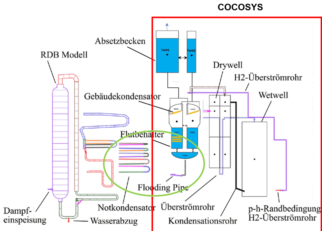
Abb. 3.97 Modifizierte ATHLET/COCOSYS-Nodalisierung der INKA-Versuchsanlage (EASY-4: Station blackout)
