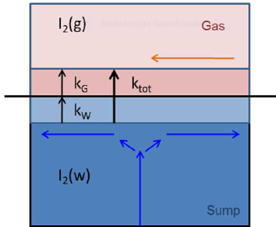
Abb. 2.34 THAI Iod-32, Schemazeichnung des Massentransfers von I_2
