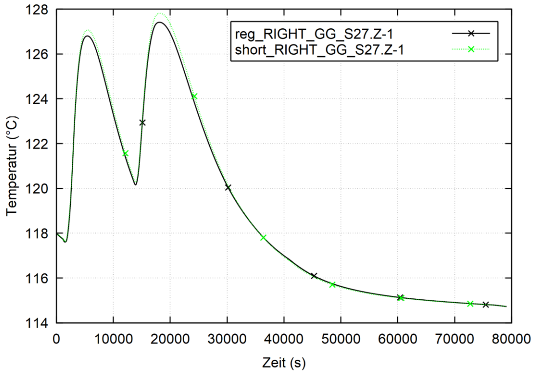
Abb. 4.13 Beispiel für die Temperaturunterschiede in THAI (am Innenzylinder)
