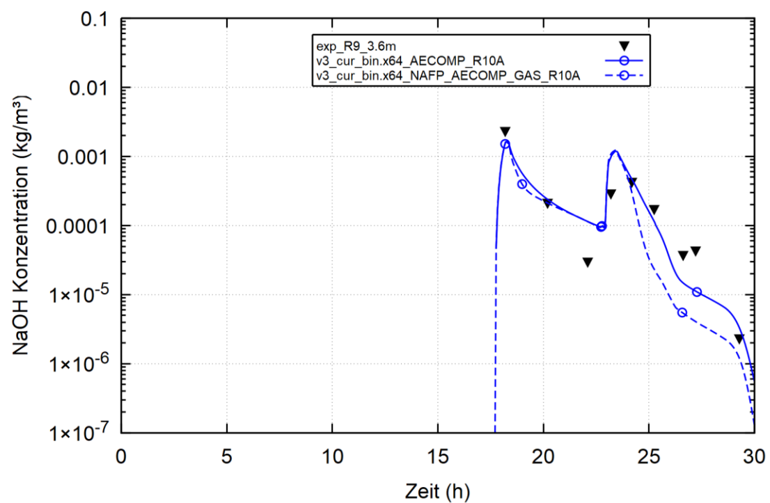
Abb. 2.63 BMC VANAM-M3, Aerosolkonzentration in R10
