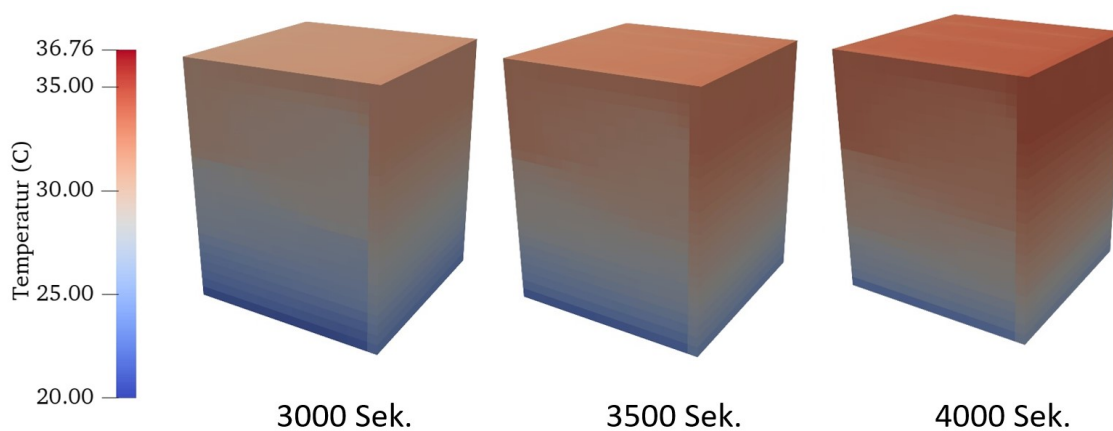
Abb. 3.6 Temperaturverteilung bei T = 3000 Sek., T = 3500 Sek. und T = 4000 Sek.
