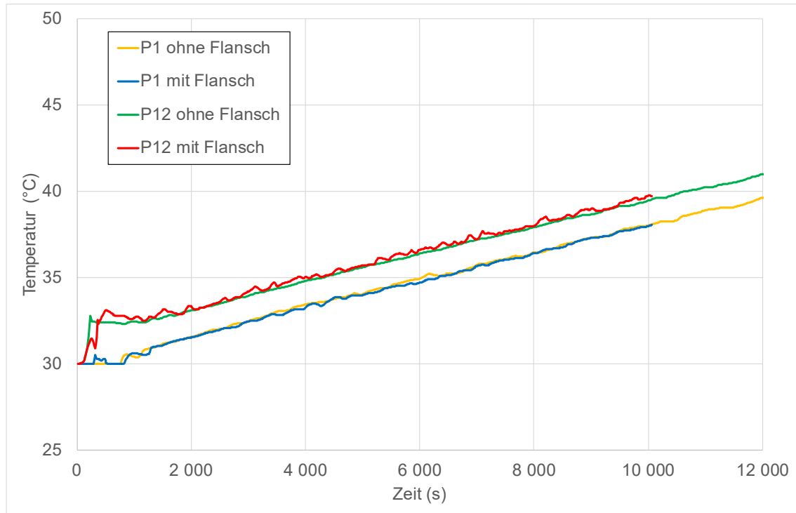
Abb. 3.43 Temperaturen bei den Rechnungen ohne und mit Flansch an den Monitorpunkten P1 und P12
