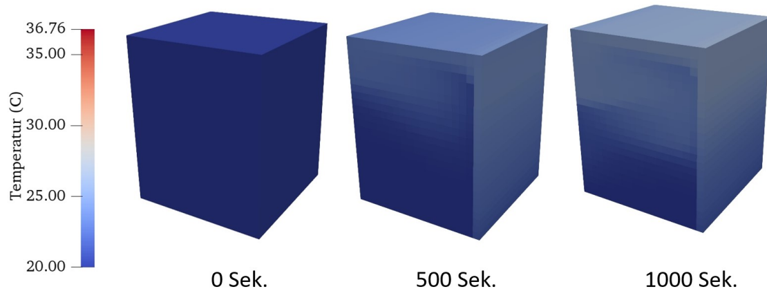
Abb. 3.4 Temperaturverteilung bei T = 0 Sek., T = 500 Sek. und T = 1000 Sek.
