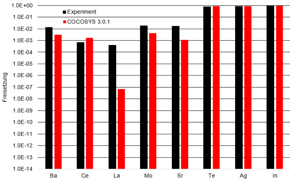
Abb. 2.94 ACE L8, Vergleich der von COCOSYS berechneten Freisetzung von Spezies (rote Balken) mit den im Experiment ermittelten, anteiligen Freisetzungsraten von Spezies (schwarzer Balken)
