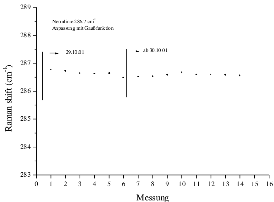
Abb. 3.3 Wellenzahldrift des Spektrometers T640000
