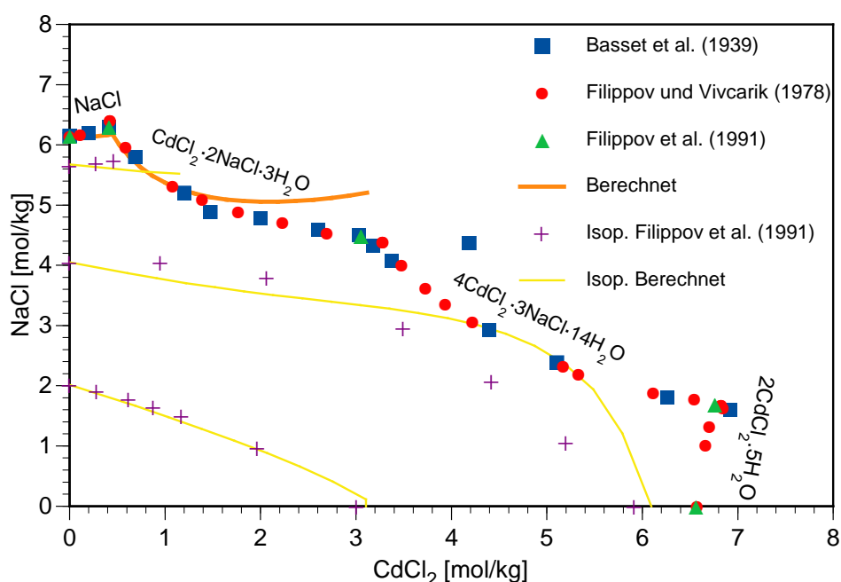
Abb. 7.12 Phasengleichgewichte im System \text{CdCl}_2\text{--NaCl--H}_2\text{O} bei 25^\circ\text{C}
