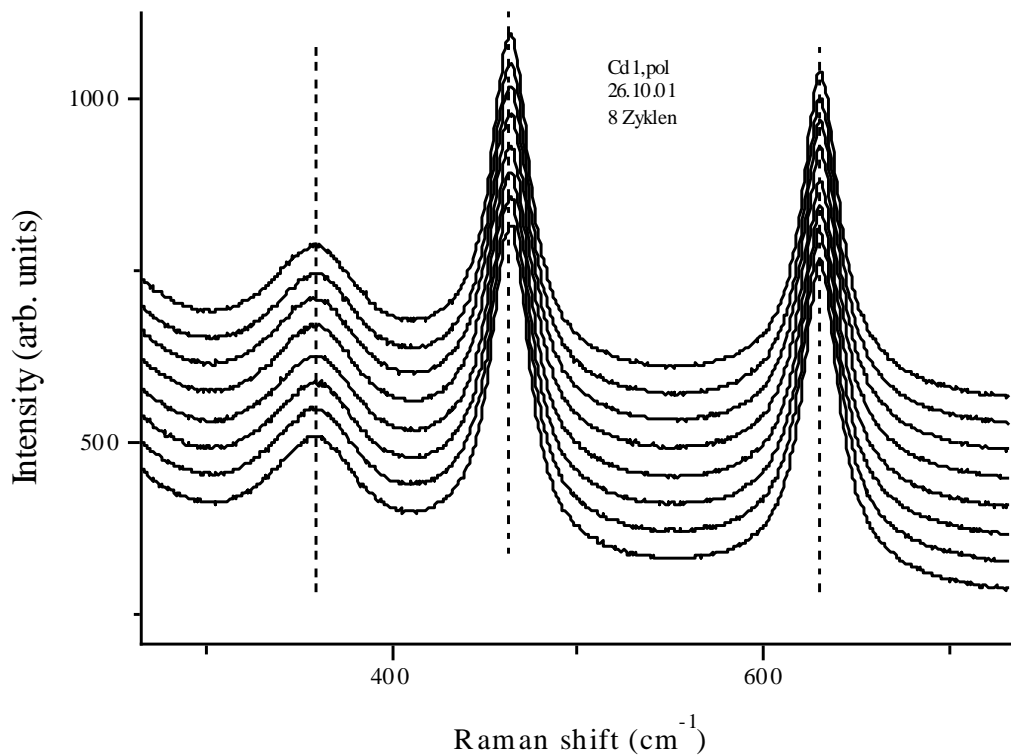
Abb. 3.7 Spektrenakkumulation
