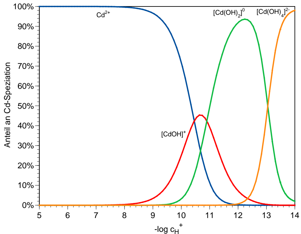
Abb. 9.4 Speziation von Cadmium (II) in 1 mol/kg NaClO 4
