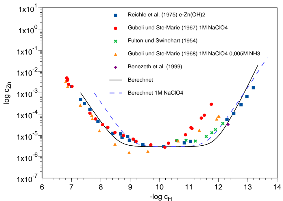
Abb. 10.1 Löslichkeit von Zn(OH) 2 in NaOH-Lösungen
