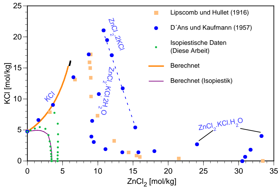
Abb. 8.11 Experimentelle und berechnete Phasengleichgewichte im System \text{ZnCl}_2 – \text{KCl} – \text{H}_2\text{O} bei 25\text{ °C}
