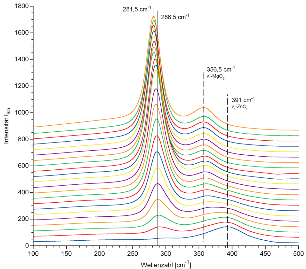
Abb. 3.18 Raman-Spektren von Lösungen des Systems \text{Zn}(\text{ClO}_4)_2\text{-MgCl}_2\text{-H}_2\text{O}
