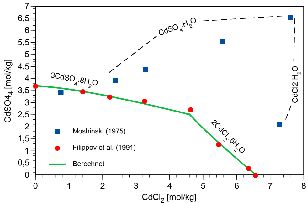
Abb. 7.11 Phasengleichgewichte im System \text{CdCl}_2\text{--CdSO}_4\text{--H}_2\text{O} bei 25 °C
