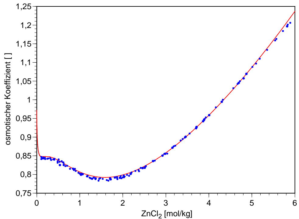
Abb. 8.2 Isopiestic bestimmte (Punkte) und berechnete (Linie) osmotische Koeffizienten im System ZnCl 2 –H 2 O bis 6 mol/kg
