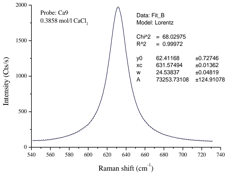
Abb. 3.12 Anpassung der Bande bei 632\text{ cm}^{-1} durch eine Lorentzbande
