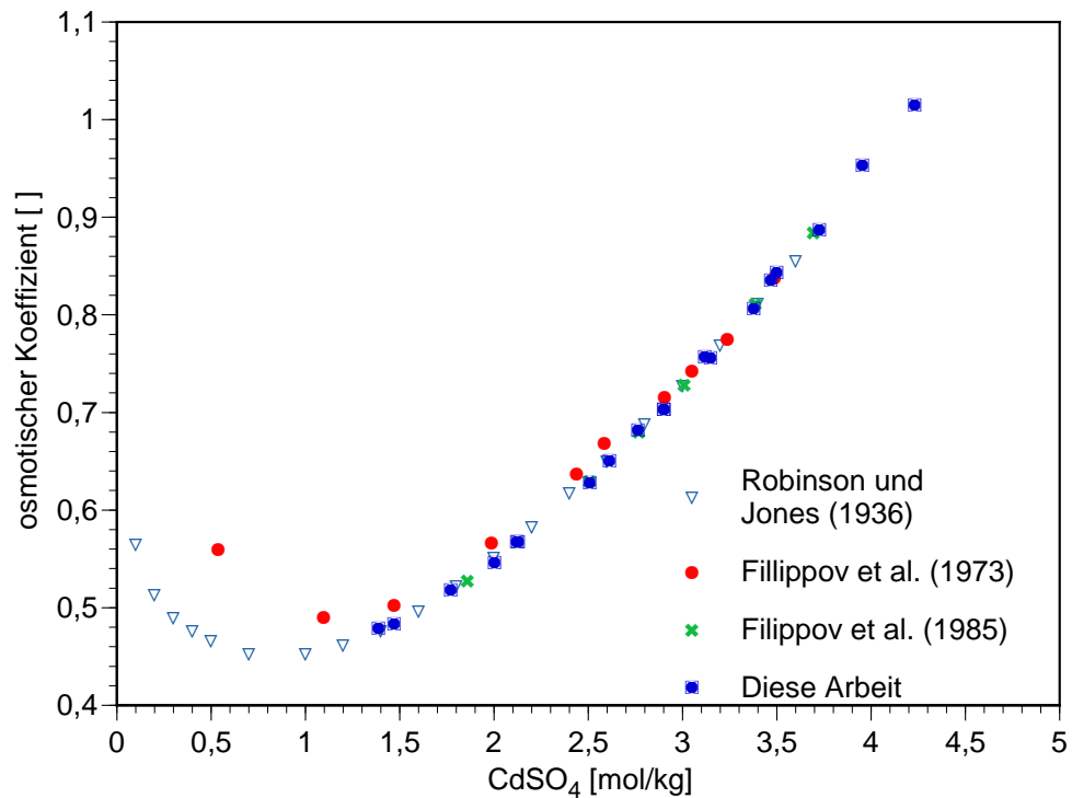
Abb. 2.16 Experimentell bestimmte osmotische Koeffizienten von CdSO 4 -Lösungen bei 25,0 °C (Literaturdaten sowie diese Arbeit)
