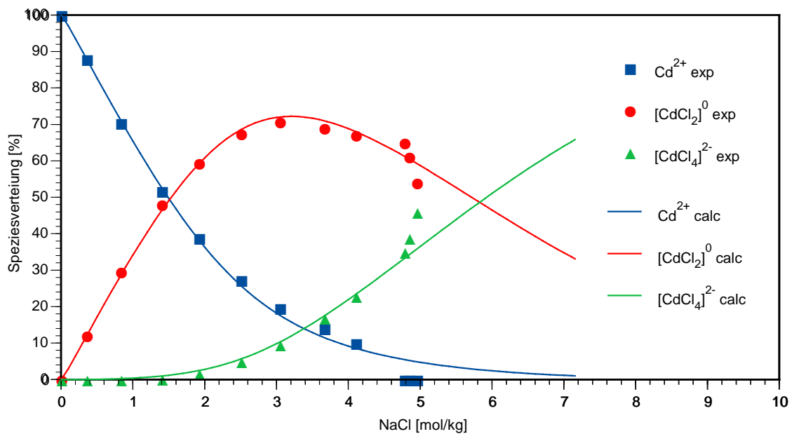
Abb. 7.1 Experimentell bestimmte (Raman) und berechnete Chlorokomplexbildung im System \text{Cd}(\text{ClO}_4)_2 - \text{NaCl} - \text{H}_2\text{O} bei 25 °C ( c[\text{Cd}(\text{ClO}_4)_2] = 1,2 \text{ mol/kg} )
