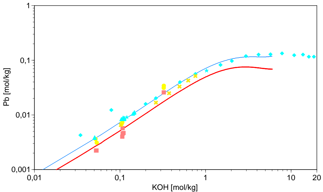
Symbole: Lithargit (rot), Massicot (gelboliv), Bleioxidhydrat (hellblau), Natriumplumbit (dunkelblau) Linien: berechnete Werte für Lithargit (rot) und Bleioxidhydrat (blau)
