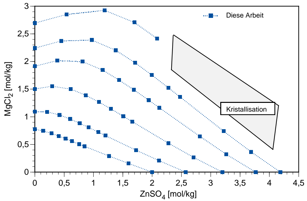
Abb. 2.13 Isoaktivitätslinien im quasi-ternären System ZnSO 4 – MgCl 2 – H 2 O
