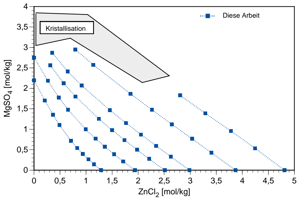
Abb. 2.14 Isoaktivitätslinien im quasi-ternären System ZnCl 2 – MgSO 4 – H 2 O
