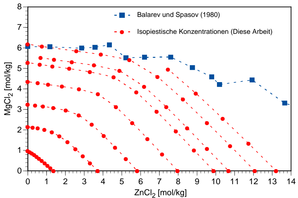
Abb. 2.7 Isopiestic Konzentrationen im System \text{ZnCl}_2 - \text{MgCl}_2 - \text{H}_2\text{O}
