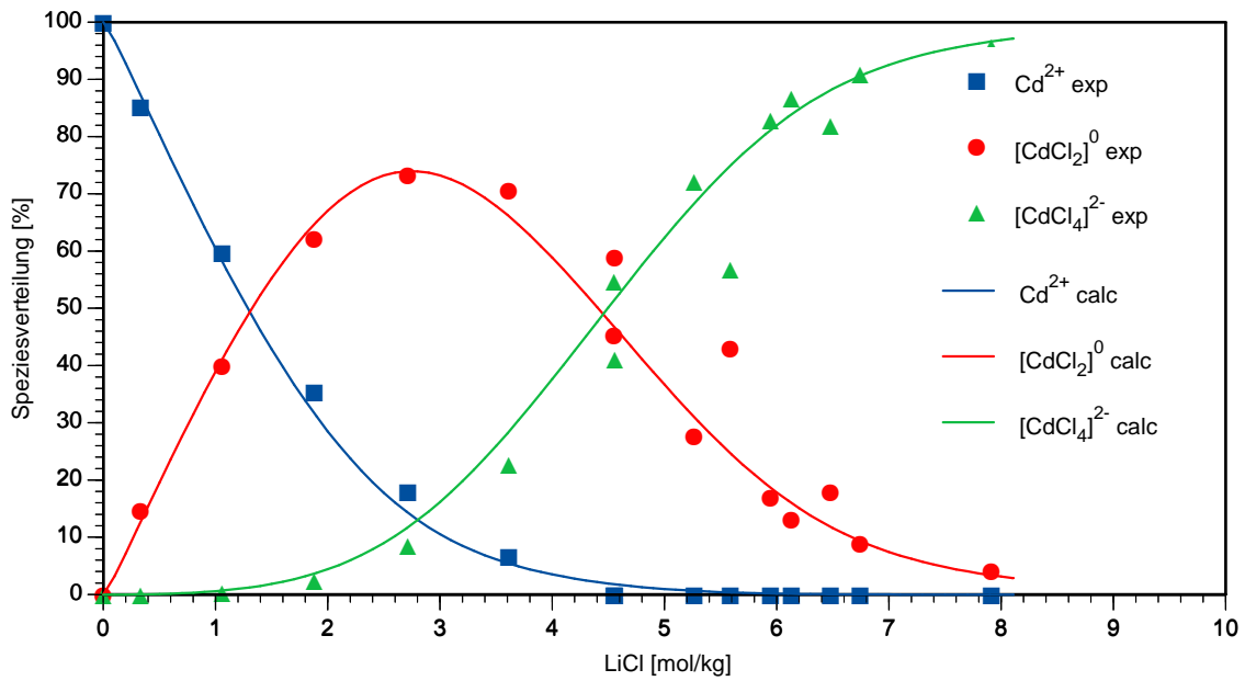
Abb. 7.2 Experimentelle (Raman) und berechnete Speziesverteilung im System \text{Cd}(\text{ClO}_4)_2 - \text{LiCl} - \text{H}_2\text{O} bei 25 °C
