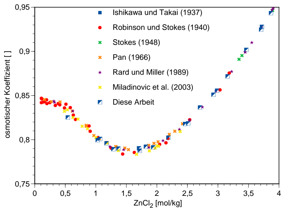
Abb. 2.2 Literaturdaten und eigene isopiestic Messungen im System \text{ZnCl}_2 – \text{H}_2\text{O}
