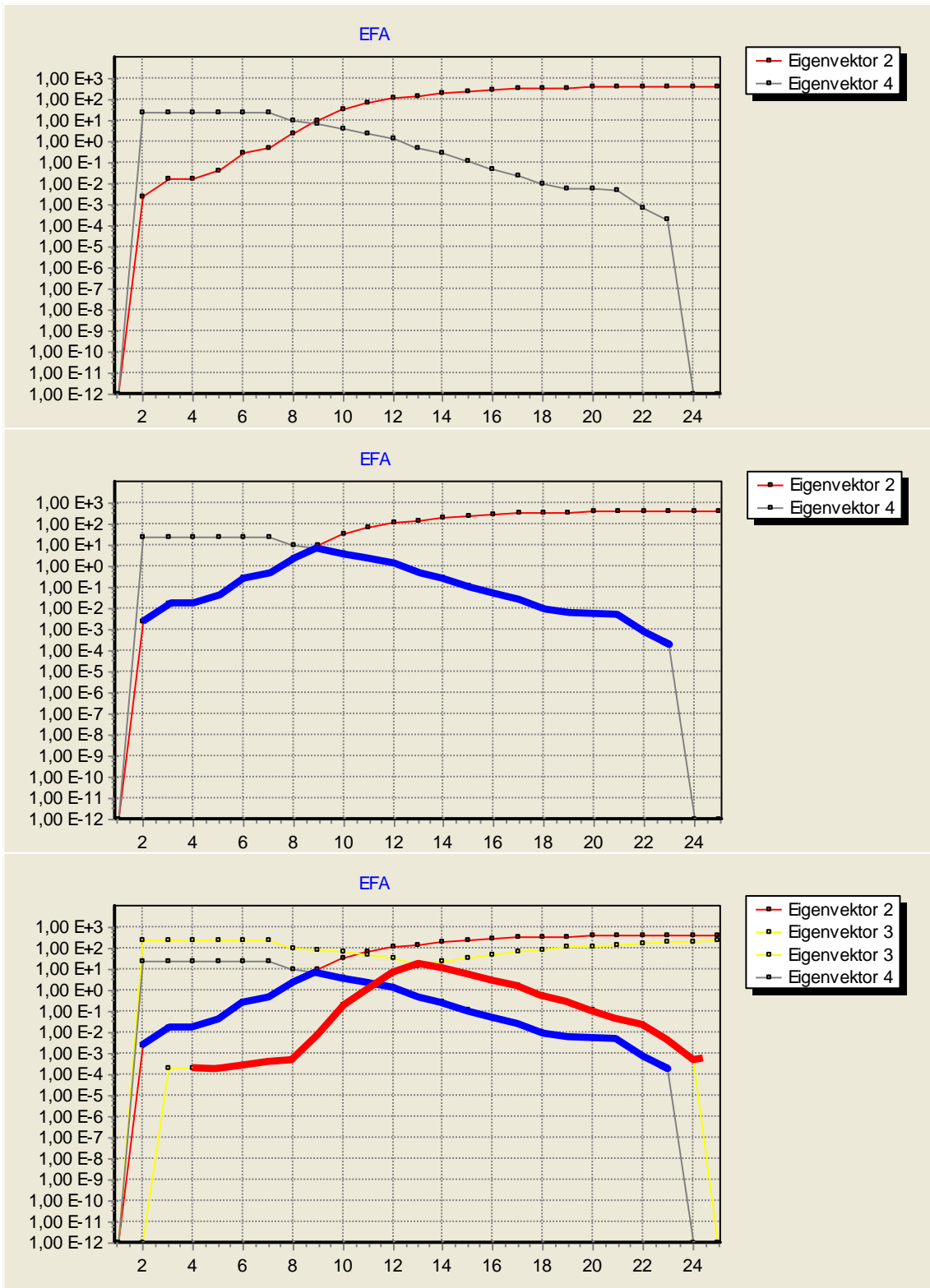
Abb. 4.2 Evolving Factor Analysis: schrittweises Hinzufügen weiterer Faktoren
