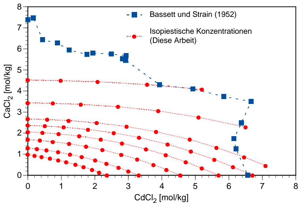
Abb. 2.19 Experimentell bestimmte Isoaktivitätslinien im System CdCl 2 – CaCl 2 – H 2 O
