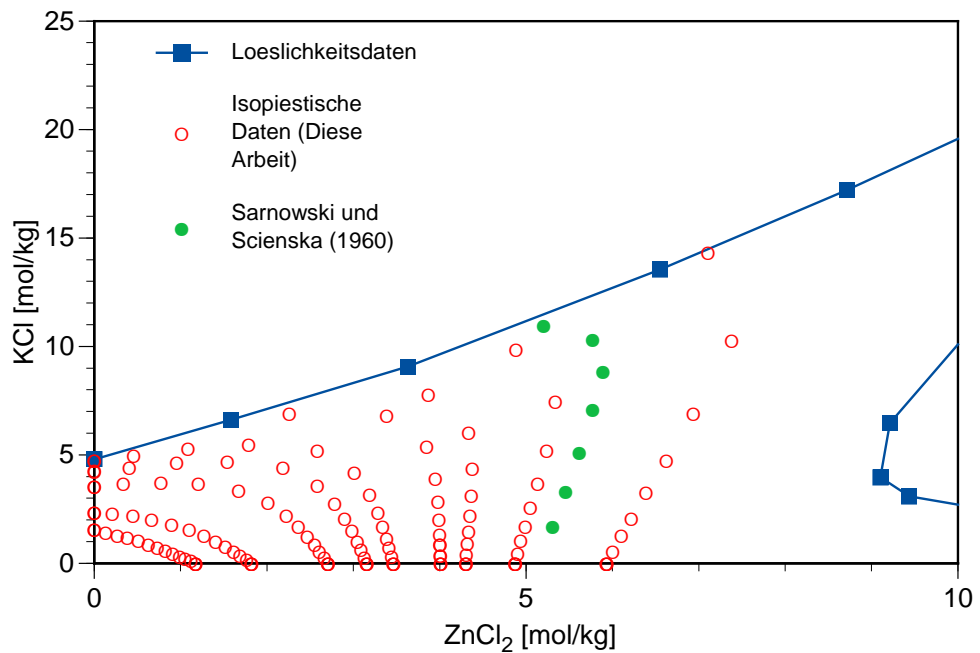
Abb. 2.6 Isopiestiche Konzentrationen im System \text{ZnCl}_2 - \text{KCl} - \text{H}_2\text{O}
