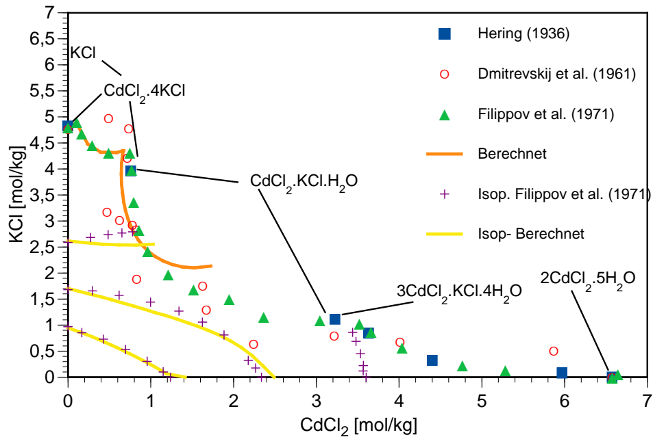
Abb. 7.13 Phasengleichgewichte im System \text{CdCl}_2\text{--KCl--H}_2\text{O} bei 25\text{ }^\circ\text{C}
