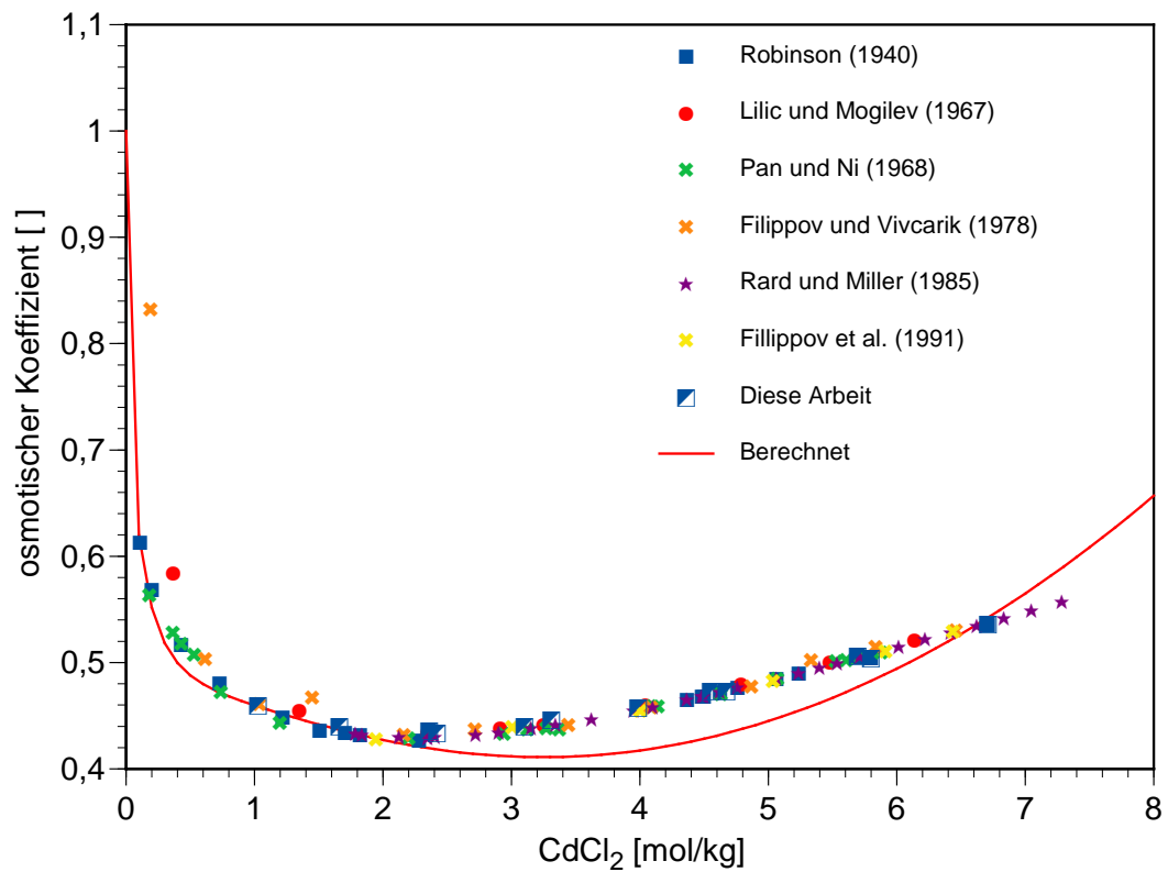
Abb. 7.6 Isopiestic bestimmte osmotische Koeffizienten im System \text{CdCl}_2 - \text{H}_2\text{O}
