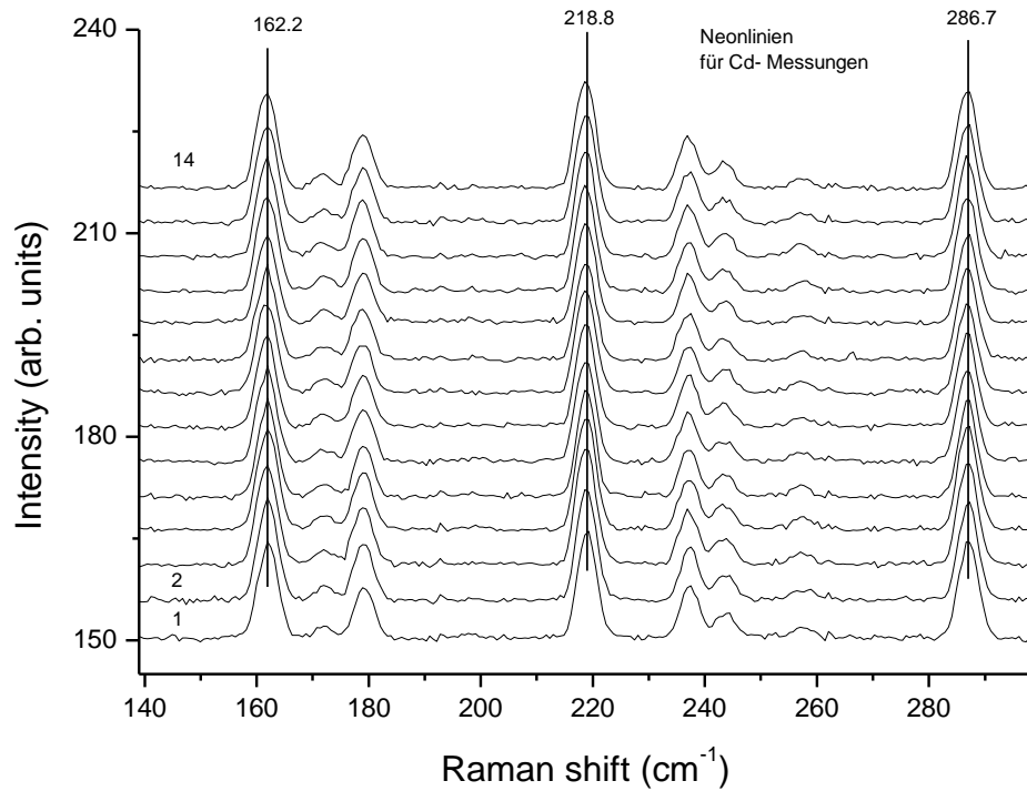
Abb. 3.4 Neonlinien der Kalibrierlampe
