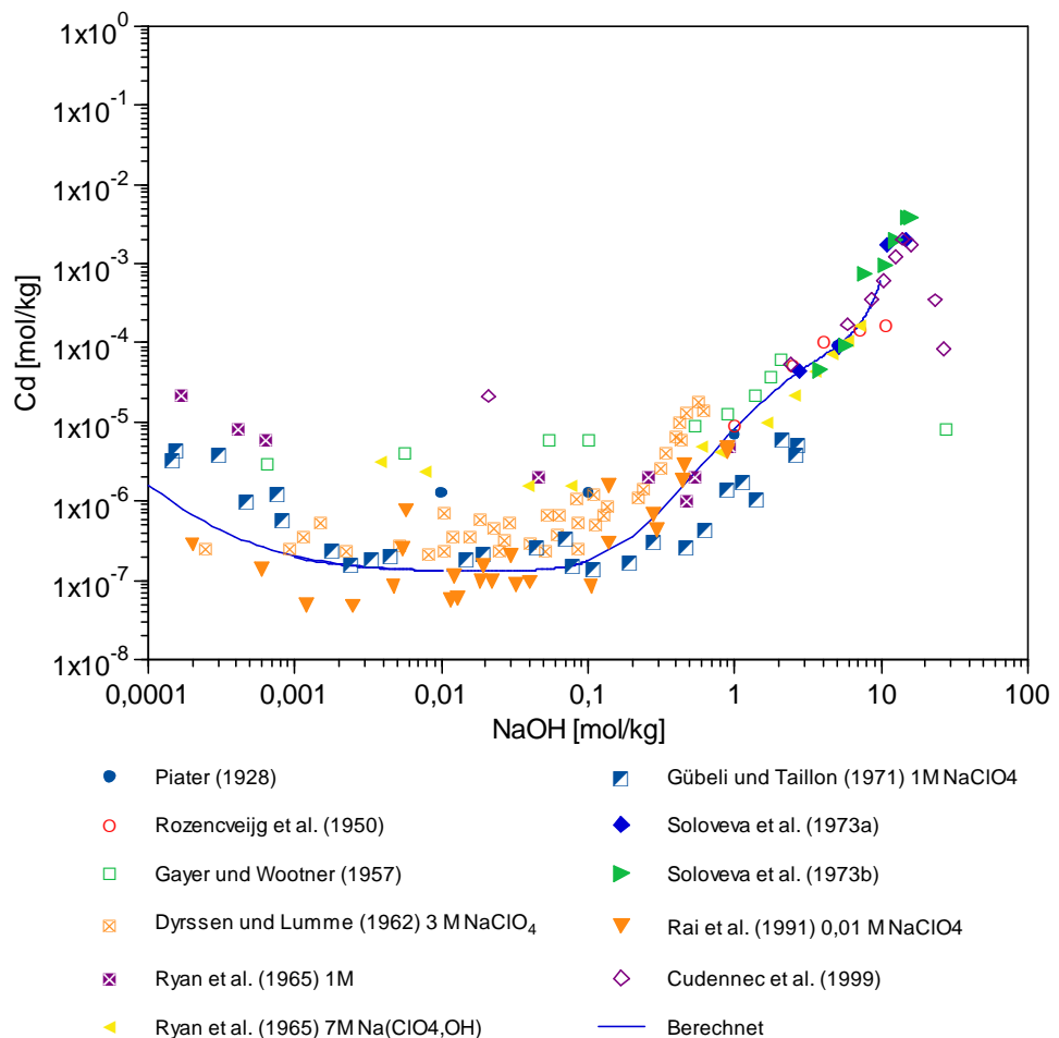
Abb. 9.3 Löslichkeit von \beta\text{-Cd}(\text{OH})_2 in NaOH-Lösungen
