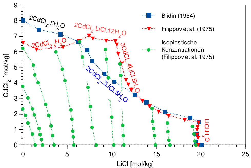
Abb. 7.16 Phasengleichgewicht im System LiCl–CdCl 2 –H 2 O bei 25 °C
