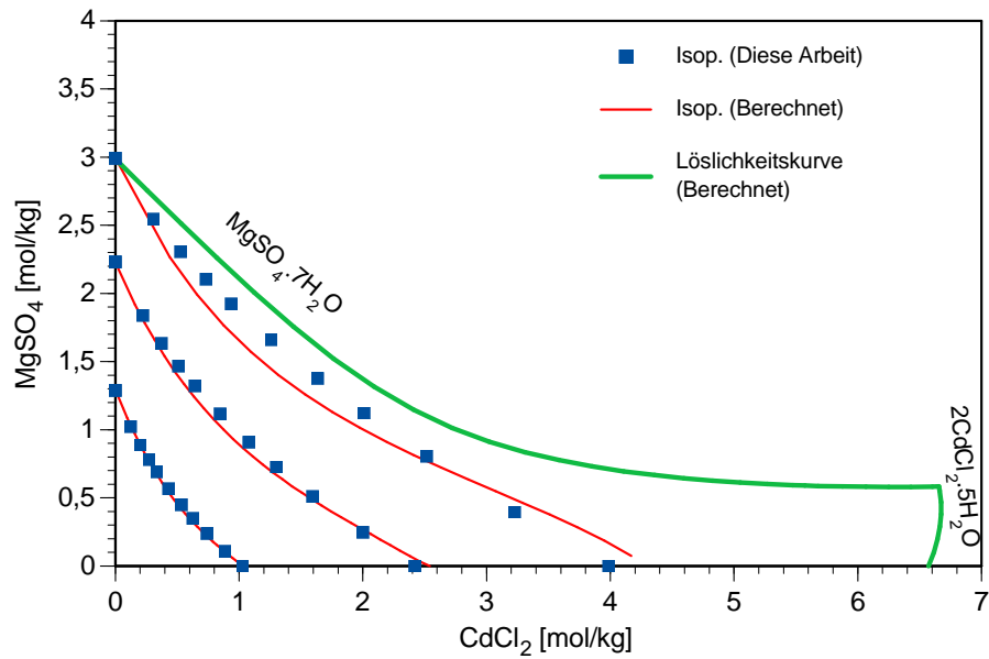
Abb. 7.23 Phasengleichgewichte im System CdCl 2 -MgSO 4 -H 2 O bei 25 °C
