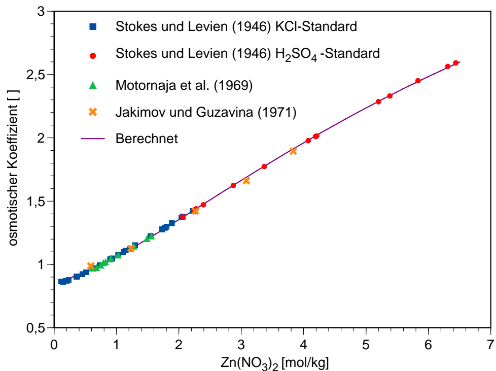
Abb. 8.7 Experimentelle und berechnete osmotische Koeffizienten von Zn(NO 3 ) 2 -Lösungen bei 25,0 °C
