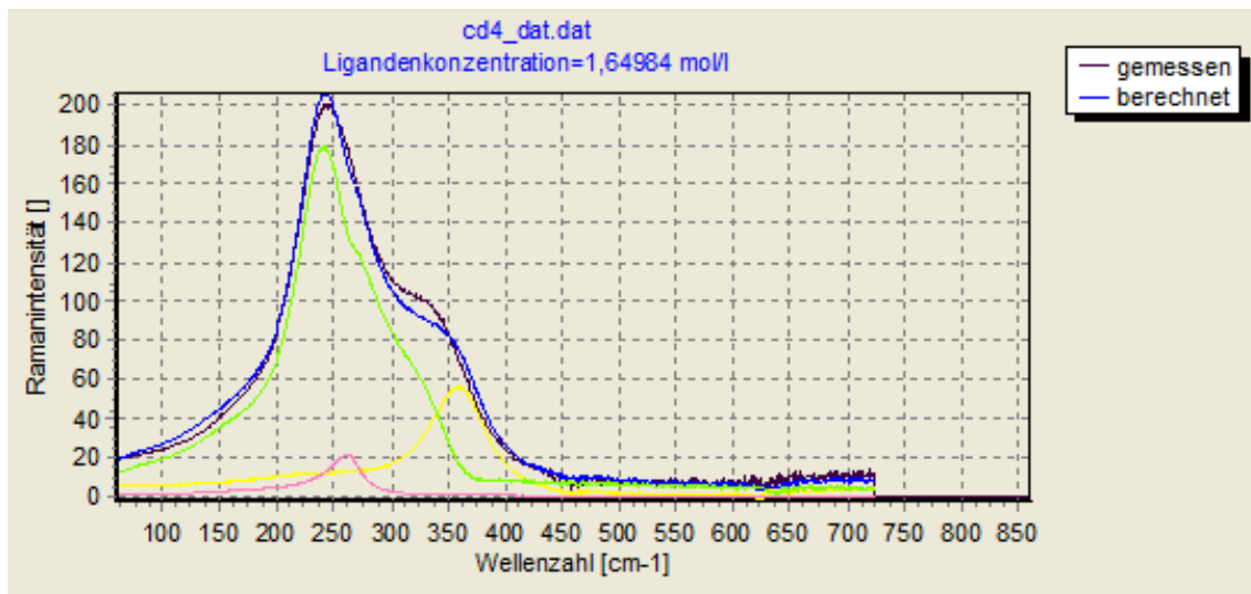
Abb. 6.4 Polarisiertes Ramanspektrum der Lösung CdLi 4 : Abweichungen zwischen berechnetem und gemessenem Spektrum bei 330 cm -1 (Hinweis auf Cadmiummonochlorokomplex)
