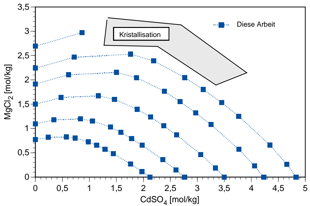
Abb. 2.25 Isopiestic concentrations im System \text{CdSO}_4 - \text{MgCl}_2 - \text{H}_2\text{O} bei 25 °C
