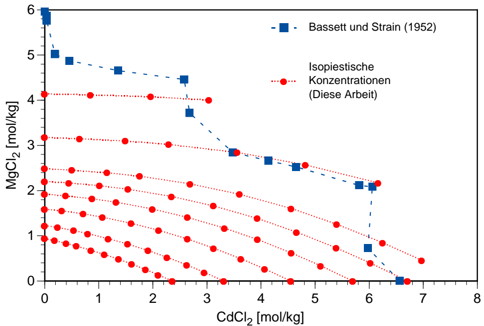
Abb. 2.18 Experimentell bestimmte Isoaktivitätslinien im System CdCl 2 – MgCl 2 – H 2 O
