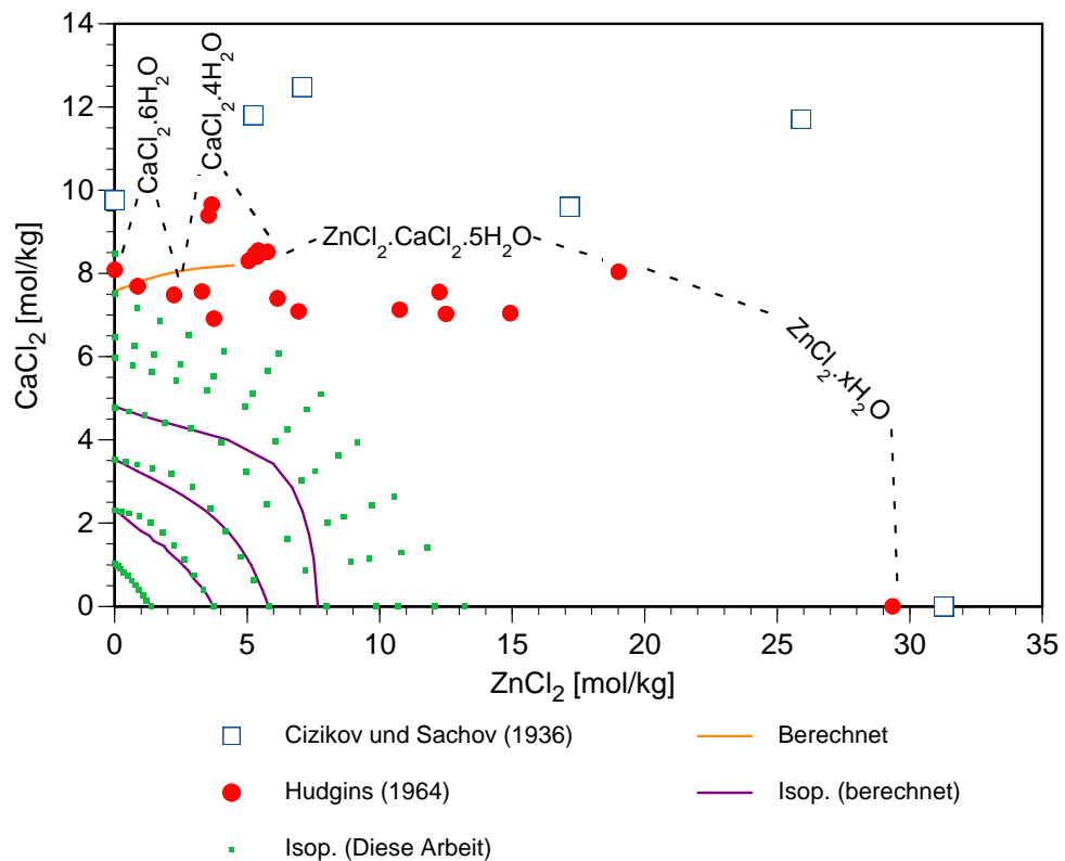
Abb. 8.13 Experimentelle und berechnete Phasengleichgewichte im System \text{ZnCl}_2 - \text{CaCl}_2 - \text{H}_2\text{O} bei 25^\circ\text{C}
