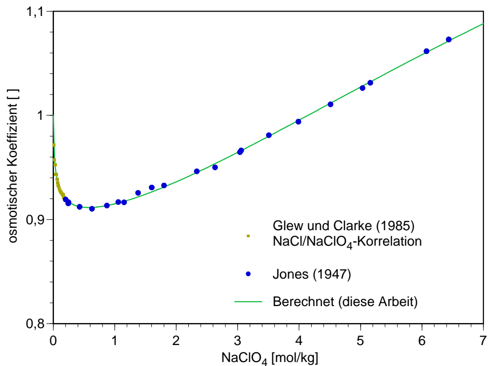
Abb. 7.26 Experimentelle und berechnete osmotische Koeffizienten im System \text{NaClO}_4 - \text{H}_2\text{O} bei 25 °C
