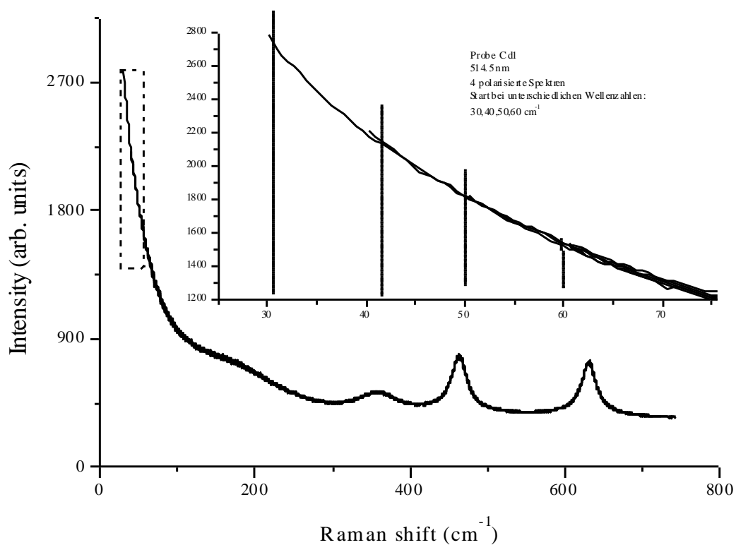
Abb. 3.6 Streulichtfreiheit des Spektrometers T64000 im „subtractive mode“
