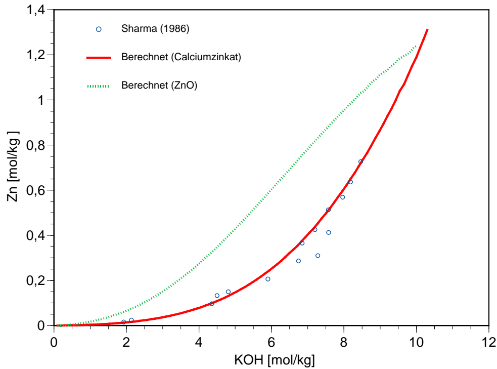
Abb. 10.5 Löslichkeit von Calciumzinkat und Zinkit in KOH-Lösungen in Gegenwart von Portlandit – \text{Ca}(\text{OH})_2
