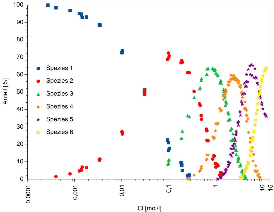
Abb. 5.3 Konzentrationsverteilung eines 6-Spezies-Modells
