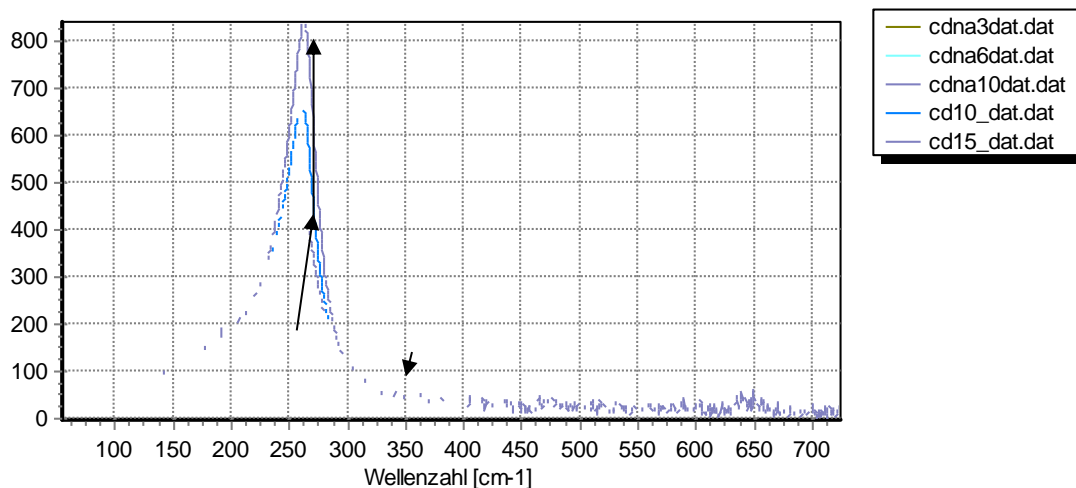
Abb. 6.2 Ramanspektren von \text{Cd}(\text{ClO}_4)_2 -Lösungen (etwa 1 mol/l) mit Zusatz von 1,2 – 6,3 mol/l NaCl oder LiCl
