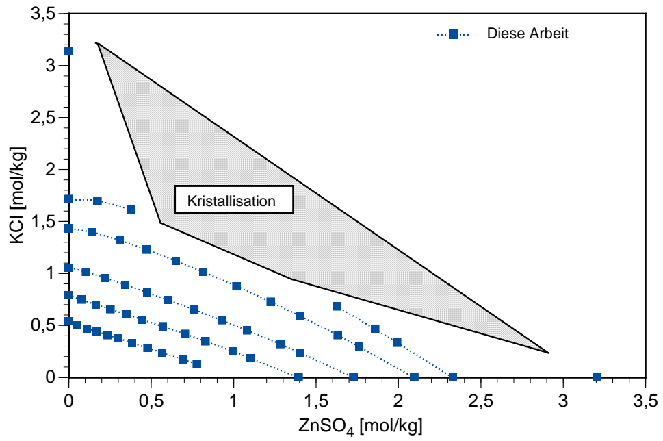
Abb. 2.11 Isoaktivitätslinien im quasi-ternären System ZnSO 4 – KCl – H 2 O
