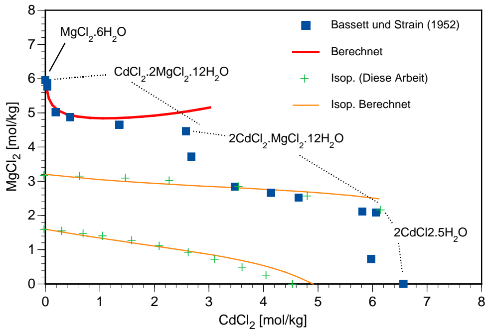
Abb. 7.14 Phasengleichgewichte im System \text{CdCl}_2\text{-MgCl}_2\text{-H}_2\text{O} bei 25 °C
