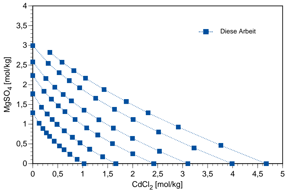
Abb. 2.24 Isopiestic concentrations im System \text{CdCl}_2 - \text{MgSO}_4 - \text{H}_2\text{O}
