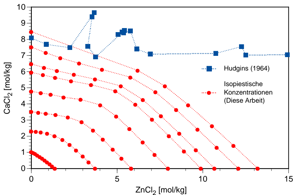
Abb. 2.8 Isopiestic Concentrations im System \text{ZnCl}_2 - \text{CaCl}_2 - \text{H}_2\text{O}
