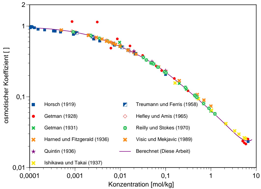
Abb. 7.5 Potentiometrisch bestimmte Aktivitätskoeffizienten im System \text{CdCl}_2 - \text{H}_2\text{O}
