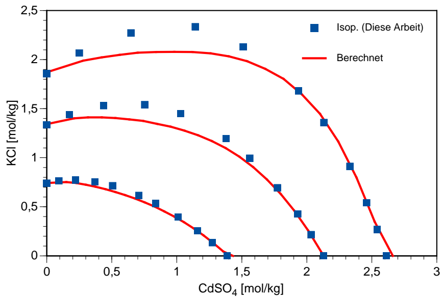
Abb. 7.22 Phasengleichgewichte im System CdSO 4 -KCl-H 2 O bei 25 °C
