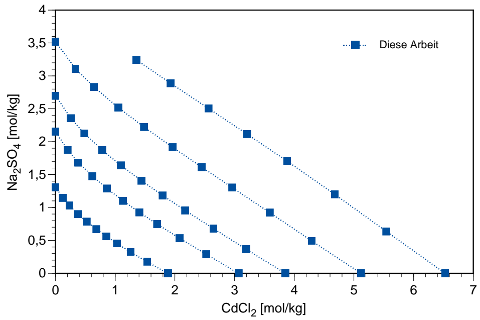
Abb. 2.21 Isopiestic Konzentrationen im System \text{CdCl}_2 - \text{Na}_2\text{SO}_4 - \text{H}_2\text{O}
