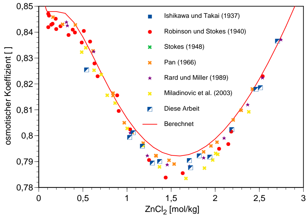
Abb. 8.1 Experimentelle und berechnete osmotische Koeffizienten im System ZnCl 2 –H 2 O bis 3 mol/kg
