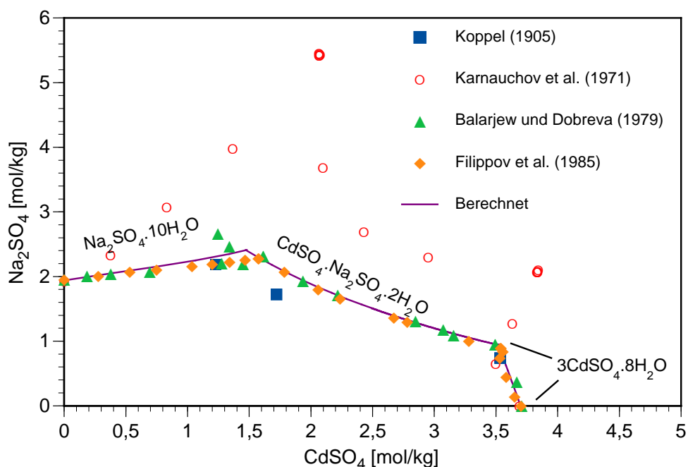
Abb. 7.17 Phasengleichgewichte im System \text{CdSO}_4\text{--Na}_2\text{SO}_4\text{--H}_2\text{O} bei 25 °C
