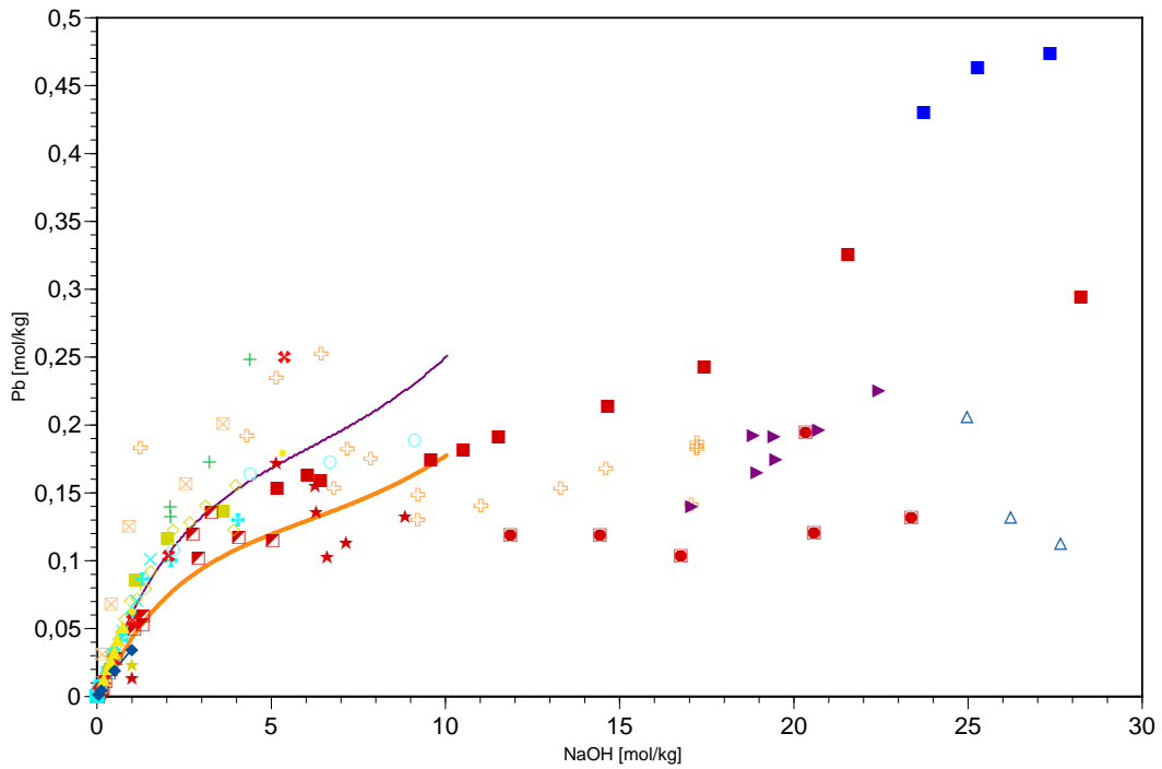
Symbole: Lithargit (rot), Massicot (gelboliv), Bleioxidhydrat (hellblau, schwarzes Bleioxid (schwarz), Natriumplumbit (dunkelblau) Linien: berechnete Werte für Lithargit (rot) und Bleioxidhydrat (blau)
