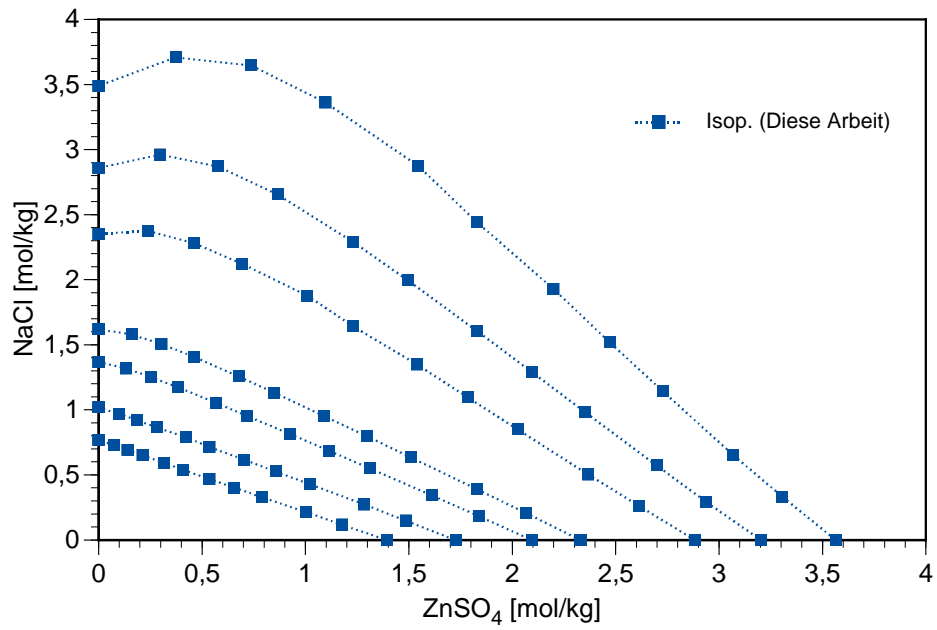
Abb. 2.9 Isoaktivitätslinien im quasi-ternären System ZnSO 4 – NaCl – H 2 O
