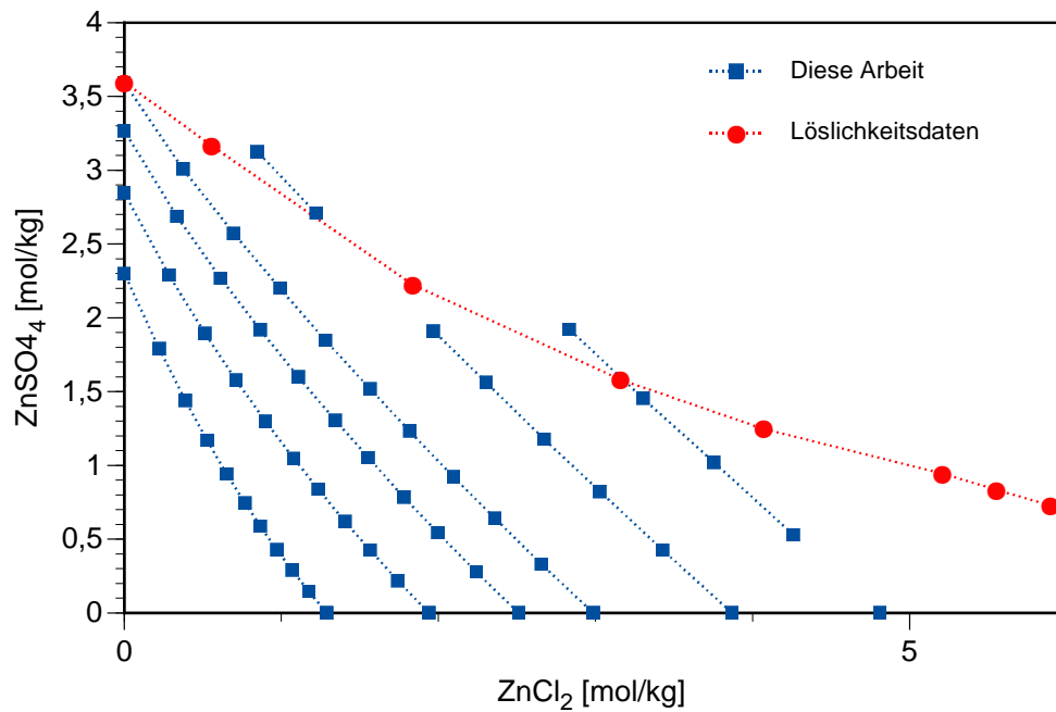
Abb. 2.4 Gemessene Isoaktivitätskurven im System \text{ZnCl}_2 - \text{ZnSO}_4 - \text{H}_2\text{O}
