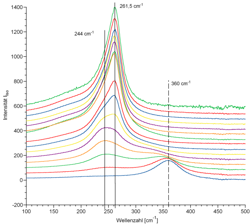
Abb. 3.16 Raman-Spektren von Cd(ClO 4 ) 2 -Lösungen mit zunehmender LiCl-Konzentration
