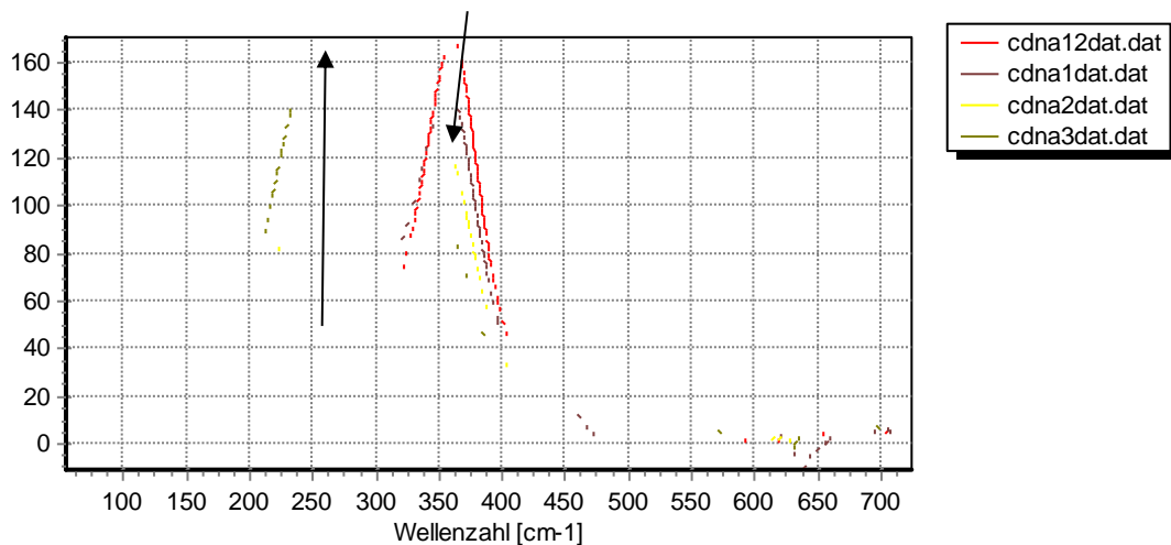
Abb. 6.1 Ramanspektren von \text{Cd}(\text{ClO}_4)_2 -Lösungen (etwa 1\text{ mol/l} ) mit Zusatz von 0 – 1,2\text{ mol/l} NaCl oder LiCl
