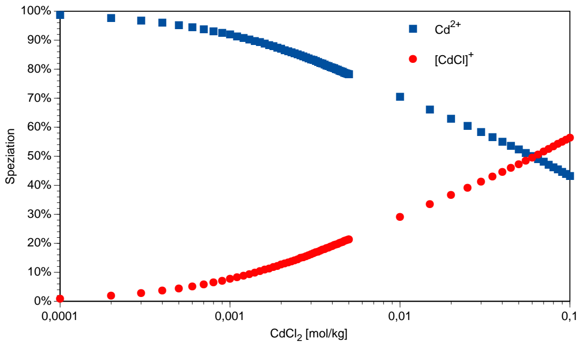
Abb. 7.4 Abgeleitete Speziation für kleine CdCl 2 -Konzentrationen
