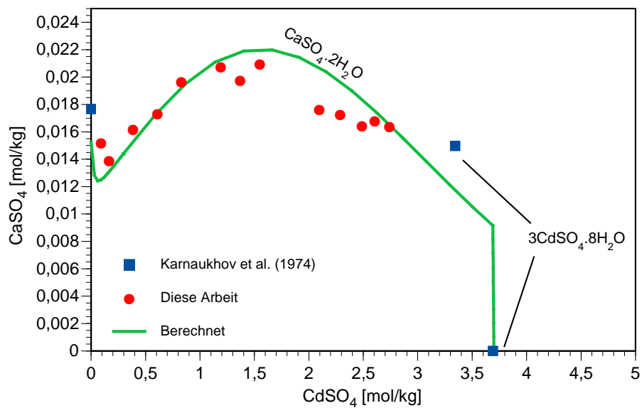
Abb. 7.20 Phasengleichgewichte im System \text{CdSO}_4\text{-CaSO}_4\text{-H}_2\text{O} bei 25\text{ }^\circ\text{C}
