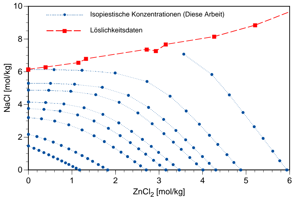
Abb. 2.5 Isopiestic Konzentrationen im System \text{ZnCl}_2 - \text{NaCl} - \text{H}_2\text{O}
