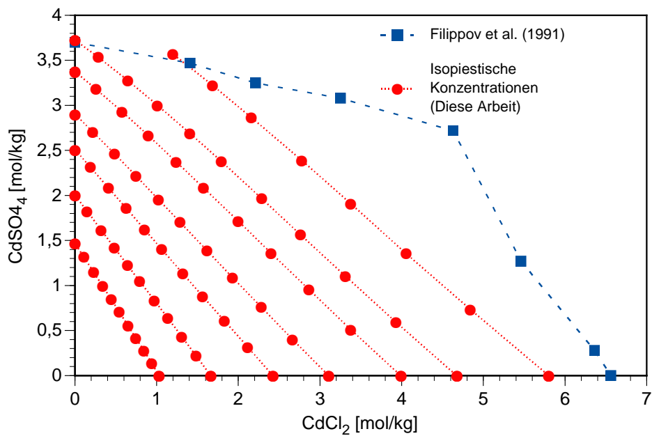
Abb. 2.17 Isopiestic Konzentrationen im System \text{CdCl}_2 - \text{CdSO}_4 - \text{H}_2\text{O}
