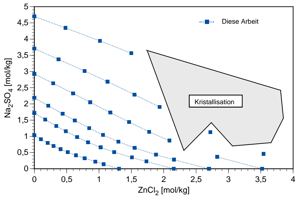
Abb. 2.10 Isoaktivitätslinien im quasi-ternären System ZnCl 2 – Na 2 SO 4 – H 2 O
