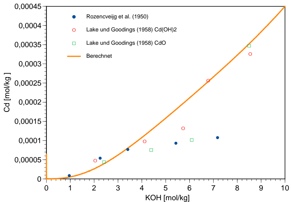
Abb. 9.5 Löslichkeit von Cd(OH) 2 in KOH-Lösungen
