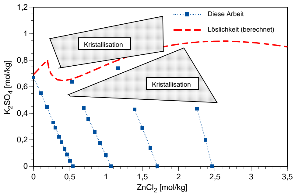
Abb. 2.12 Isoaktivitätslinien im quasi-ternären System ZnCl 2 -K 2 SO 4 -H 2 O
