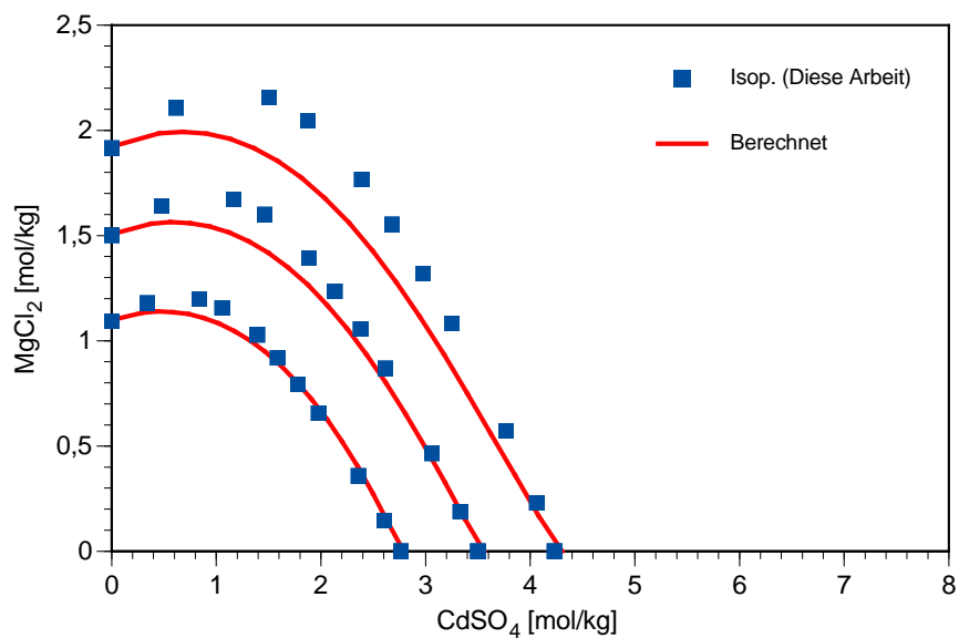
Abb. 7.24 Phasengleichgewichte im System CdSO 4 -MgCl 2 -H 2 O bei 25 °C
