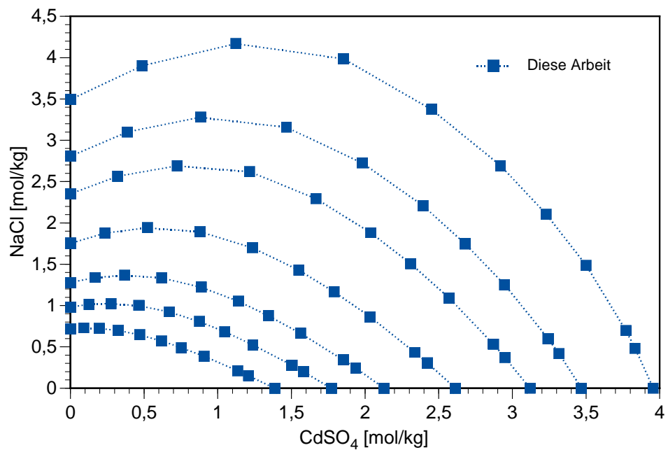
Abb. 2.20 Isopiestic Konzentrationen im System CdSO 4 – NaCl – H 2 O
