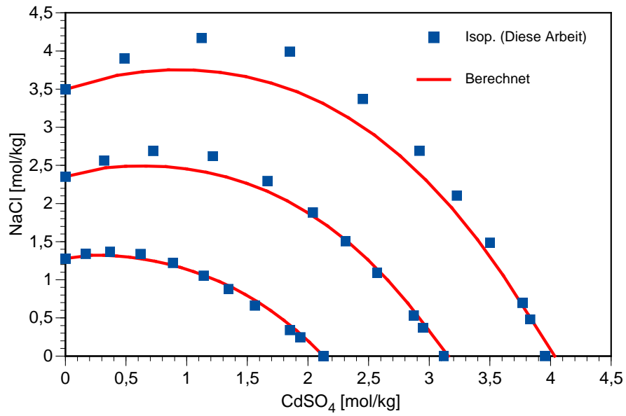
Abb. 7.21 Phasengleichgewichte im System CdSO 4 -NaCl-H 2 O bei 25 °C
