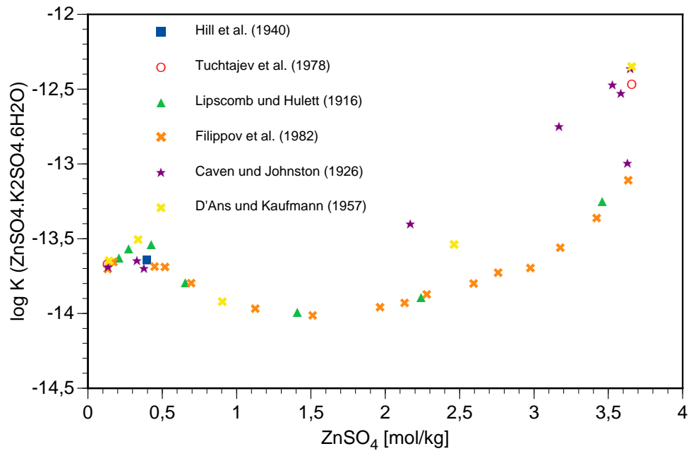
Abb. 8.15 Berechnete Löslichkeitskonstante für \text{ZnSO}_4 \cdot \text{K}_2\text{SO}_4 \cdot 6\text{H}_2\text{O}
