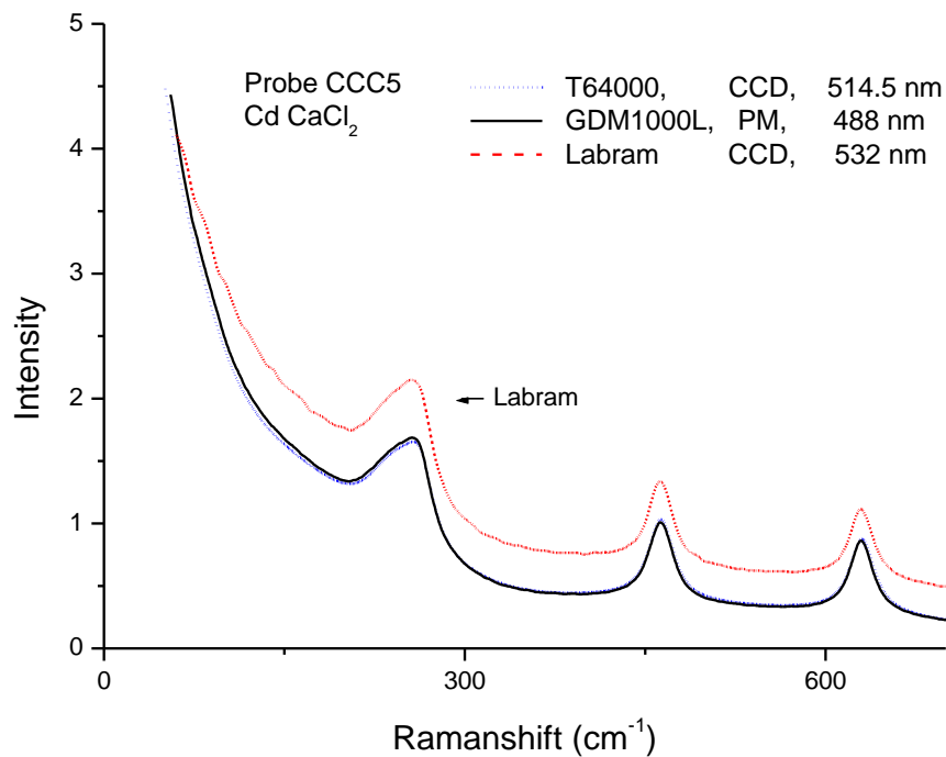
Abb. 3.2 Vergleichsmessungen für eine Probe mit unterschiedlichen Messanordnungen
