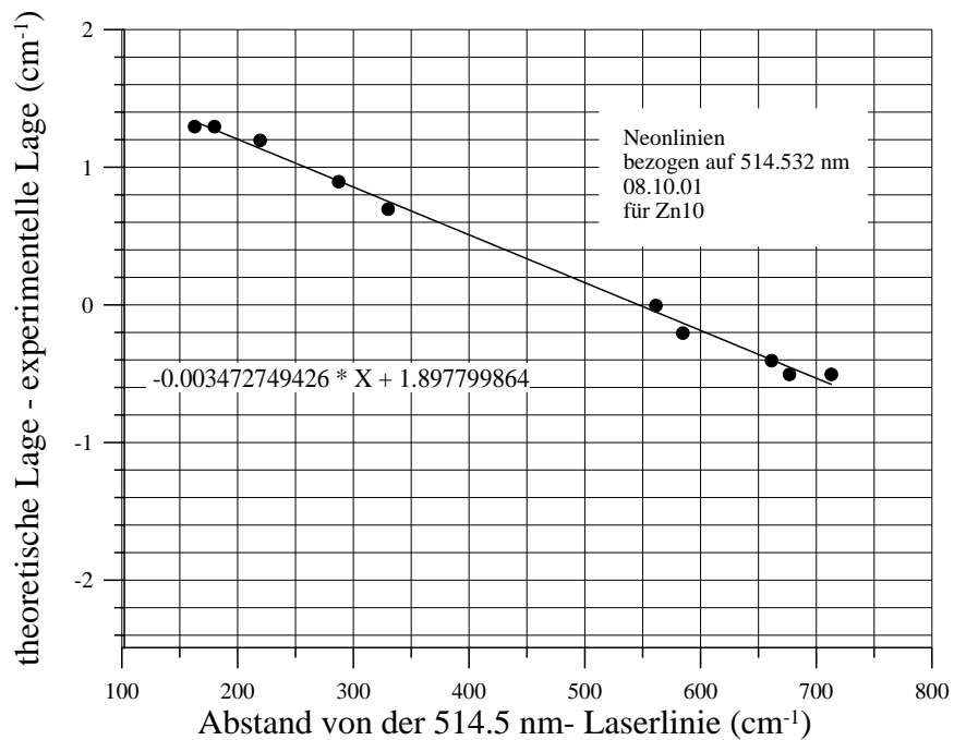
Abb. 3.5 Wellenzahlkorrektur
