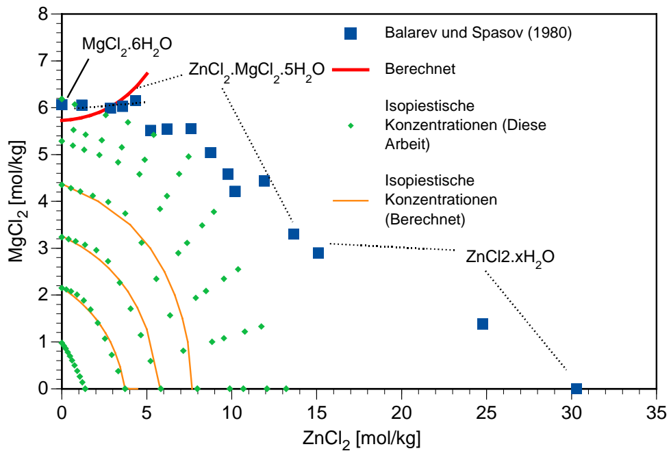
Abb. 8.12 Experimentelle und berechnete Phasengleichgewichte im System ZnCl 2 –MgCl 2 –H 2 O bei 25 °C
