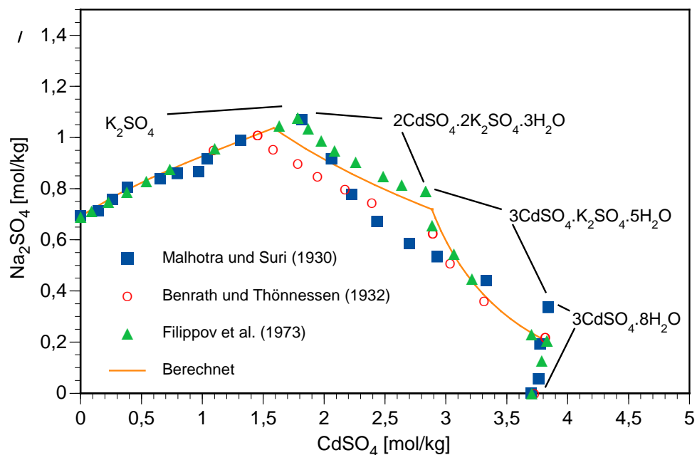
Abb. 7.18 Phasengleichgewichte im System \text{CdSO}_4 - \text{K}_2\text{SO}_4 - \text{H}_2\text{O} bei 25\text{ °C}
