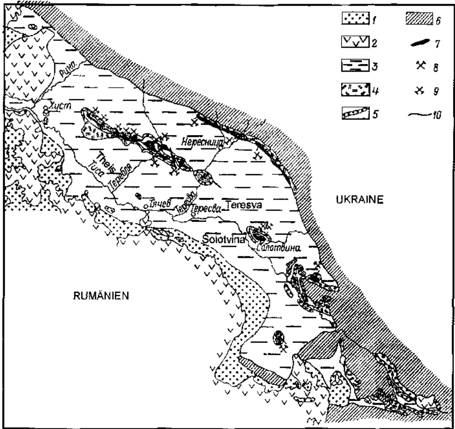
Abb. 6.12 Lage der Ukrainischen Salzbergwerke im Transkarpaten-Raum
