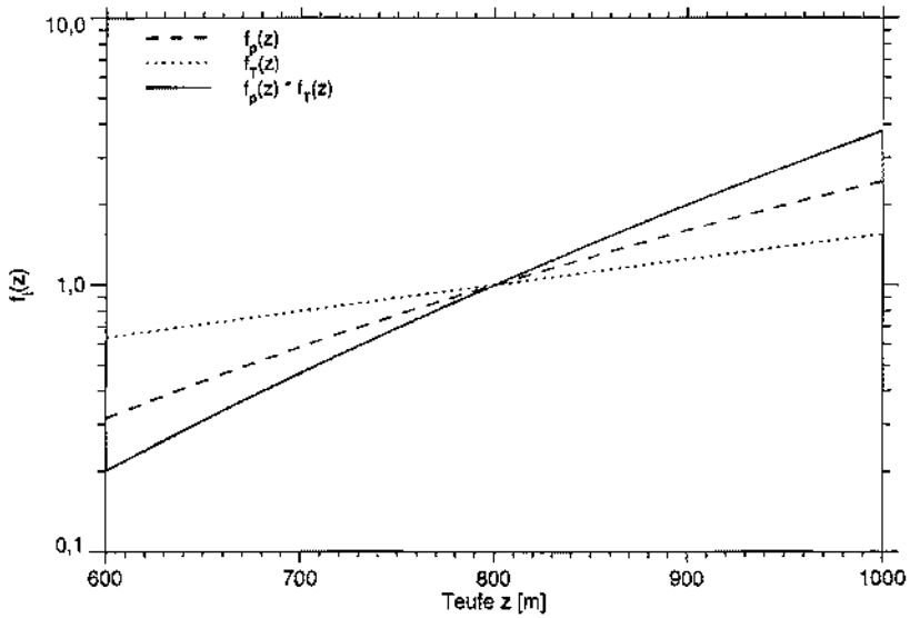
Abb. 5.2 Abhängigkeit der thermomechanischen Funktionen von der Teufenlage, bezogen auf eine Referenztiefe von z_r = 800 m
