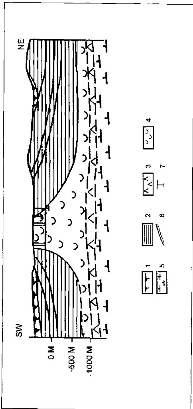
Schematisches Profil durch den Salinar-Bereich von Soltovina, Westukraine
