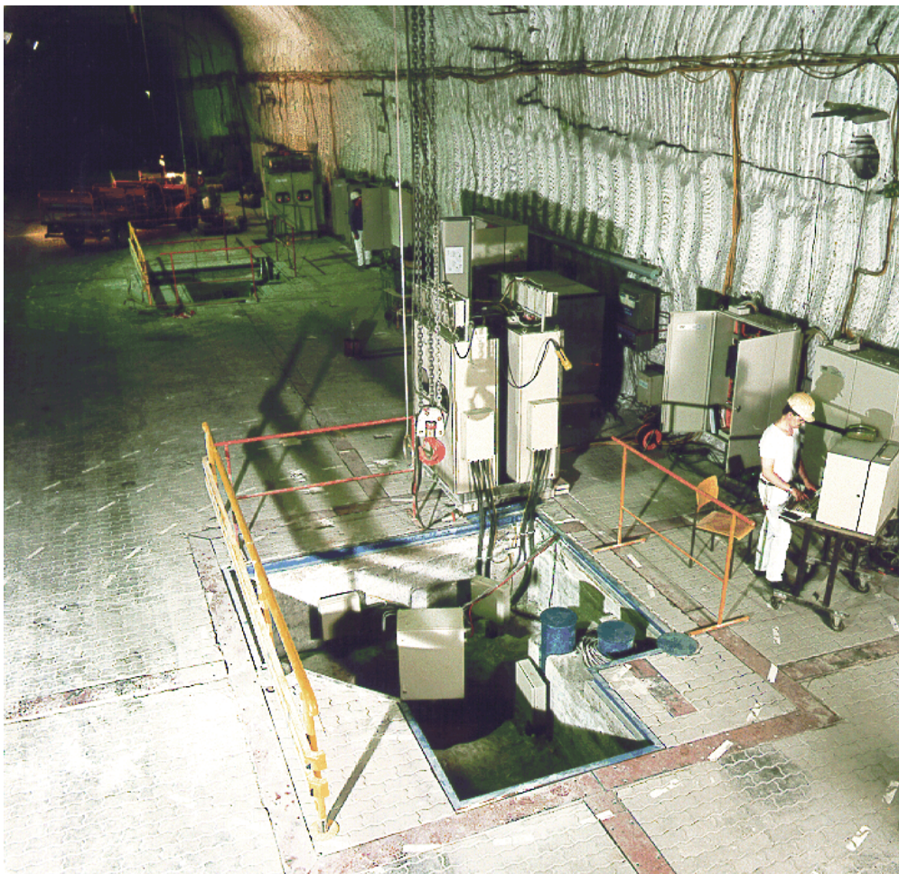
Abb. 48 DEBORA-Versuche im HAW-Versuchsfeld auf der 800-m-Sohle der Schachtanlage Asse
