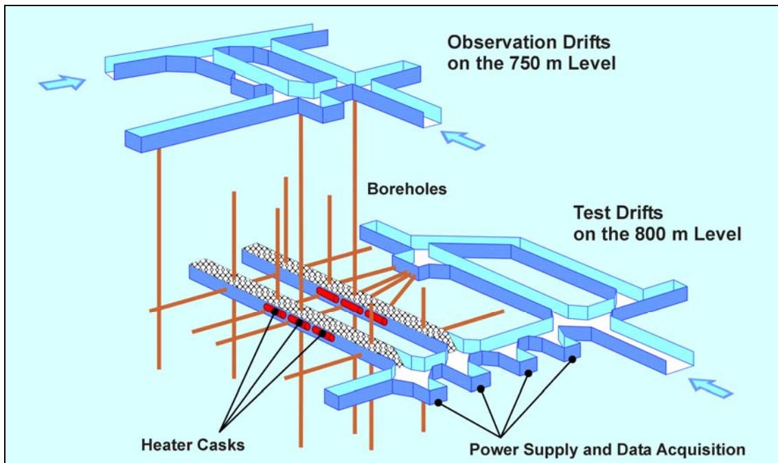
Abb. 41 TSS-Versuchsfeld in der Schachtanlage Asse mit den beiden versetzten Versuchsstrecken auf der 800-m-Sohle sowie Zugangs- und Beobachtungsstrecken auf der 750-m- und 800-m-Sohle
