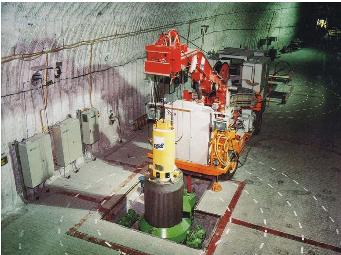
Abb. 40 HAW-Versuch zur Demonstrationseinlagerung hochradioaktiver Versuchsquellen: Einlagerungsmaschine am Einlagerungsbohrloch /GSF 95/
