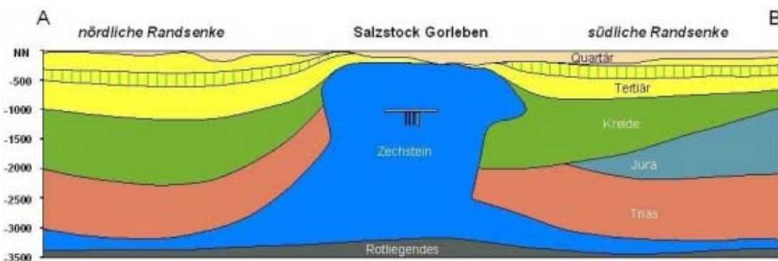
Abb. 3 Vereinfachter geologischer Schnitt durch den Salzstock Gorleben („Zechstein“). Die Endlagerung radioaktiver Abfälle ist im zentralen Teil des Salzstockes in etwa 840 m Teufe vorgesehen /BGR 08/
