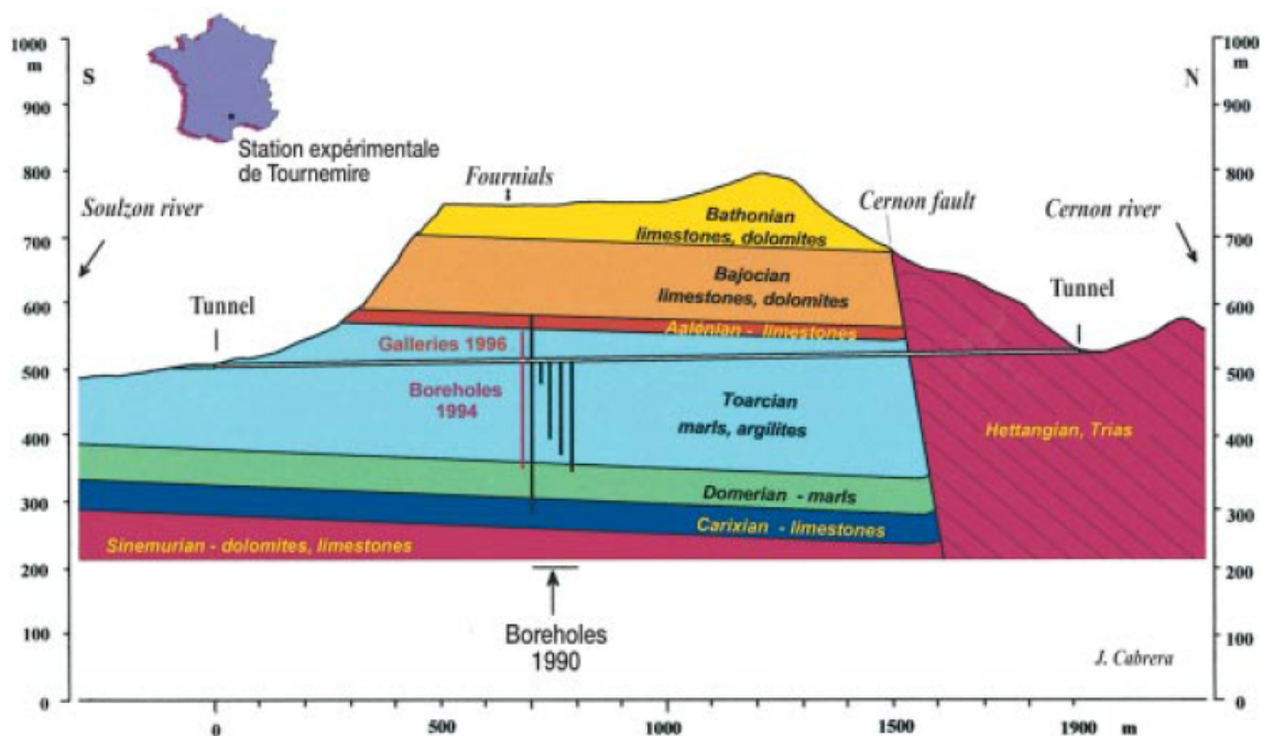
Abb. 19 Geologischer Schnitt durch den als UTL genutzten stillgelegten Eisenbahntunnel bei Tournemire /CAB 02/
